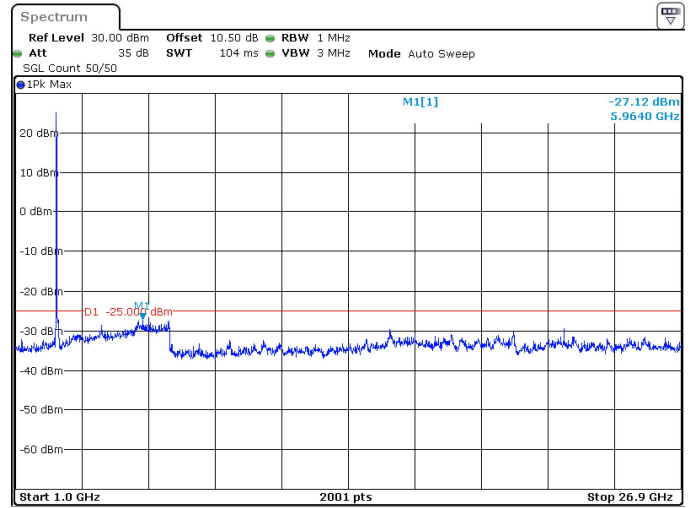
100MHz_30kHz_2640MHz_DFT-s-OFDM QPSK_RB1@0 -27.12 dBm
