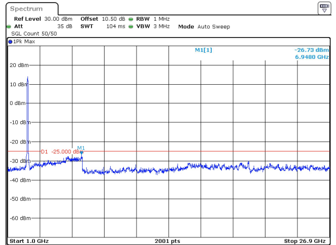
100MHz_30kHz_2592.99MHz_DFT-s-OFDM QPSK_RB270@0 -26.73 dBm
