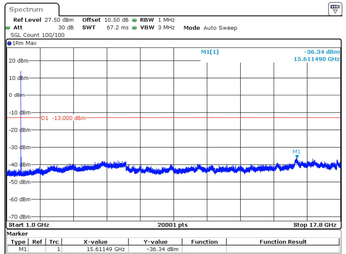
5MHz_15kHz_1712.5MHz_DFT-s-OFDM QPSK_RB1@0 -36.34 dBm
