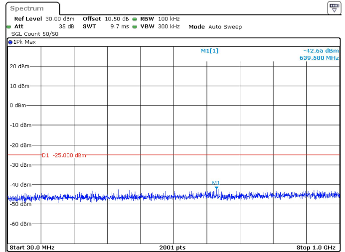
100MHz_30kHz_2640MHz_DFT-s-OFDM QPSK_RB1@272 -42.65 dBm
