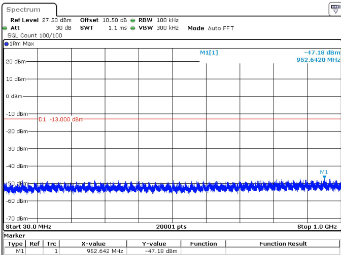
5MHz_15kHz_1712.5MHz_DFT-s-OFDM QPSK_RB1@0 -47.18 dBm
