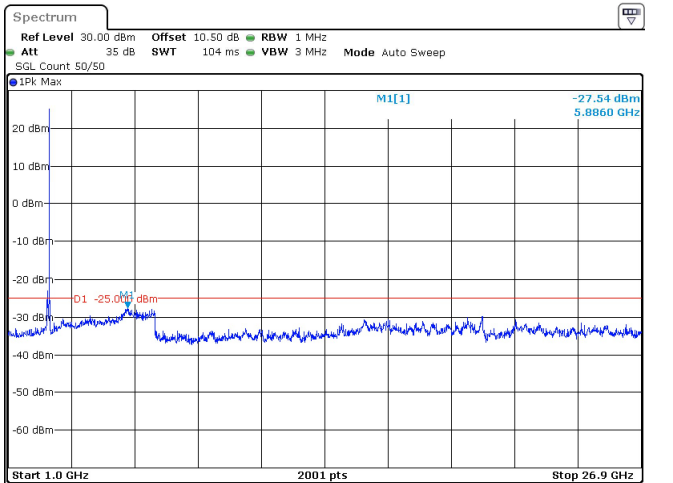
100MHz_30kHz_2640MHz_DFT-s-OFDM QPSK_RB1@272 -27.54 dBm
