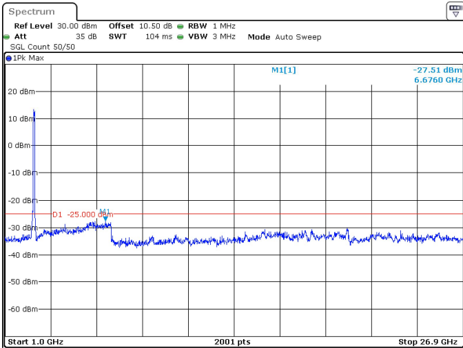
100MHz_30kHz_2640MHz_DFT-s-OFDM QPSK_RB270@0 -27.51 dBm
