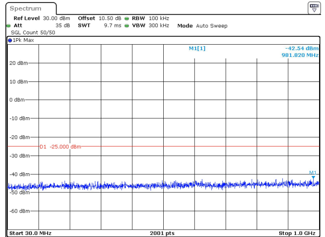
100MHz_30kHz_2640MHz_DFT-s-OFDM QPSK_RB270@0 -42.54 dBm
