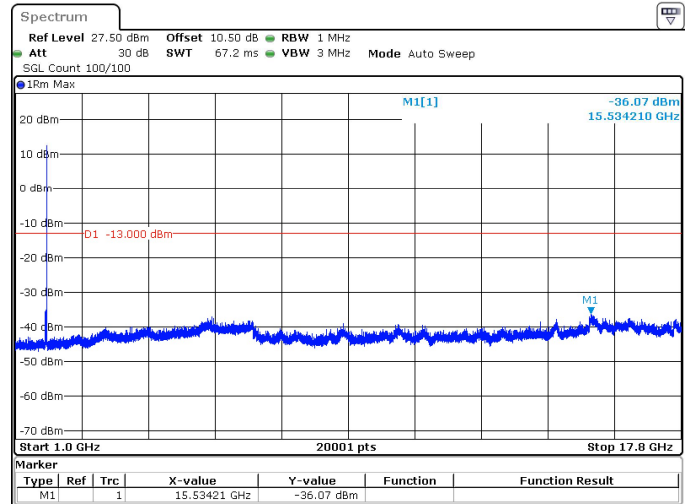
20MHz_15kHz_1770MHz_DFT-s-OFDM QPSK_RB1@105 -36.07 dBm
