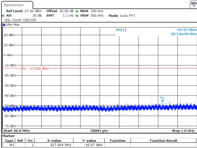
20MHz_15kHz_1770MHz_DFT-s-OFDM QPSK_RB100@0 -45.97 dBm
