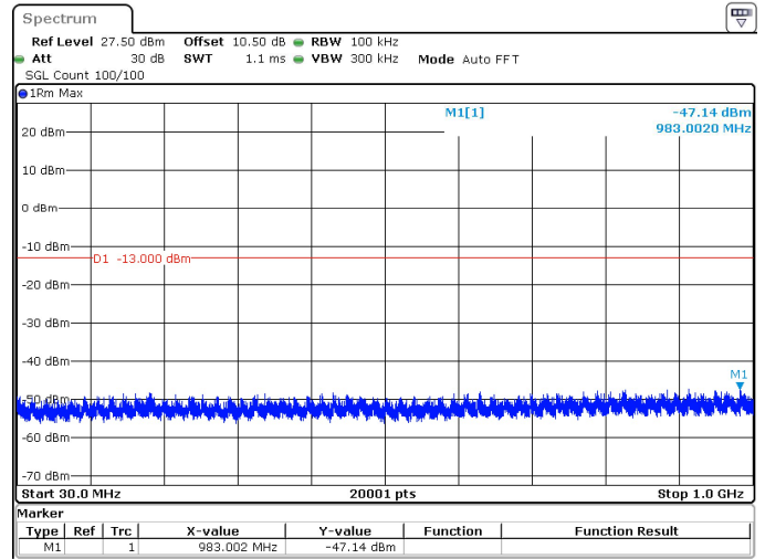
20MHz_15kHz_1745MHz_DFT-s-OFDM QPSK_RB1@0 -47.14 dBm
