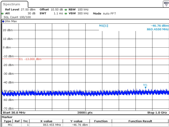
20MHz_15kHz_1770MHz_DFT-s-OFDM QPSK_RB1@0 -46.76 dBm
