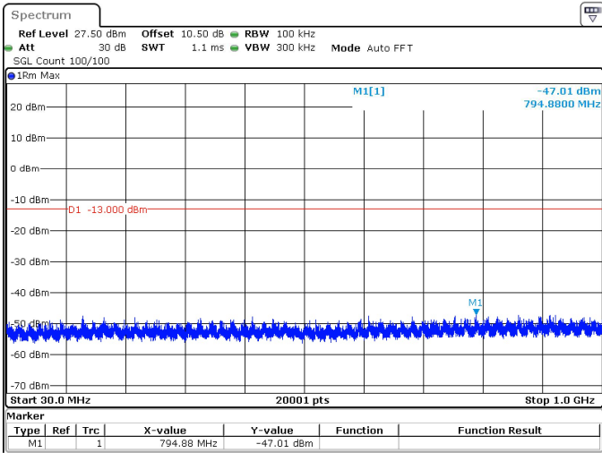
20MHz_15kHz_1720MHz_DFT-s-OFDM QPSK_RB100@0 -47.01 dBm
