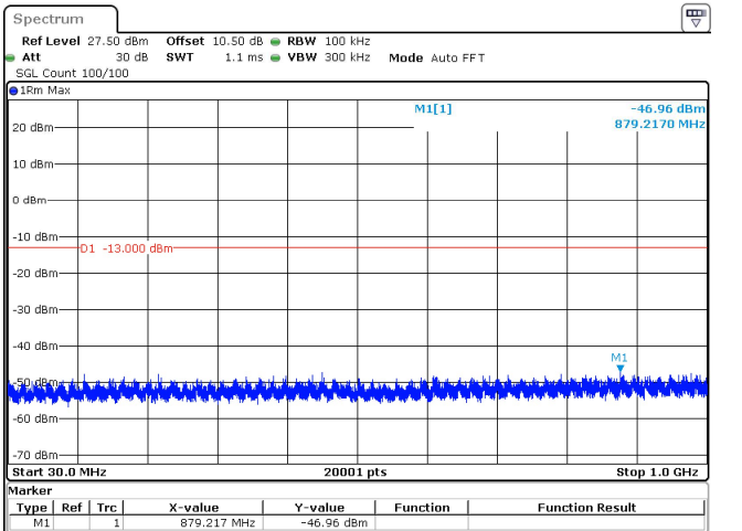
20MHz_15kHz_1770MHz_DFT-s-OFDM QPSK_RB1@105 -46.96 dBm
