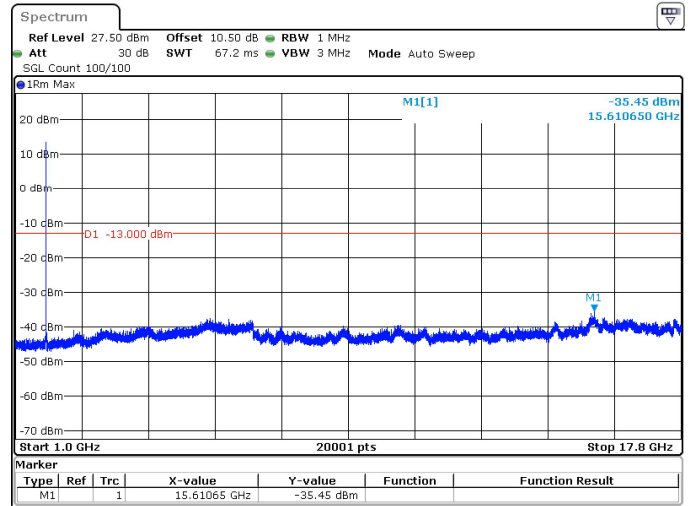
20MHz_15kHz_1770MHz_DFT-s-OFDM QPSK_RB1@0 -35.45 dBm
