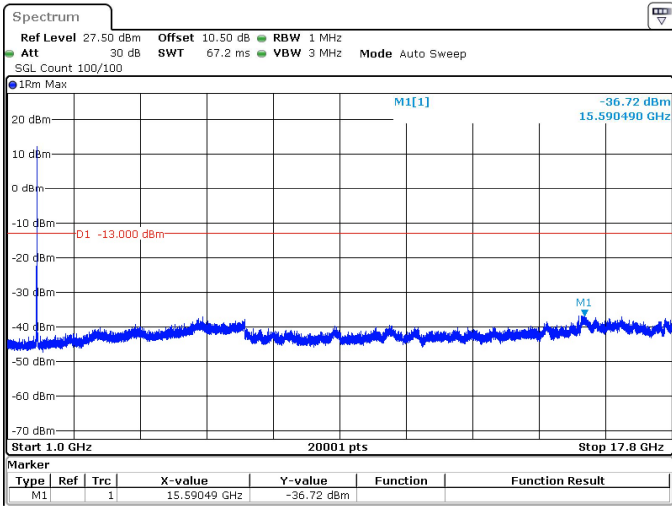
20MHz_15kHz_1745MHz_DFT-s-OFDM QPSK_RB1@0 -36.72 dBm
