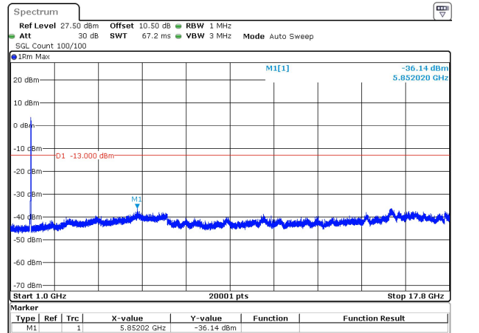
20MHz_15kHz_1770MHz_DFT-s-OFDM QPSK_RB100@0 -36.14 dBm
