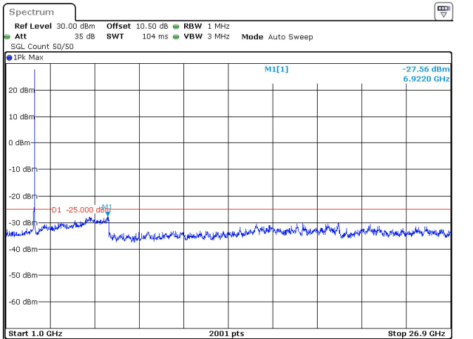
90MHz_30kHz_2644.98MHz_DFT-s-OFDM QPSK_RB1@244 -27.56 dBm
