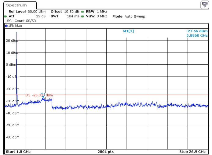
100MHz_30kHz_2546.01MHz_DFT-s-OFDM QPSK_RB1@0 -27.55 dBm
