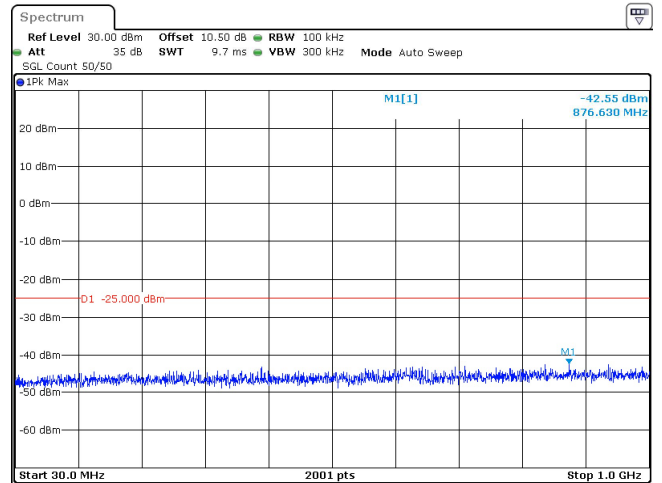
100MHz_30kHz_2546.01MHz_DFT-s-OFDM QPSK_RB270@0 -42.55 dBm
