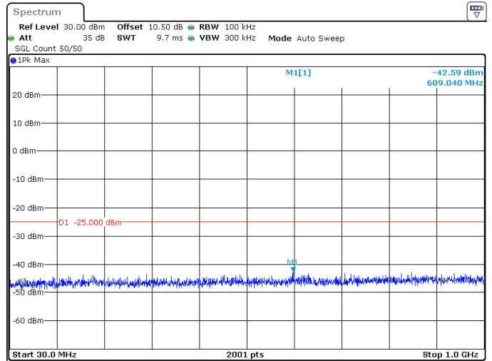
90MHz_30kHz_2644.98MHz_DFT-s-OFDM QPSK_RB1@244 -42.59 dBm
