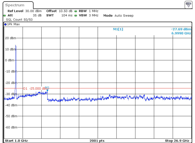
90MHz_30kHz_2644.98MHz_DFT-s-OFDM QPSK_RB243@0 -27.69 dBm
