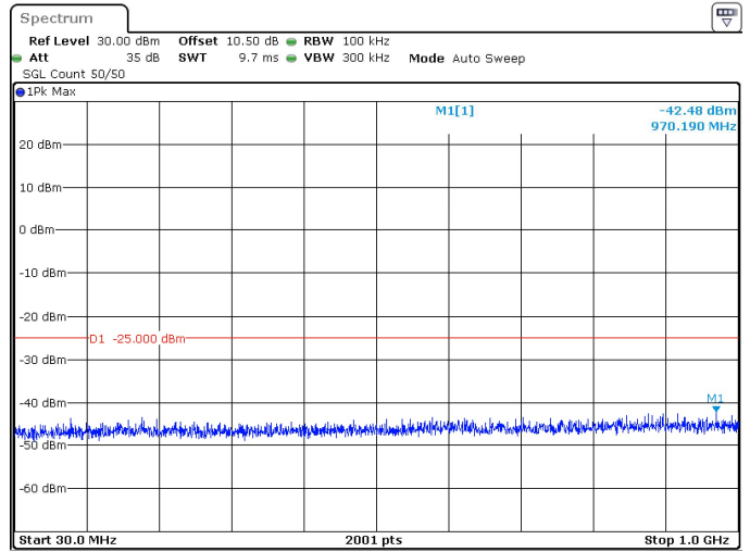
90MHz_30kHz_2644.98MHz_DFT-s-OFDM QPSK_RB1@0 -42.48 dBm
