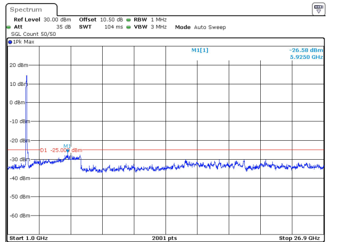
90MHz_30kHz_2541MHz_DFT-s-OFDM QPSK_RB243@0 -26.58 dBm
