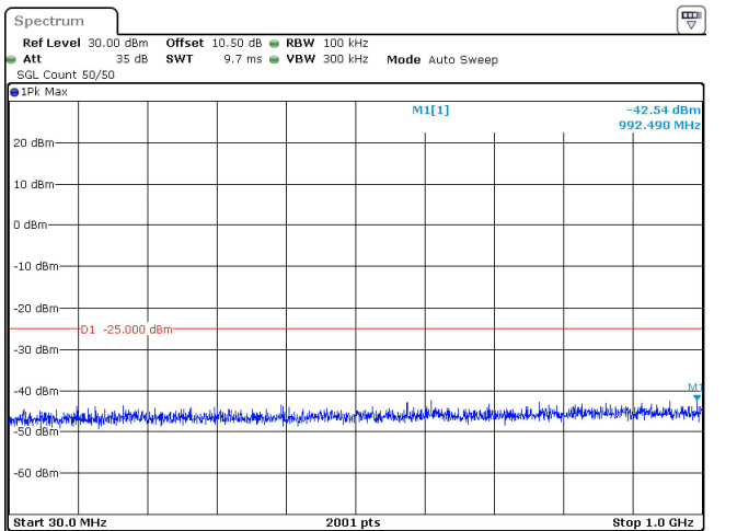
90MHz_30kHz_2541MHz_DFT-s-OFDM QPSK_RB1@244 -42.54 dBm
