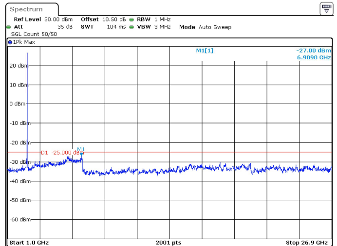
90MHz_30kHz_2541MHz_DFT-s-OFDM QPSK_RB1@244 -27.00 dBm
