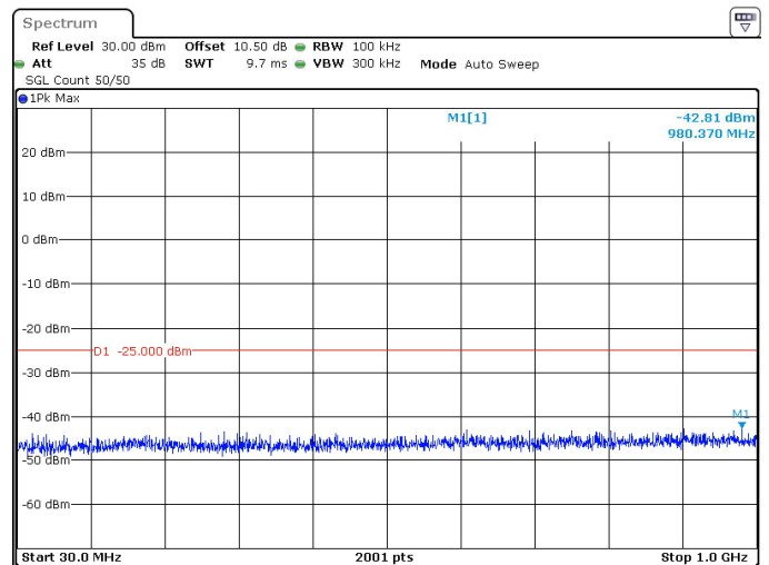
80MHz_30kHz_2649.99MHz_DFT-s-OFDM QPSK_RB1@216 -42.81 dBm
