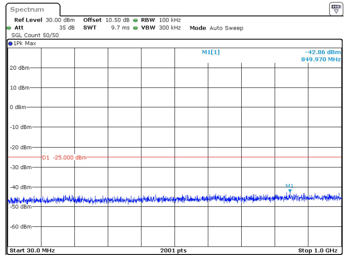
90MHz_30kHz_2541MHz_DFT-s-OFDM QPSK_RB1@0 -42.86 dBm
