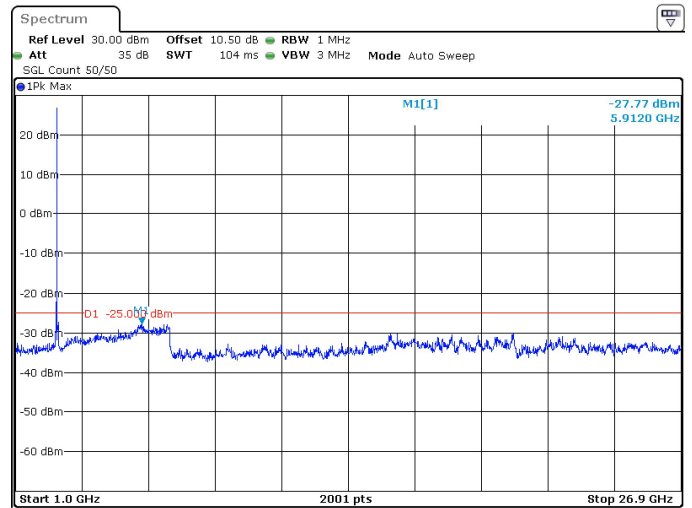
80MHz_30kHz_2649.99MHz_DFT-s-OFDM QPSK_RB1@0 -27.77 dBm
