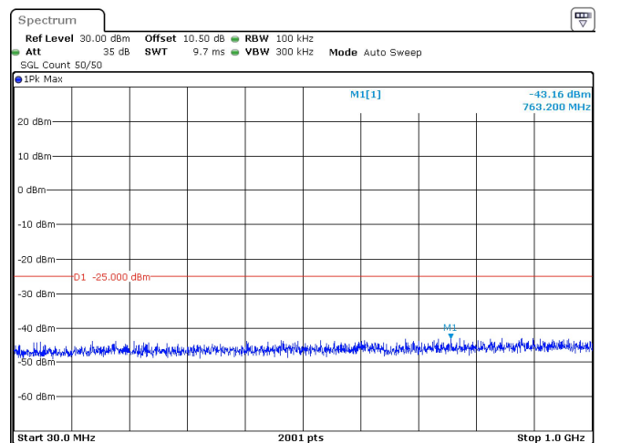
80MHz_30kHz_2649.99MHz_DFT-s-OFDM QPSK_RB216@0 -43.16 dBm
