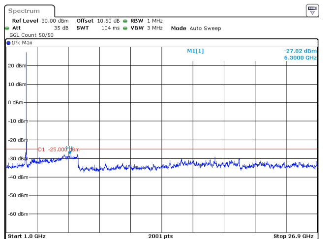
80MHz_30kHz_2649.99MHz_DFT-s-OFDM QPSK_RB1@216 -27.82 dBm
