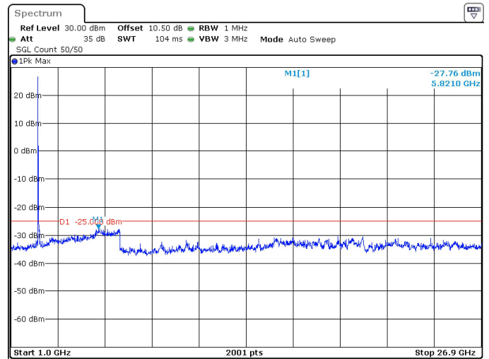
60MHz_30kHz_2526MHz_DFT-s-OFDM QPSK_RB1@0 -27.76 dBm
