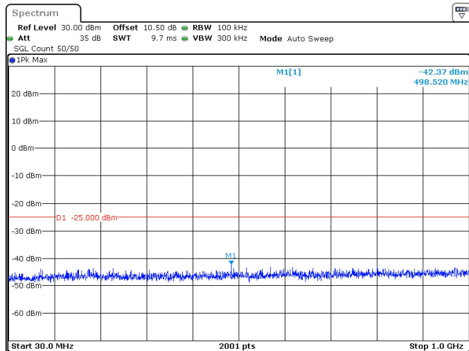
60MHz_30kHz_2526MHz_DFT-s-OFDM QPSK_RB1@0 -42.37 dBm
