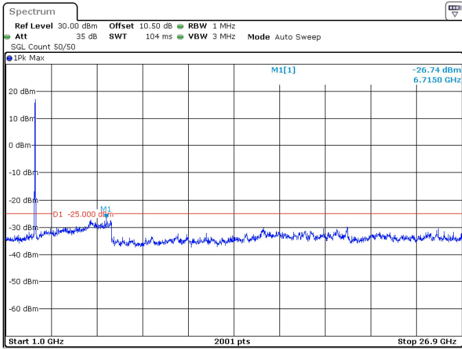
40MHz_30kHz_2670MHz_DFT-s-OFDM QPSK_RB100@0 -26.74 dBm
