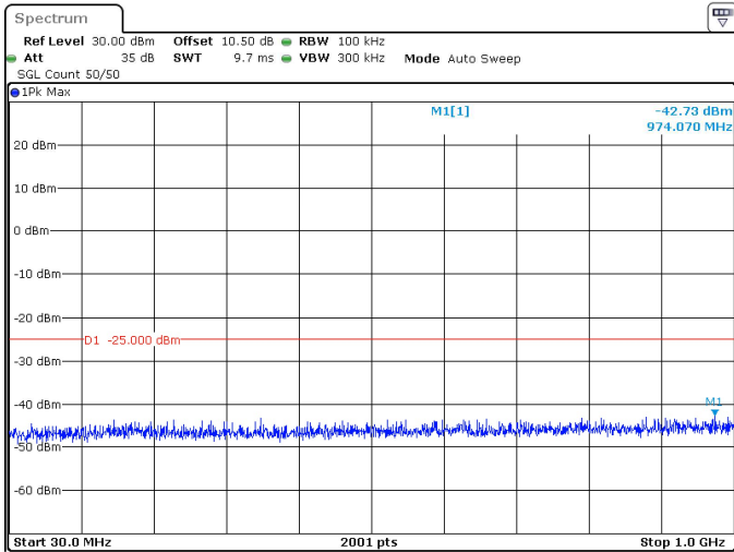
40MHz_30kHz_2670MHz_DFT-s-OFDM QPSK_RB1@0 -42.73 dBm
