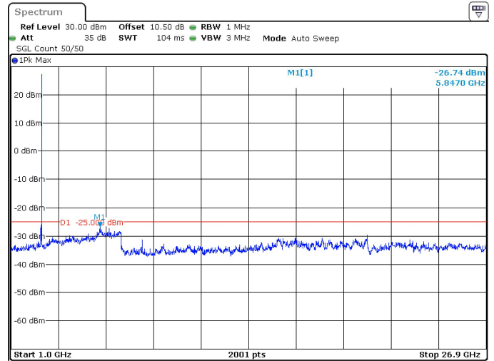
40MHz_30kHz_2670MHz_DFT-s-OFDM QPSK_RB1@105 -26.74 dBm
