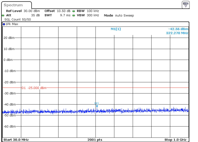
40MHz_30kHz_2670MHz_DFT-s-OFDM QPSK_RB1@105 -42.56 dBm
