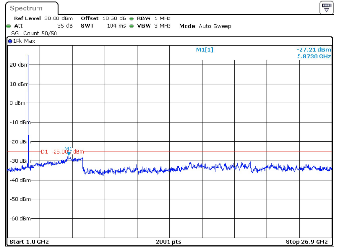
40MHz_30kHz_2670MHz_DFT-s-OFDM QPSK_RB1@0 -27.21 dBm
