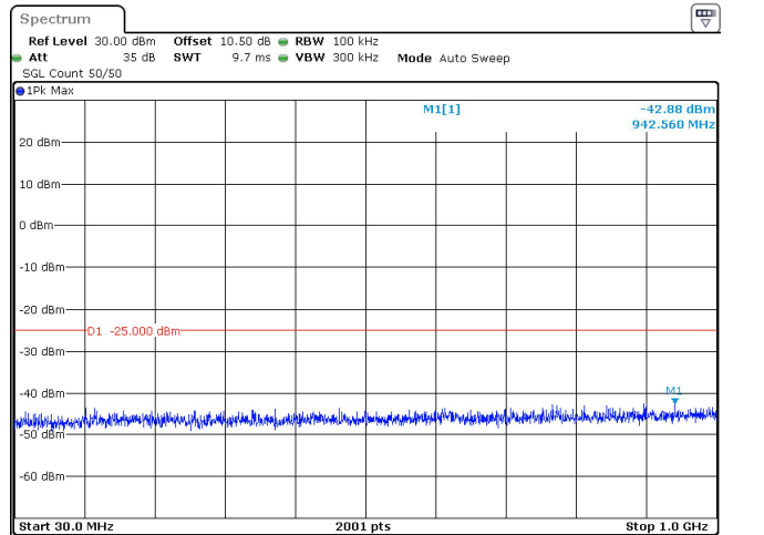
20MHz_30kHz_2679.99MHz_DFT-s-OFDM QPSK_RB50@0 -42.88 dBm
