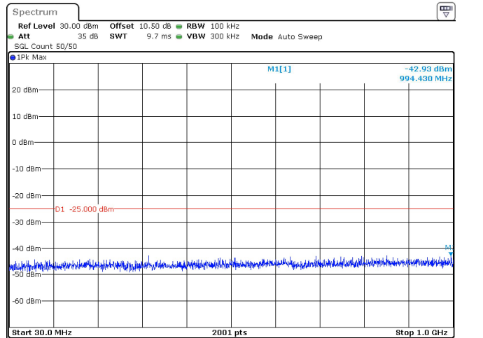
20MHz_30kHz_2592.99MHz_DFT-s-OFDM QPSK_RB50@0 -42.93 dBm
