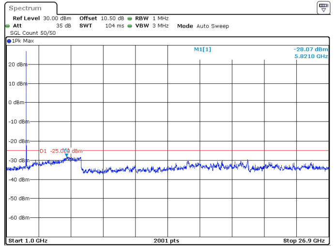
20MHz_30kHz_2592.99MHz_DFT-s-OFDM QPSK_RB1@0 -28.07 dBm
