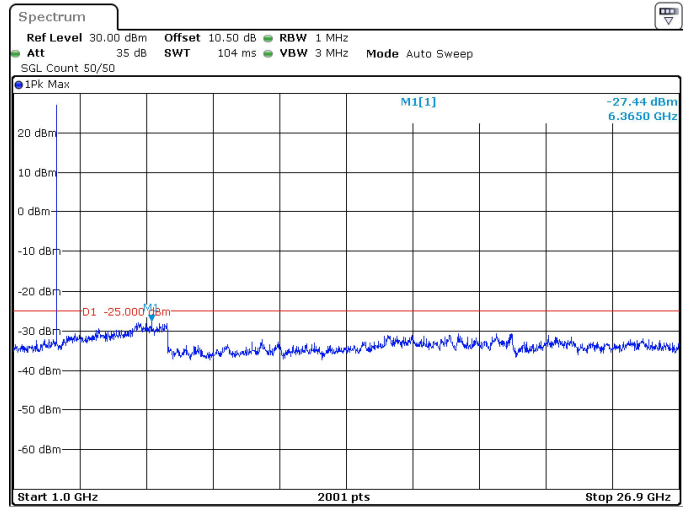
20MHz_30kHz_2679.99MHz_DFT-s-OFDM QPSK_RB1@0 -27.44 dBm
