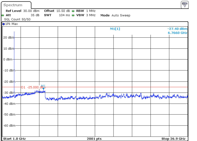
20MHz_30kHz_2679.99MHz_DFT-s-OFDM QPSK_RB1@50 -27.40 dBm
