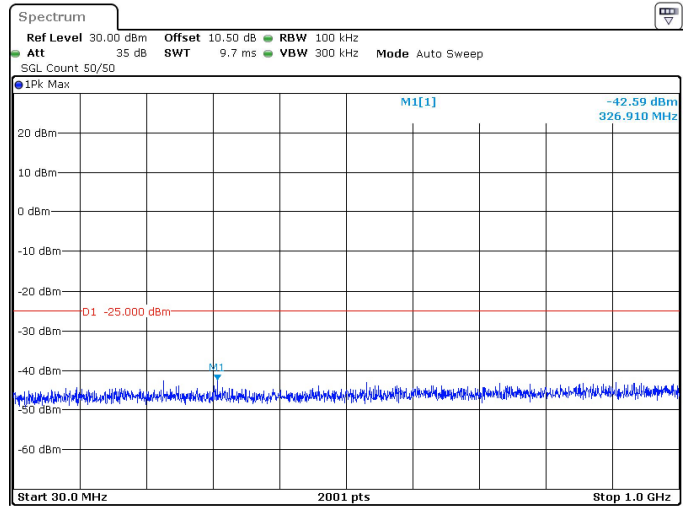
20MHz_30kHz_2679.99MHz_DFT-s-OFDM QPSK_RB1@50 -42.59 dBm
