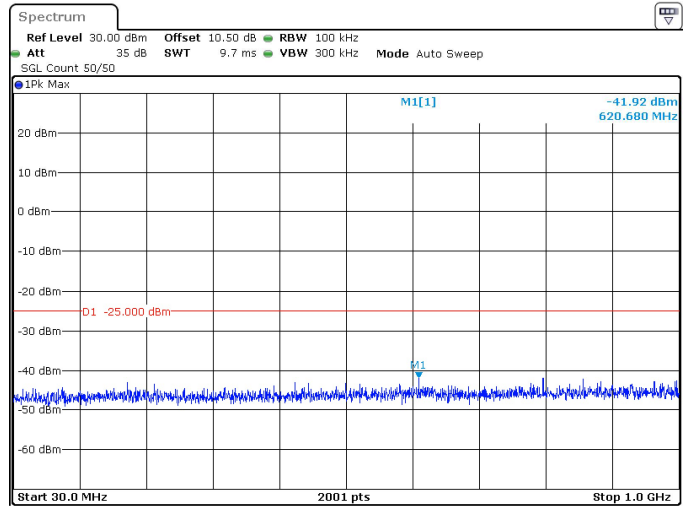
20MHz_30kHz_2592.99MHz_DFT-s-OFDM QPSK_RB1@50 -41.92 dBm
