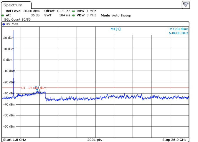
20MHz_30kHz_2592.99MHz_DFT-s-OFDM QPSK_RB1@50 -27.68 dBm
