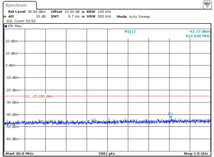
15MHz_30kHz_2682.48MHz_DFT-s-OFDM QPSK_RB1@0 -42.77 dBm
