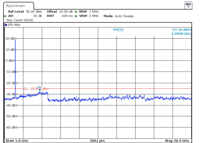
20MHz_30kHz_2506.02MHz_DFT-s-OFDM QPSK_RB50@0 -27.16 dBm
