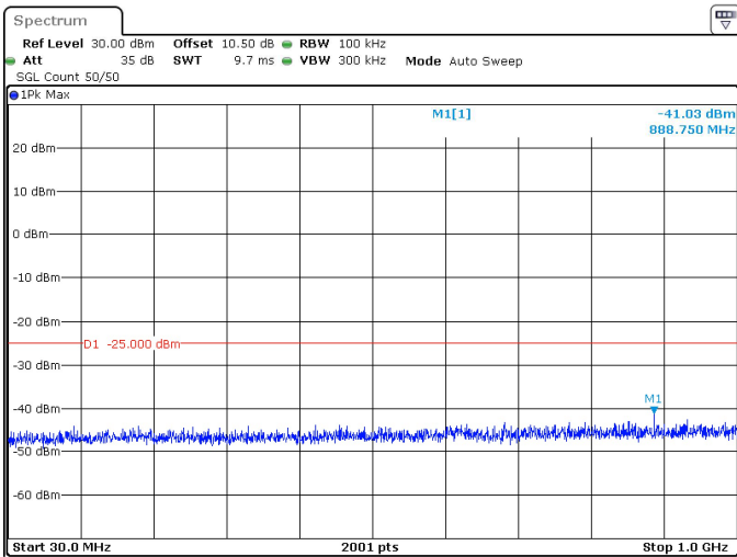
20MHz_30kHz_2506.02MHz_DFT-s-OFDM QPSK_RB1@0 -41.03 dBm
