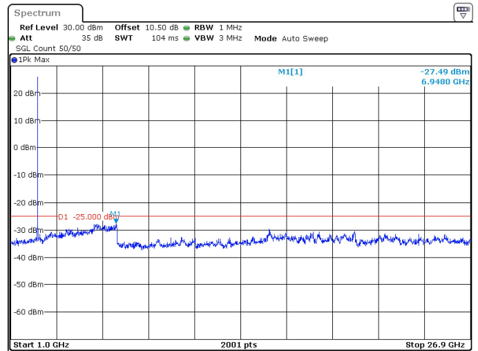
20MHz_30kHz_2506.02MHz_DFT-s-OFDM QPSK_RB1@50 -27.49 dBm
