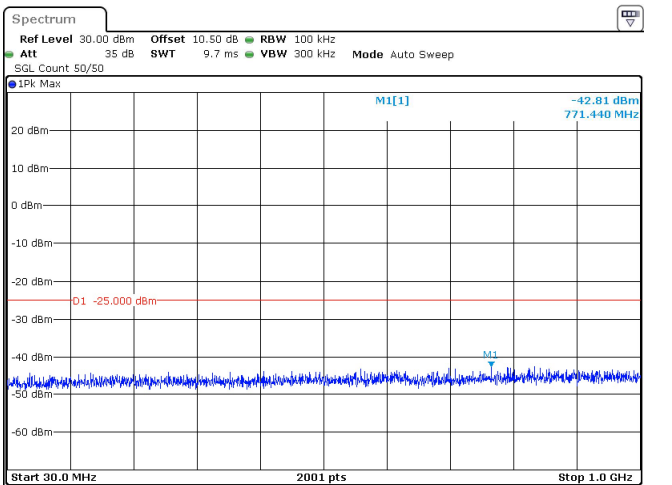
20MHz_30kHz_2506.02MHz_DFT-s-OFDM QPSK_RB1@50 -42.81 dBm
