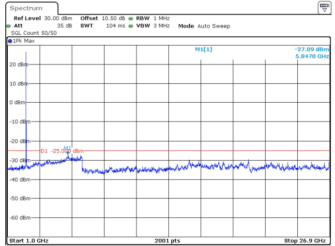
20MHz_30kHz_2506.02MHz_DFT-s-OFDM QPSK_RB1@0 -27.09 dBm
