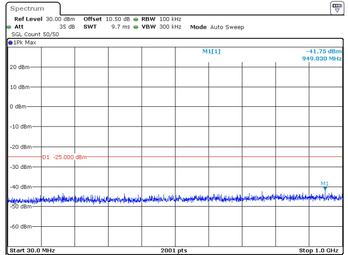
10MHz_30kHz_2592.99MHz_DFT-s-OFDM QPSK_RB1@0 -41.75 dBm
