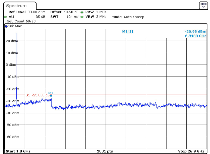
15MHz_30kHz_2503.5MHz_DFT-s-OFDM QPSK_RB1@0 -26.98 dBm
