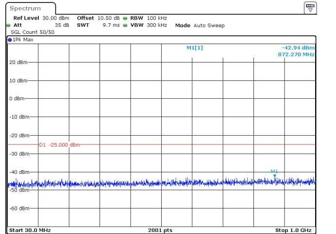
10MHz_30kHz_2685MHz_DFT-s-OFDM QPSK_RB24@0 -42.94 dBm
