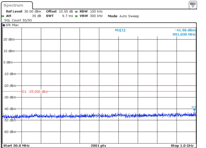
10MHz_30kHz_2685MHz_DFT-s-OFDM QPSK_RB1@23 -41.96 dBm
