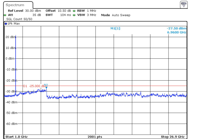
10MHz_30kHz_2592.99MHz_DFT-s-OFDM QPSK_RB24@0 -27.50 dBm
