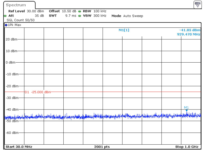
10MHz_30kHz_2685MHz_DFT-s-OFDM QPSK_RB1@0 -41.85 dBm
