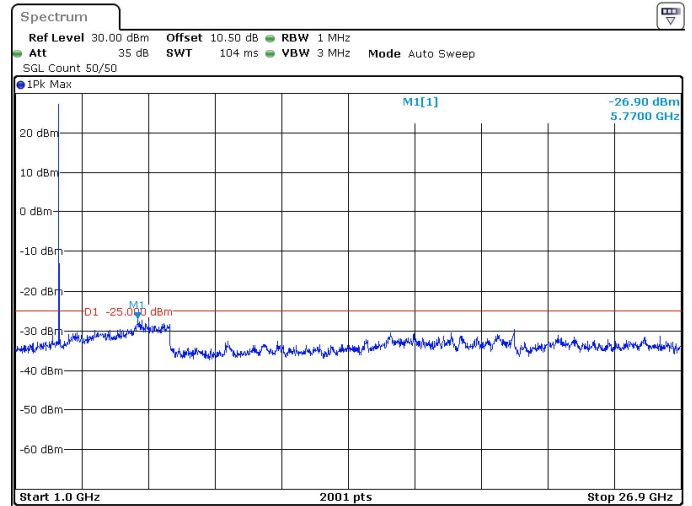
10MHz_30kHz_2685MHz_DFT-s-OFDM QPSK_RB1@23 -26.90 dBm
