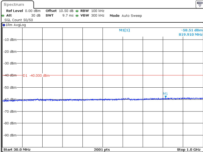
10MHz_30kHz_2355MHz_DFT-s-OFDM QPSK_RB1@0 -58.51 dBm
