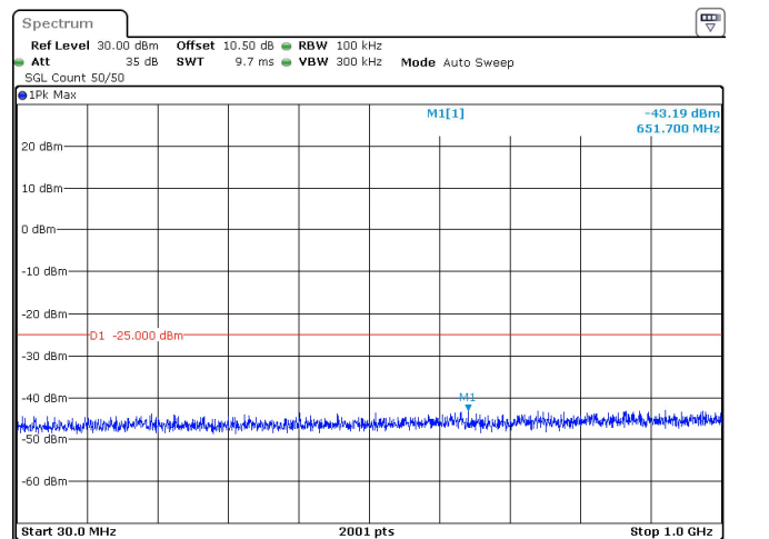
10MHz_30kHz_2501.01MHz_DFT-s-OFDM QPSK_RB24@0 -43.19 dBm
