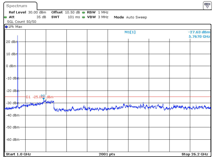
20MHz_30kHz_2595MHz_DFT-s-OFDM QPSK_RB1@0 -27.63 dBm
