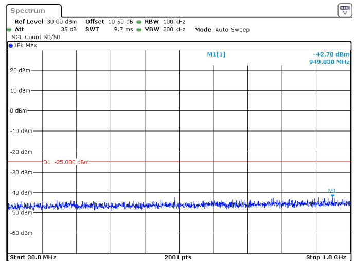
20MHz_30kHz_2580MHz_DFT-s-OFDM QPSK_RB1@50 -42.70 dBm
