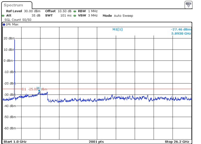
20MHz_30kHz_2610MHz_DFT-s-OFDM QPSK_RB50@0 -27.46 dBm
