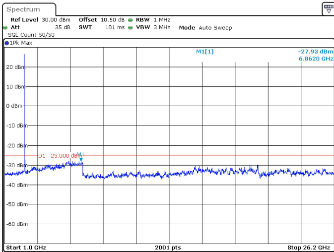
20MHz_30kHz_2580MHz_DFT-s-OFDM QPSK_RB1@0 -27.93 dBm
