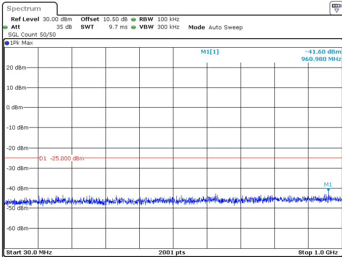
20MHz_30kHz_2610MHz_DFT-s-OFDM QPSK_RB1@50 -41.60 dBm
