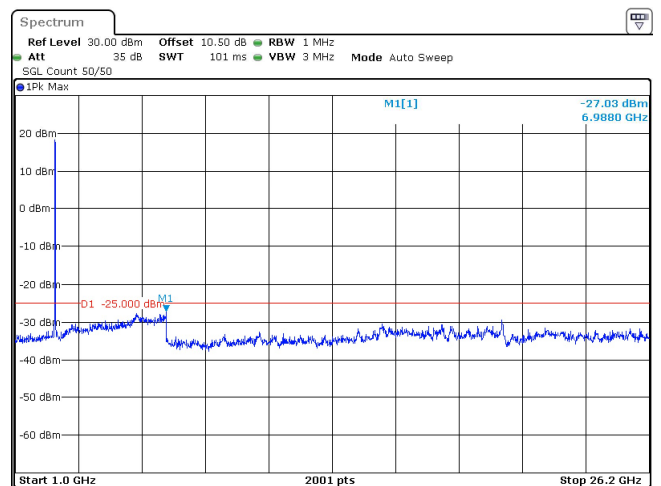
20MHz_30kHz_2580MHz_DFT-s-OFDM QPSK_RB50@0 -27.03 dBm
