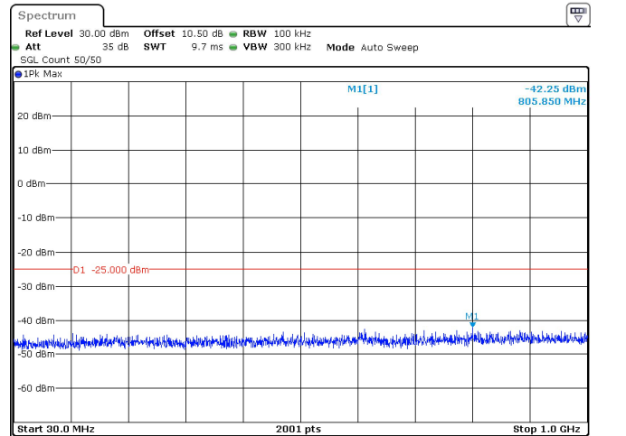
20MHz_30kHz_2610MHz_DFT-s-OFDM QPSK_RB50@0 -42.25 dBm
