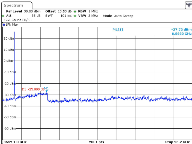
20MHz_30kHz_2595MHz_DFT-s-OFDM QPSK_RB1@50 -27.73 dBm
