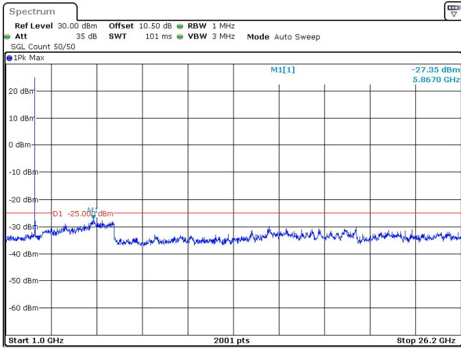
20MHz_30kHz_2610MHz_DFT-s-OFDM QPSK_RB1@0 -27.35 dBm
