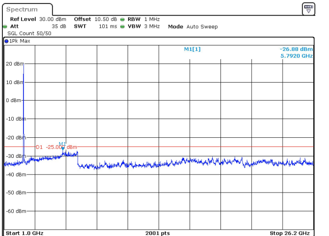
20MHz_30kHz_2595MHz_DFT-s-OFDM QPSK_RB50@0 -26.88 dBm
