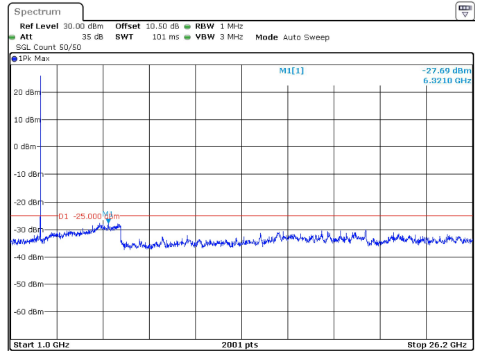
20MHz_30kHz_2610MHz_DFT-s-OFDM QPSK_RB1@50 -27.69 dBm
