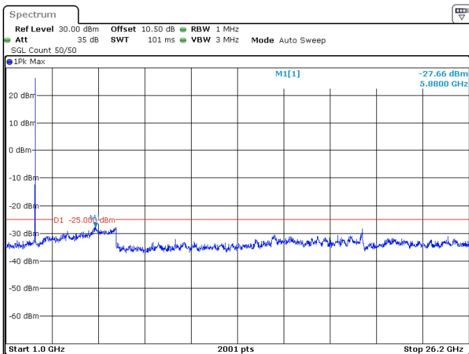
20MHz_30kHz_2580MHz_DFT-s-OFDM QPSK_RB1@50 -27.66 dBm
