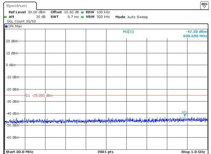
20MHz_30kHz_2595MHz_DFT-s-OFDM QPSK_RB1@50 -42.50 dBm
