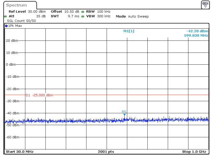
20MHz_30kHz_2610MHz_DFT-s-OFDM QPSK_RB1@0 -42.20 dBm
