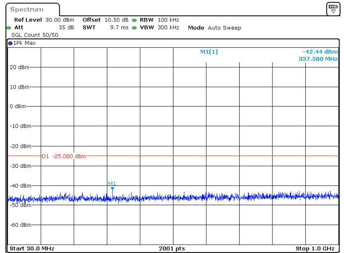
20MHz_30kHz_2580MHz_DFT-s-OFDM QPSK_RB1@0 -42.44 dBm
