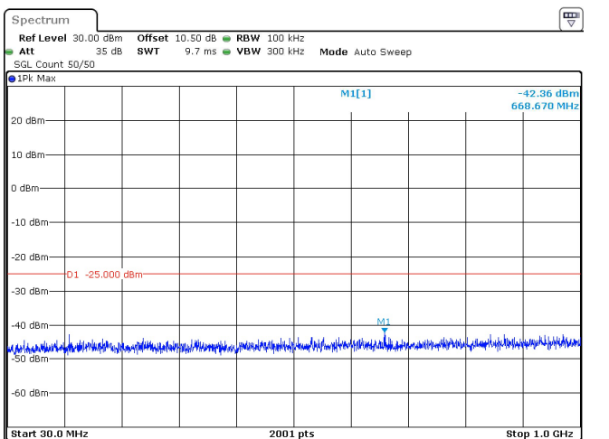
20MHz_30kHz_2580MHz_DFT-s-OFDM QPSK_RB50@0 -42.36 dBm
