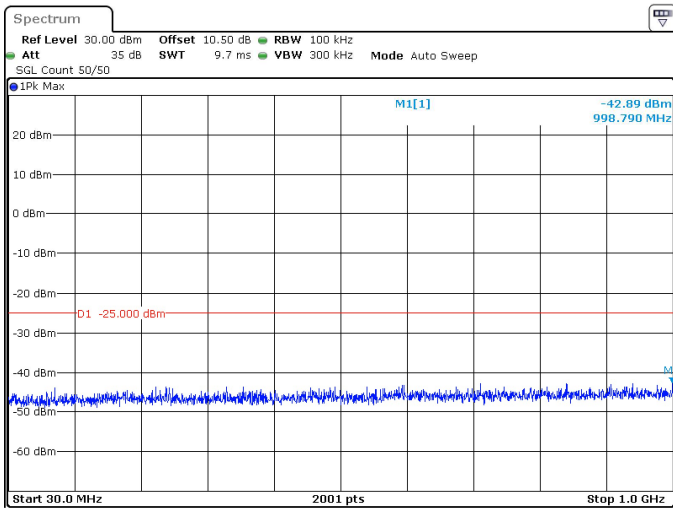
20MHz_30kHz_2595MHz_DFT-s-OFDM QPSK_RB1@0 -42.89 dBm
