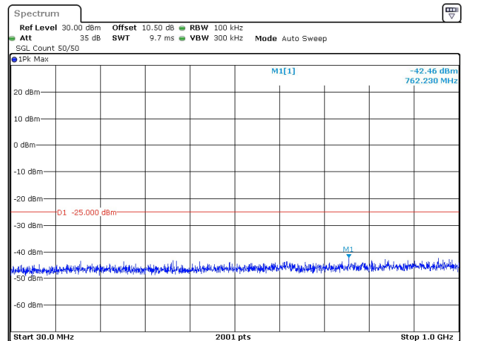
20MHz_30kHz_2595MHz_DFT-s-OFDM QPSK_RB50@0 -42.46 dBm
