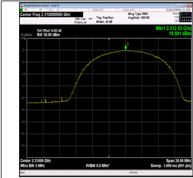
40(2305-2315)-10MHz-QPSK-38750-25RB#25-PASS
