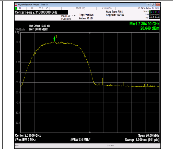
40(2305-2315)-10MHz-64QAM-38750-1RB#0-PASS
