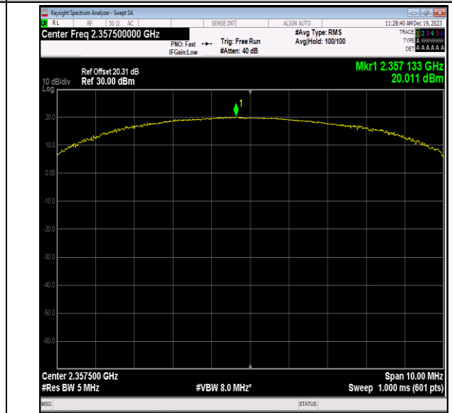
40(2350-2360)-5MHz-QPSK-39225-25RB#25-PASS
