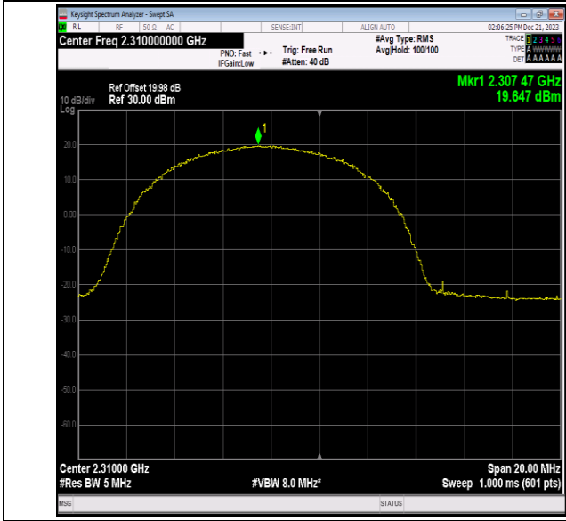
40(2305-2315)-10MHz-16QAM-38750-25RB#12-PASS
