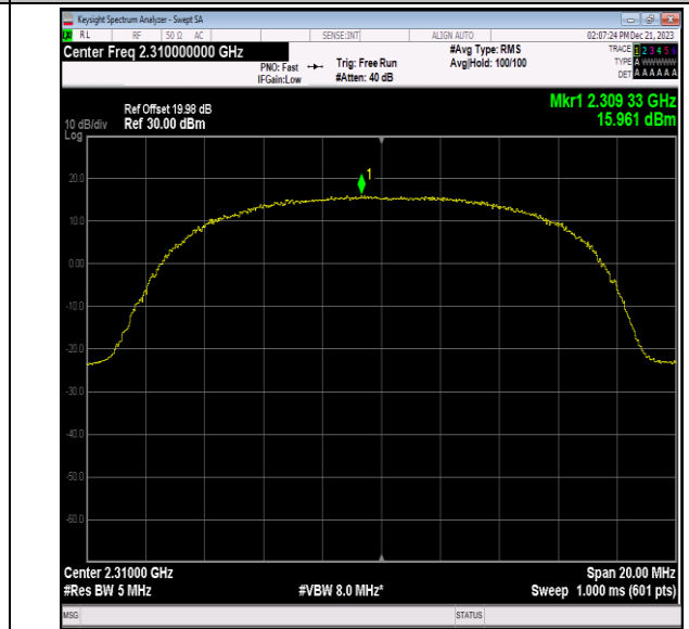
40(2305-2315)-10MHz-64QAM-38750-50RB#0-PASS
