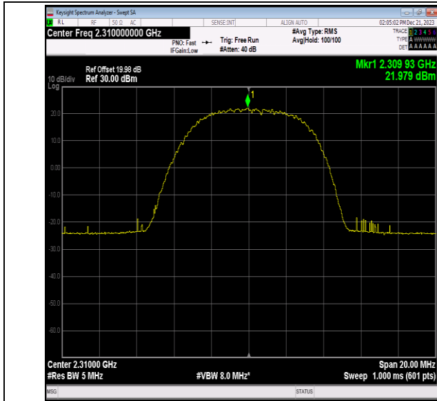
40(2305-2315)-10MHz-QPSK-38750-1RB#24-PASS
