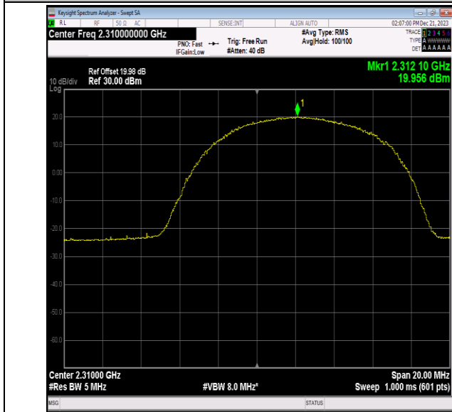
40(2305-2315)-10MHz-64QAM-38750-25RB#25-PASS
