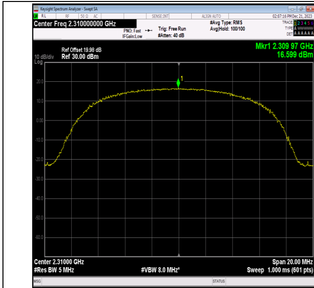
40(2305-2315)-10MHz-16QAM-38750-50RB#0-PASS
