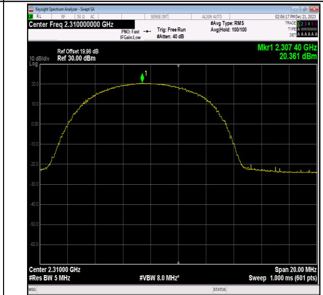
40(2305-2315)-10MHz-QPSK-38750-25RB#12-PASS
