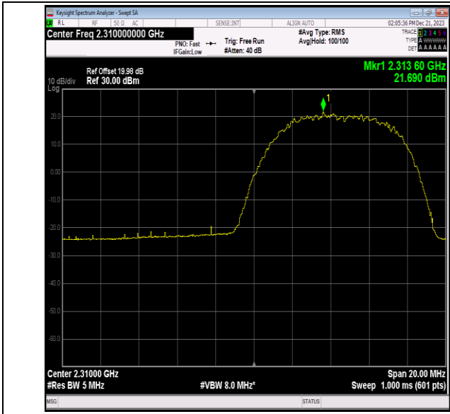
40(2305-2315)-10MHz-16QAM-38750-1RB#49-PASS
