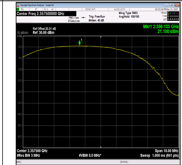
40(2350-2360)-5MHz-QPSK-39225-12RB#6-PASS
