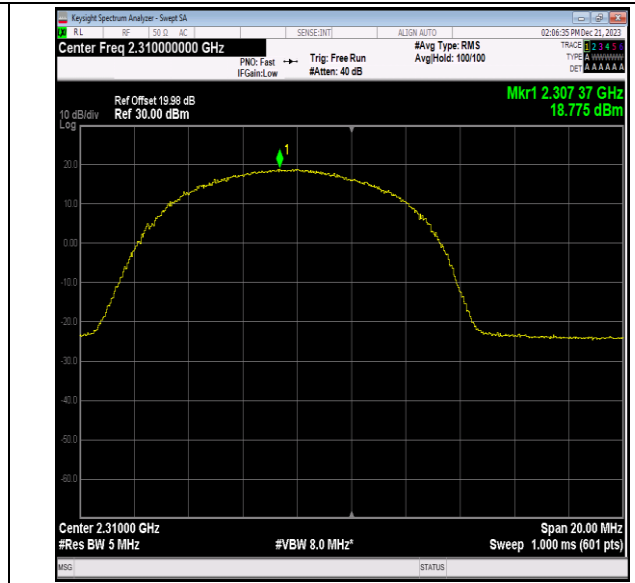
40(2305-2315)-10MHz-64QAM-38750-25RB#12-PASS
