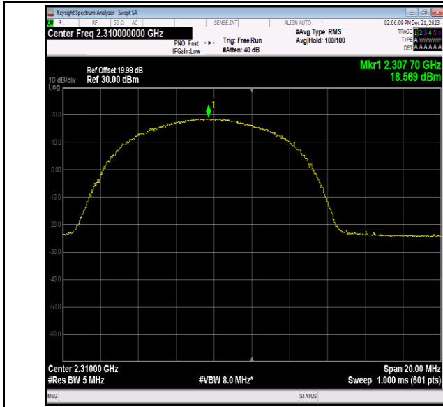
40(2305-2315)-10MHz-64QAM-38750-25RB#0-PASS
