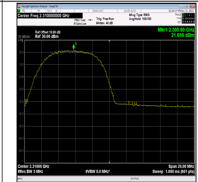
40(2305-2315)-10MHz-QPSK-38750-1RB#0-PASS
