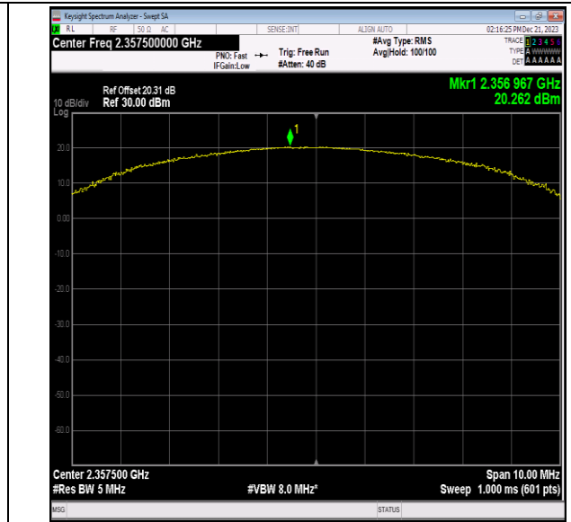
40(2350-2360)-5MHz-QPSK-39225-25RB#0-PASS
