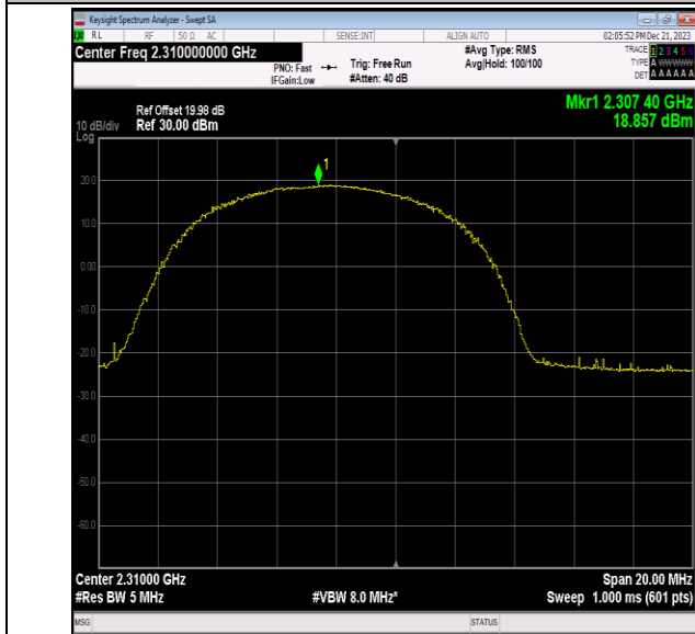
40(2305-2315)-10MHz-QPSK-38750-25RB#0-PASS
