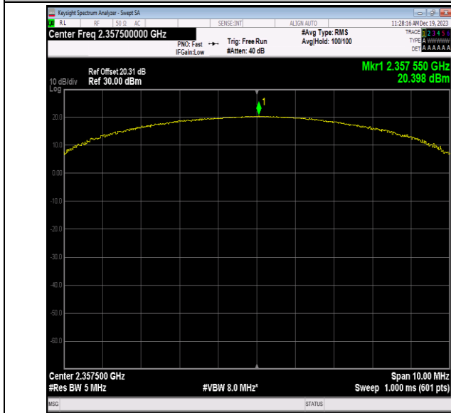
40(2350-2360)-5MHz-QPSK-39225-25RB#12-PASS
