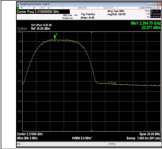
40(2305-2315)-10MHz-16QAM-38750-1RB#0-PASS
