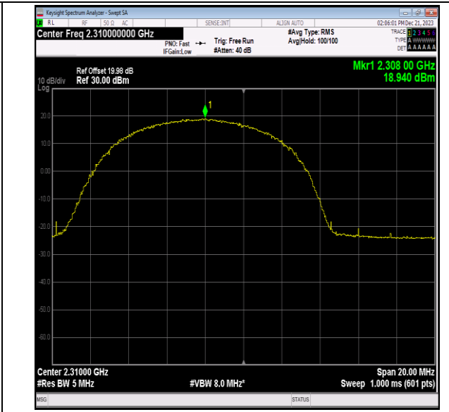
40(2305-2315)-10MHz-16QAM-38750-25RB#0-PASS
