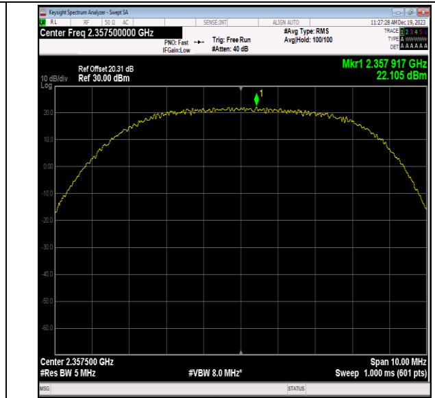
40(2350-2360)-5MHz-QPSK-39225-1RB#49-PASS
