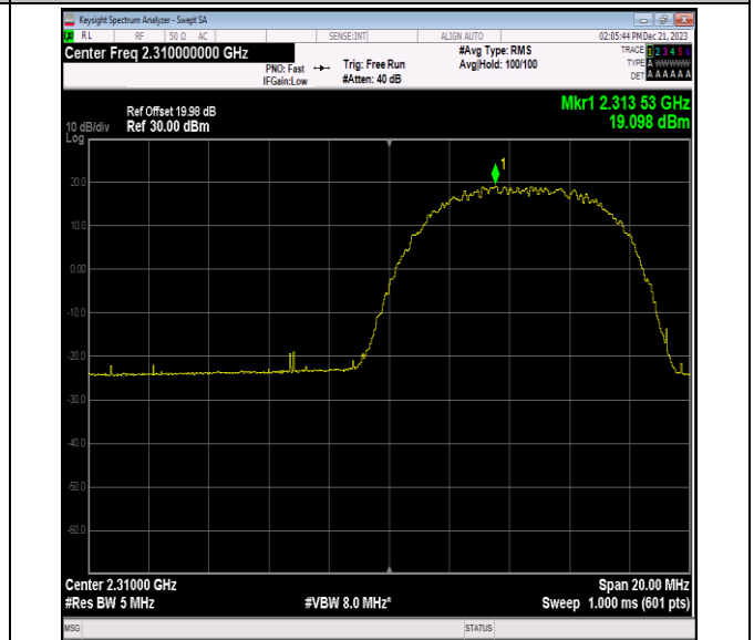
40(2305-2315)-10MHz-64QAM-38750-1RB#49-PASS
