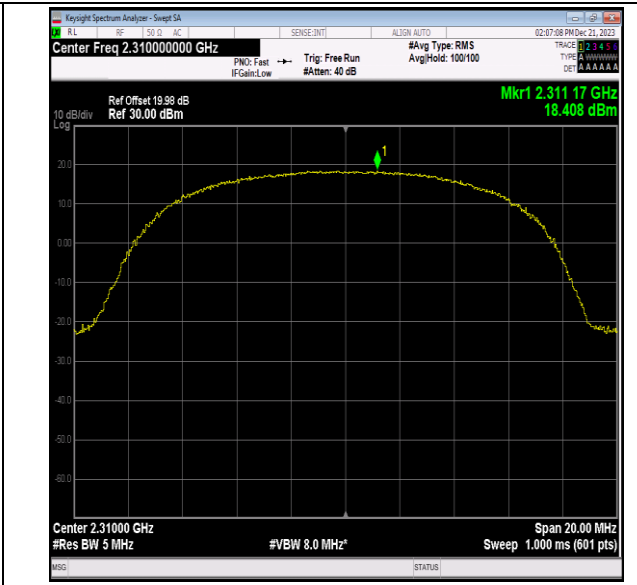
40(2305-2315)-10MHz-QPSK-38750-50RB#0-PASS
