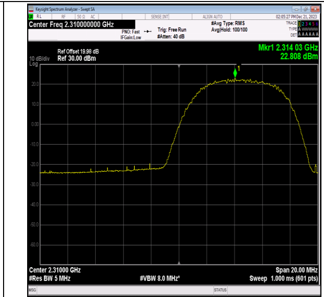
40(2305-2315)-10MHz-QPSK-38750-1RB#49-PASS
