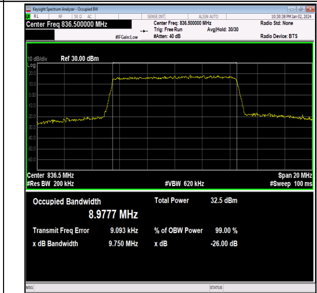
26(824-849)-10MHz-QPSK-26915-50RB#0-PASS
