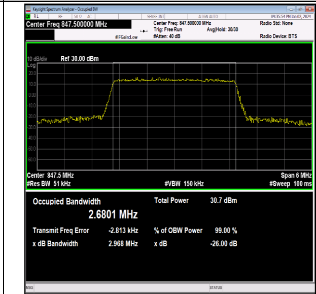
26(824-849)-3MHz-16QAM-27025-15RB#0-PASS
