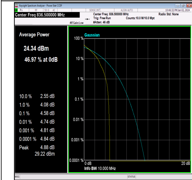
26(824-849)-10MHz-QPSK-26915-1RB#0-PASS
