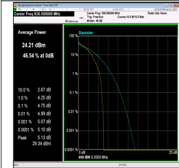
26(824-849)-5MHz-QPSK-26915-1RB#0-PASS
