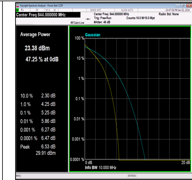
26(824-849)-10MHz-QPSK-26990-50RB#0-PASS
