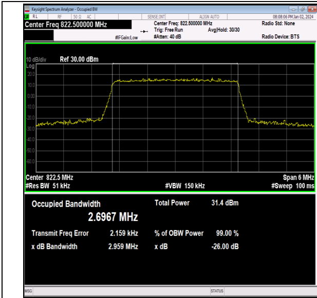
26(814-824)-3MHz-QPSK-26775-15RB#0-PASS
