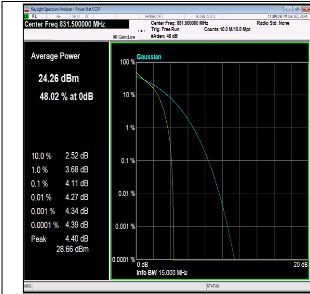
26(824-849)-15MHz-QPSK-26865-1RB#0-PASS
