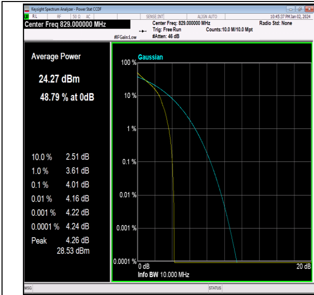
26(824-849)-10MHz-QPSK-26840-1RB#0-PASS
