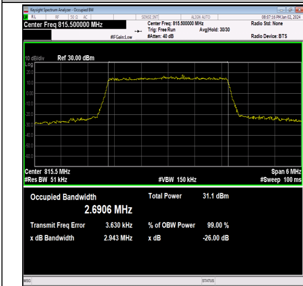
26(814-824)-3MHz-QPSK-26705-15RB#0-PASS
