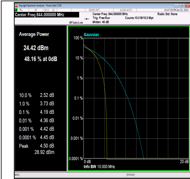
26(824-849)-10MHz-QPSK-26990-1RB#0-PASS
