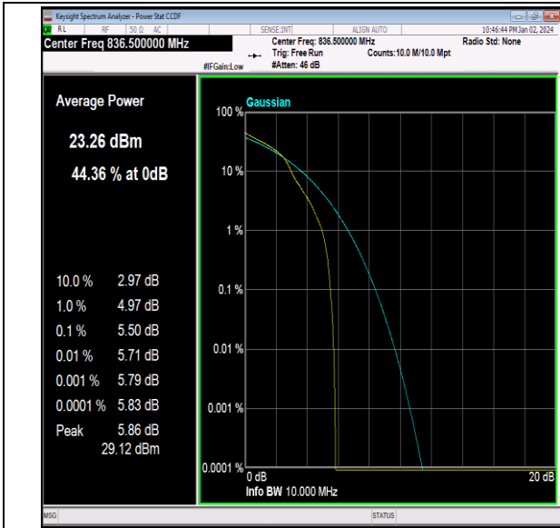
26(824-849)-10MHz-16QAM-26915-1RB#0-PASS
