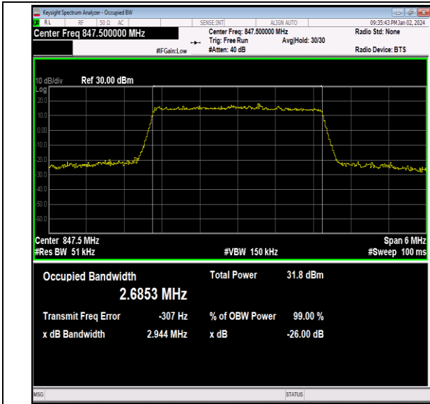
26(824-849)-3MHz-QPSK-27025-15RB#0-PASS
