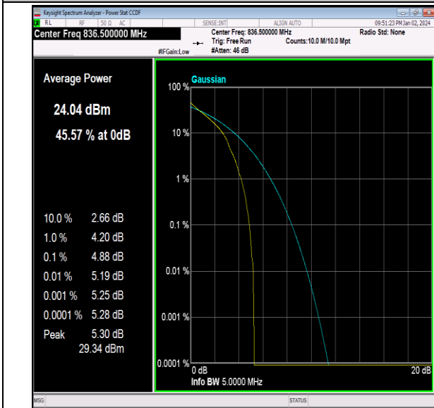
26(824-849)-3MHz-QPSK-26915-1RB#0-PASS
