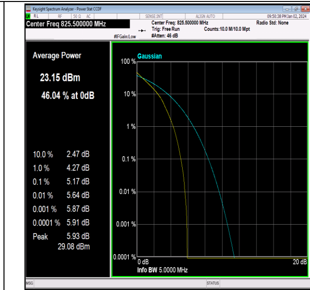
26(824-849)-3MHz-QPSK-26805-15RB#0-PASS
