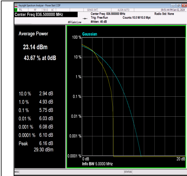
26(824-849)-3MHz-16QAM-26915-1RB#0-PASS
