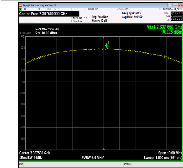
40(2305-2315)-5MHz-16QAM-38725-25RB#25-PASS
