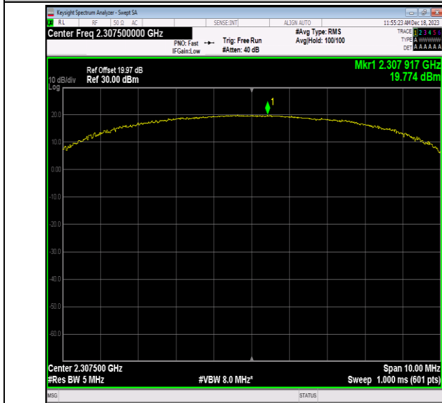
40(2305-2315)-5MHz-QPSK-38725-50RB#0-PASS
