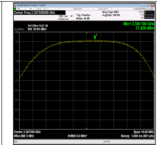
40(2305-2315)-5MHz-QPSK-38725-1RB#12-PASS
