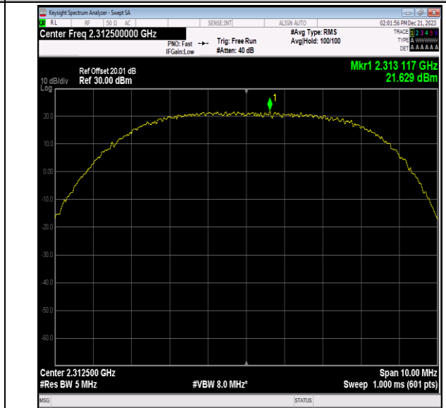
40(2305-2315)-5MHz-QPSK-38775-1RB#12-PASS
