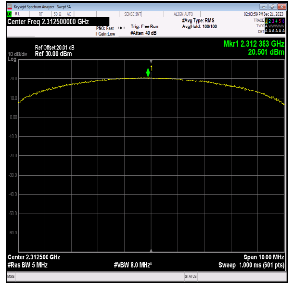
40(2305-2315)-5MHz-QPSK-38775-25RB#0-PASS
