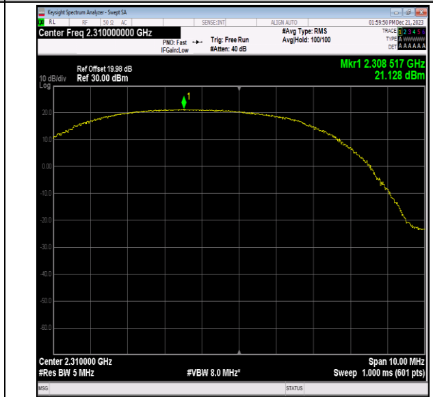
40(2305-2315)-5MHz-QPSK-38750-12RB#0-PASS
