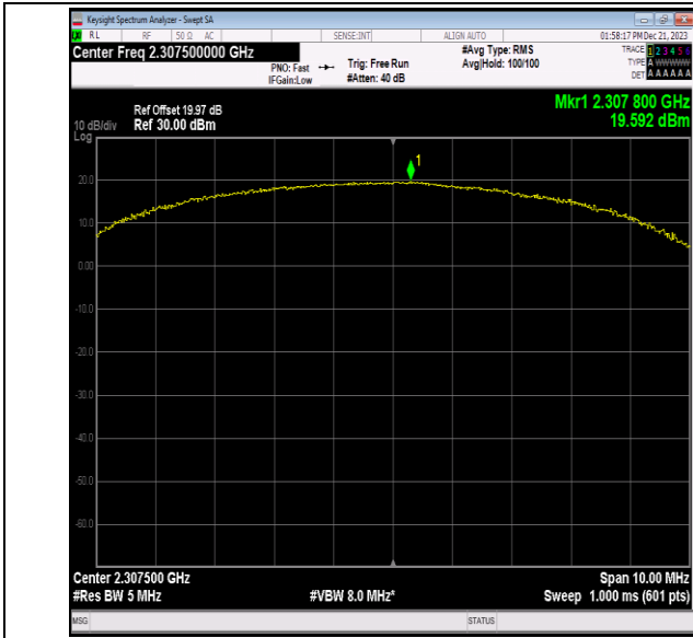
40(2305-2315)-5MHz-16QAM-38725-25RB#0-PASS
