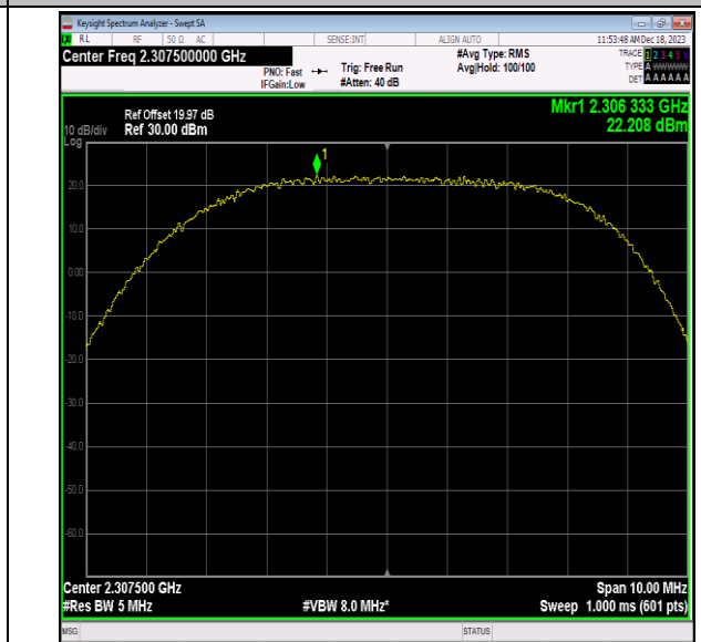
40(2305-2315)-5MHz-QPSK-38725-1RB#49-PASS
