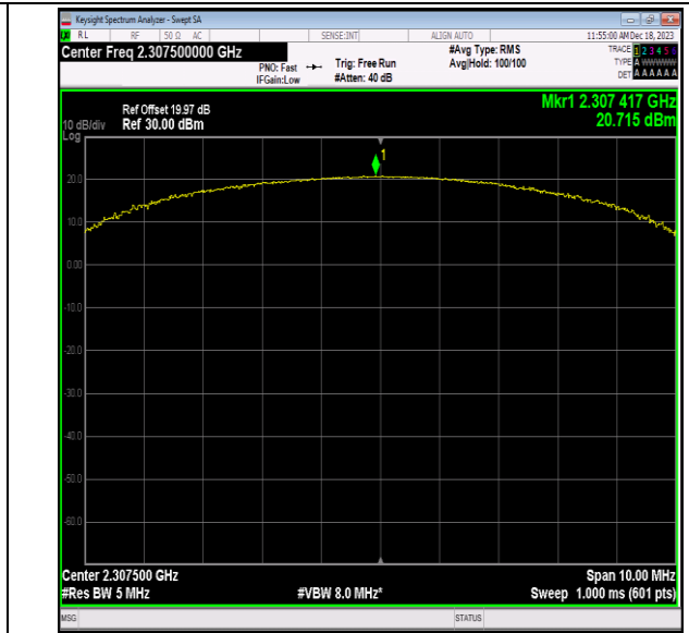
40(2305-2315)-5MHz-QPSK-38725-25RB#25-PASS
