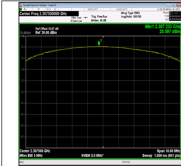
40(2305-2315)-5MHz-QPSK-38725-25RB#12-PASS
