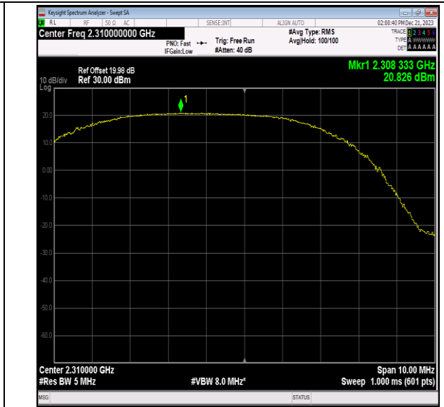
40(2305-2315)-5MHz-QPSK-38750-12RB#11-PASS
