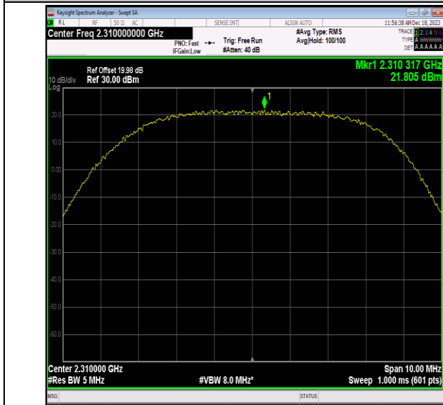
40(2305-2315)-5MHz-QPSK-38750-1RB#49-PASS
