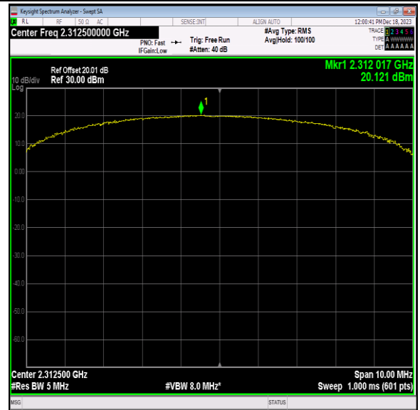
40(2305-2315)-5MHz-QPSK-38775-25RB#25-PASS
