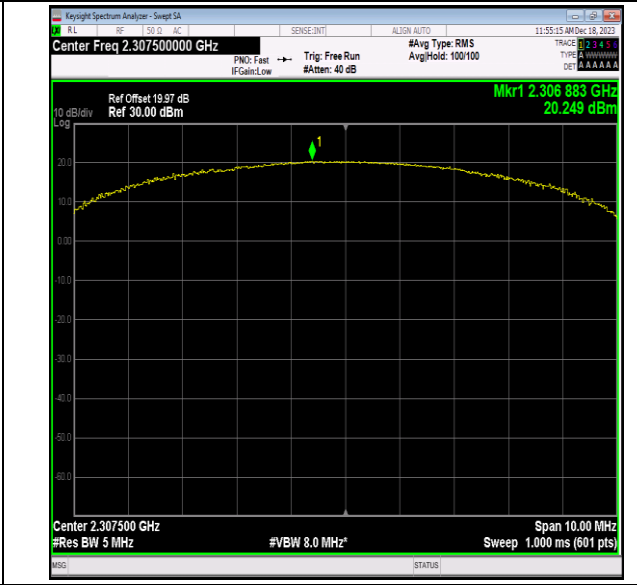
40(2305-2315)-5MHz-64QAM-38725-25RB#25-PASS
