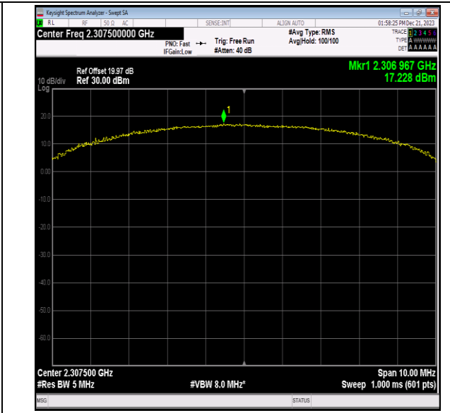
40(2305-2315)-5MHz-64QAM-38725-25RB#0-PASS
