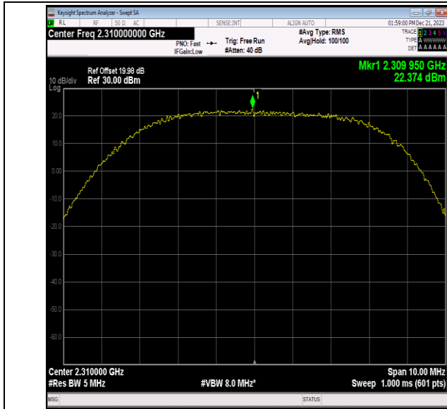
40(2305-2315)-5MHz-QPSK-38750-1RB#12-PASS
