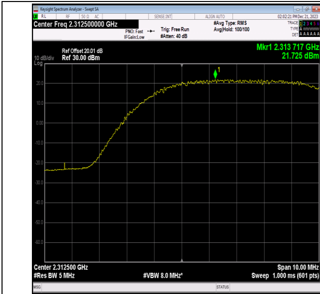
40(2305-2315)-5MHz-QPSK-38775-1RB#24-PASS
