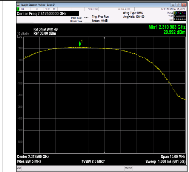
40(2305-2315)-5MHz-QPSK-38775-12RB#6-PASS
