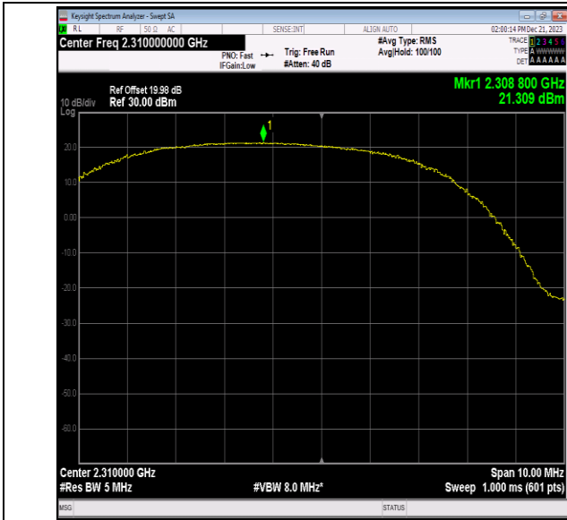
40(2305-2315)-5MHz-QPSK-38750-12RB#6-PASS
