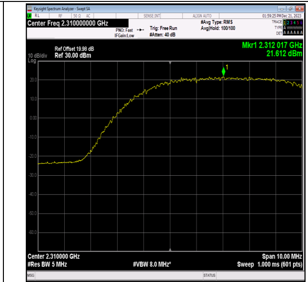
40(2305-2315)-5MHz-QPSK-38750-1RB#24-PASS
