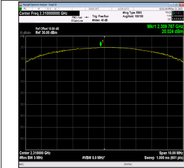
40(2305-2315)-5MHz-QPSK-38750-25RB#0-PASS
