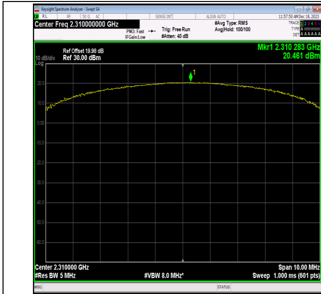
40(2305-2315)-5MHz-QPSK-38750-25RB#25-PASS
