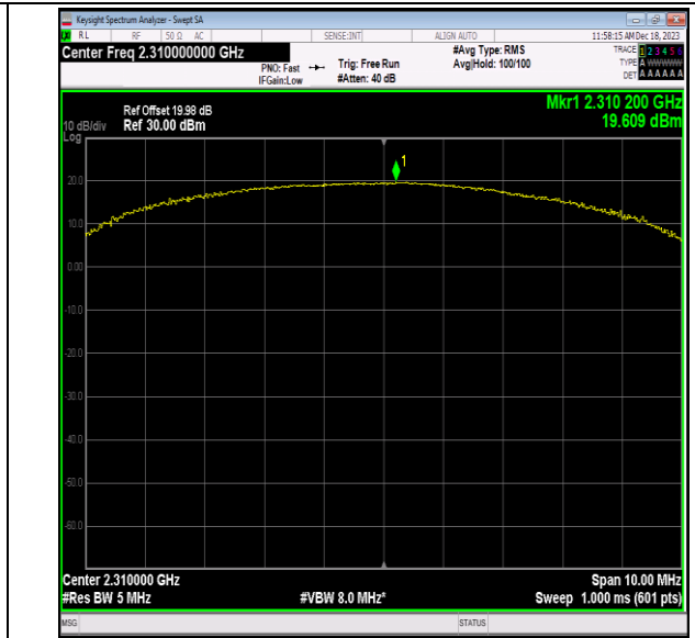
40(2305-2315)-5MHz-QPSK-38750-50RB#0-PASS
