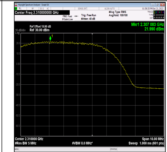
40(2305-2315)-5MHz-QPSK-38750-1RB#0-PASS
