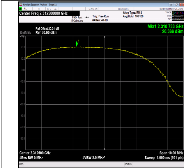
40(2305-2315)-5MHz-QPSK-38775-12RB#0-PASS
