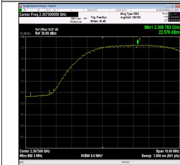
40(2305-2315)-5MHz-QPSK-38725-1RB#24-PASS
