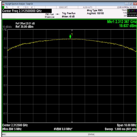
40(2305-2315)-5MHz-QPSK-38775-25RB#12-PASS
