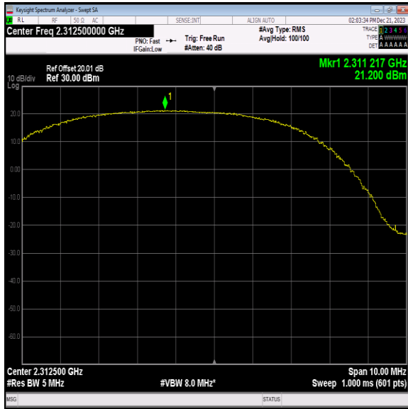
40(2305-2315)-5MHz-QPSK-38775-12RB#11-PASS
