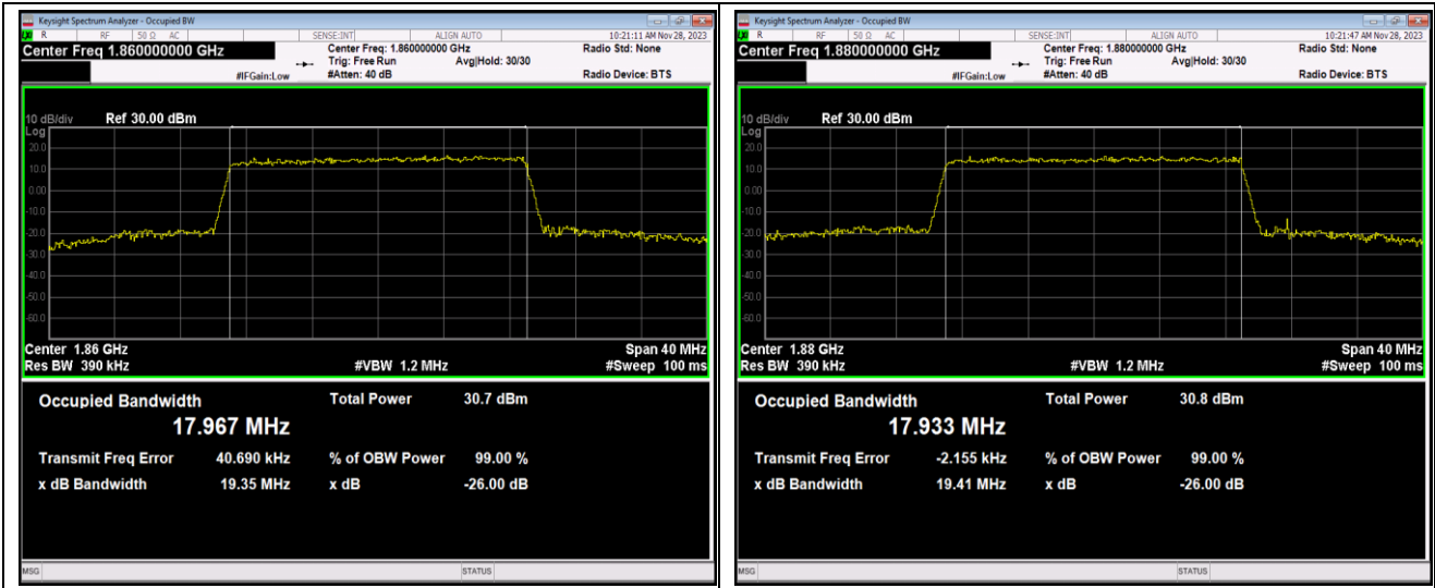
Band2-20MHz-16QAM-19100-100RB#0
