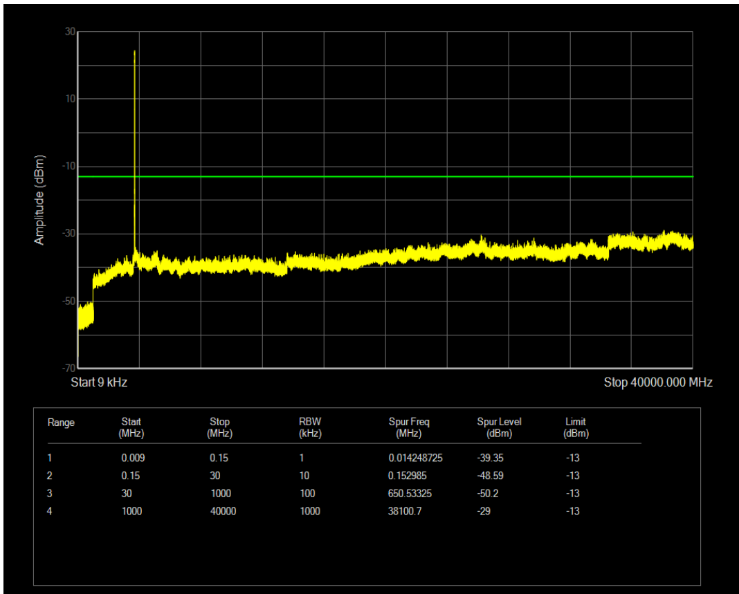
n77(3700-3980) SCS=30kHz DFT_QPSK BW=10MHz Channel=647000 RB=1@0
