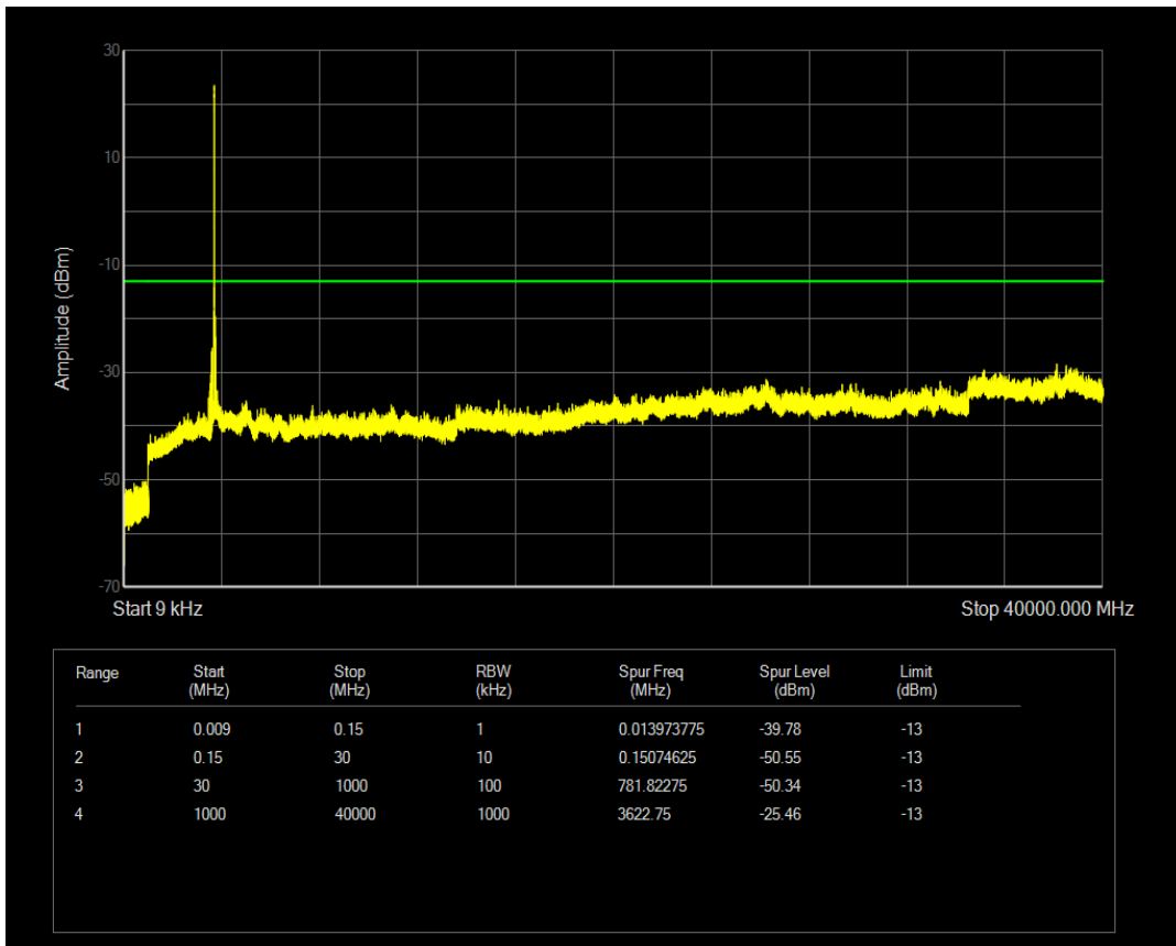
n77(3700-3980) SCS=15kHz DFT_QPSK BW=10MHz Channel=647000 RB=1@0
