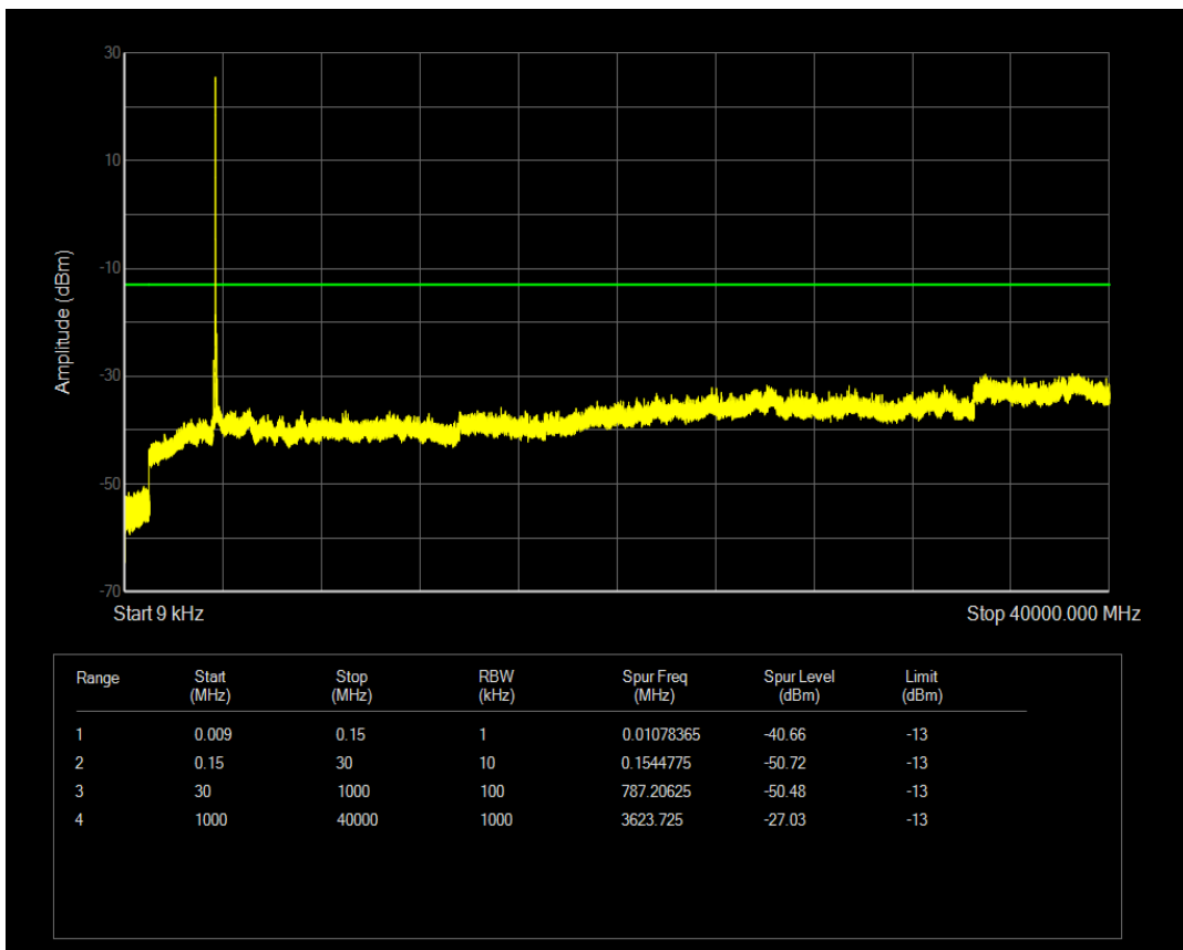
n77(3700-3980) SCS=15kHz DFT_QPSK BW=10MHz Channel=647000 RB=1@51
