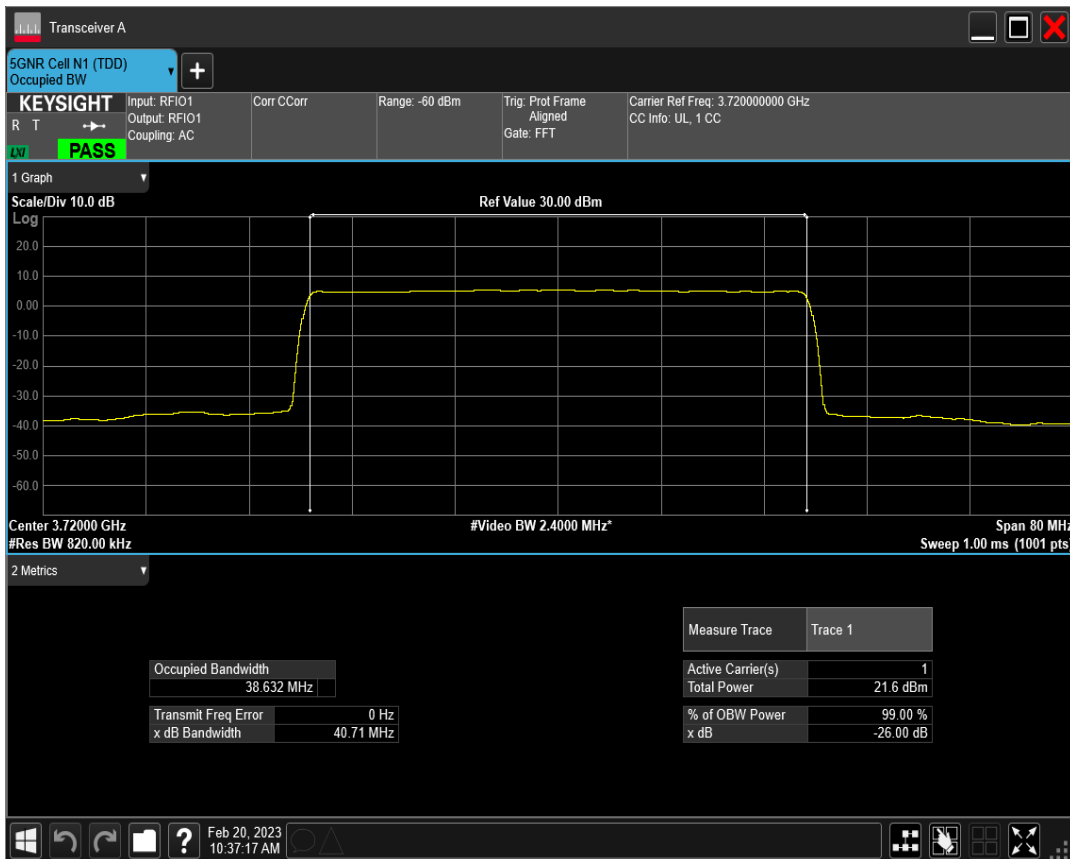
n77(3700-3980) SCS=15kHz CP_QPSK BW=40MHz Channel=648000 RB=216@0
