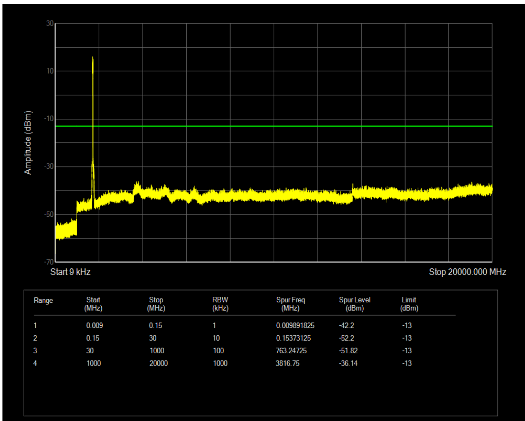
n66 SCS=15kHz DFT_QPSK BW=40MHz Channel=346000 RB=1@0
