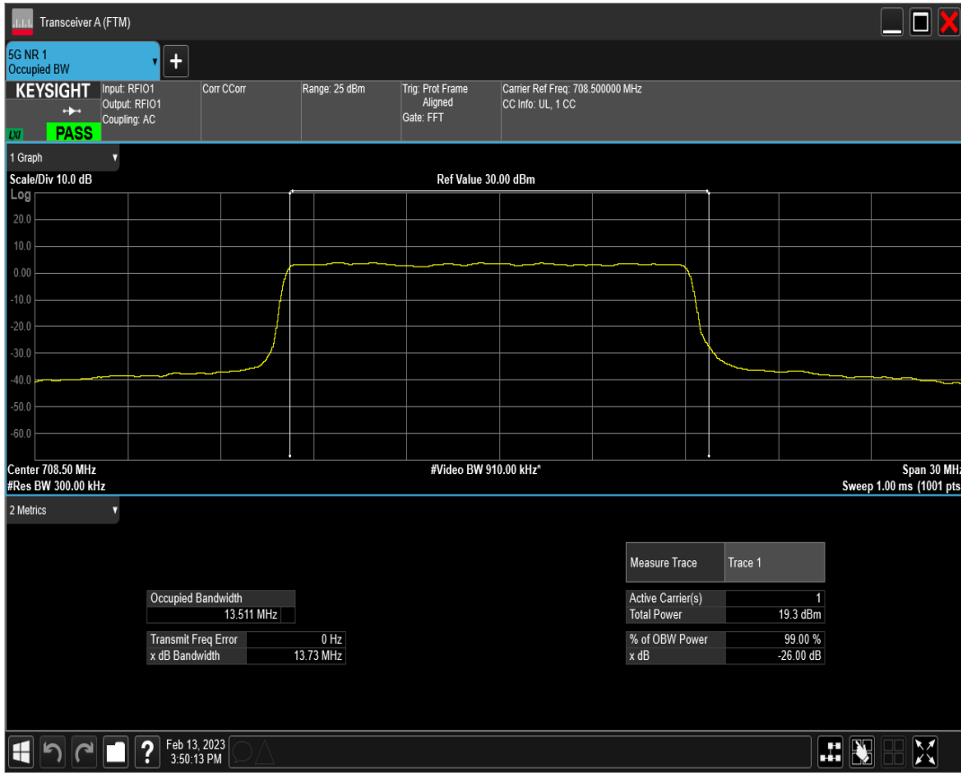
n12 SCS=30kHz CP_QPSK BW=15MHz Channel=141700 RB=38@0
