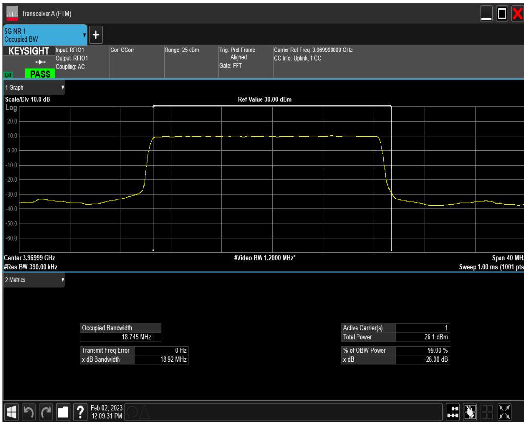
n77(3700-3980) SCS=15kHz DFT_QPSK BW=20MHz Channel=664666 RB=100@0
