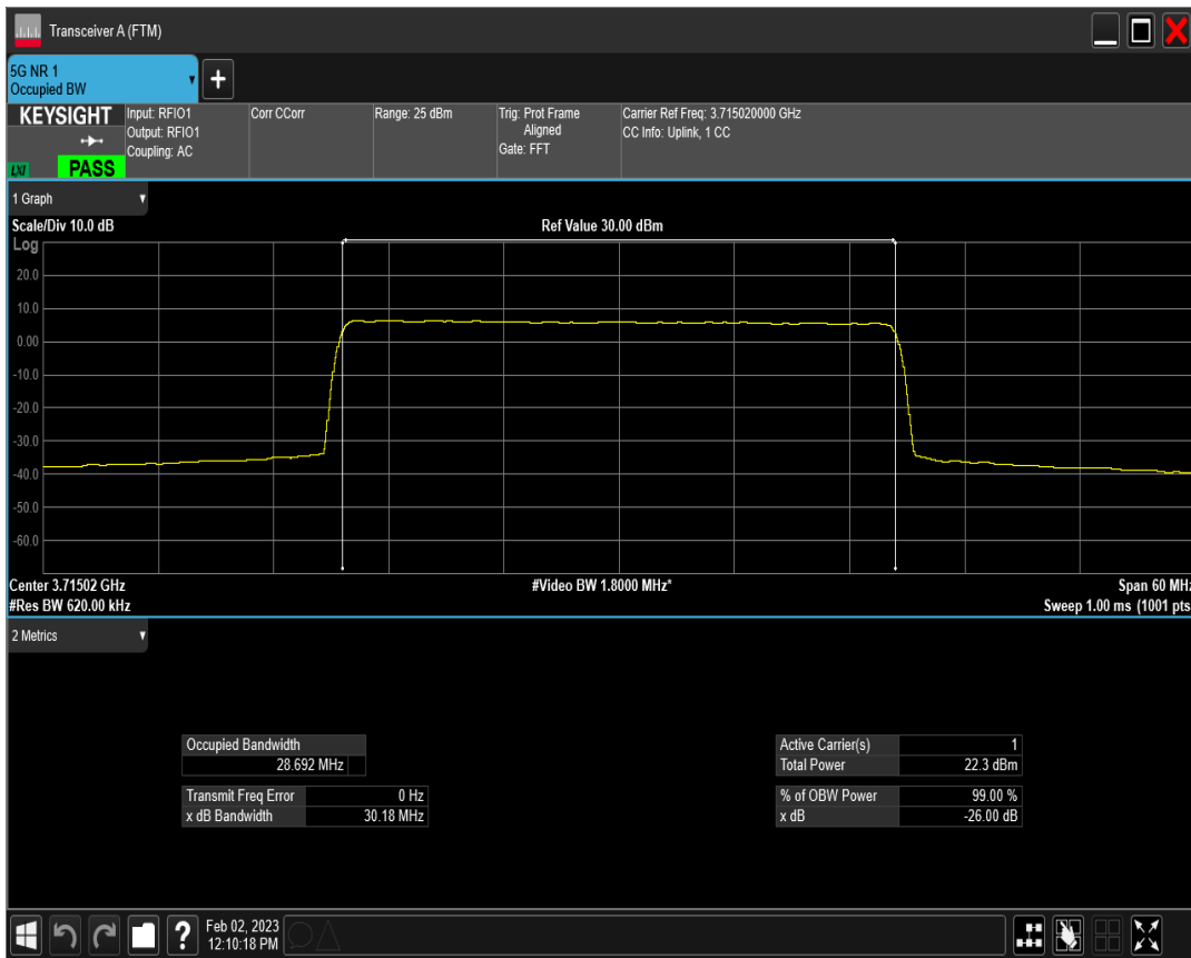
n77(3700-3980) SCS=15kHz CP_QPSK BW=30MHz Channel=647668 RB=160@0
