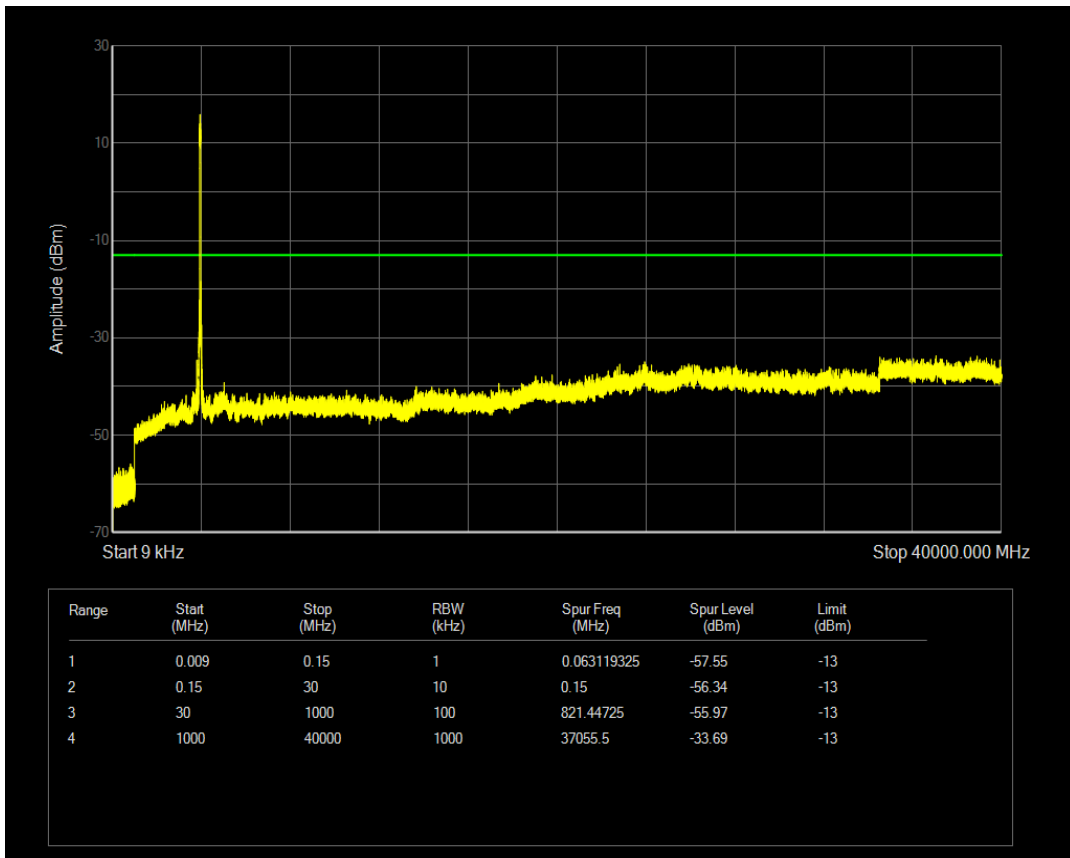
n77(3700-3980) SCS=15kHz DFT_QPSK BW=50MHz Channel=663666 RB=1@0
