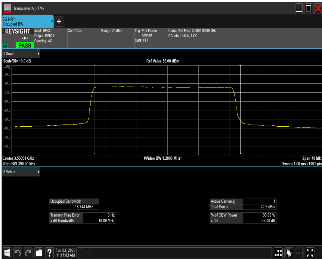
n77(3450-3550) SCS=15kHz CP_QPSK BW=20MHz Channel=633334 RB=106@0
