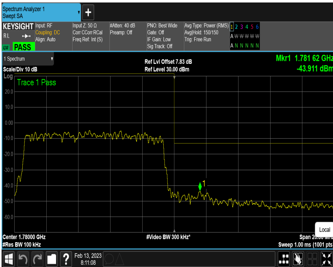
n66 SCS=30kHz DFT_QPSK BW=10MHz Channel=355000 RB=1@23
