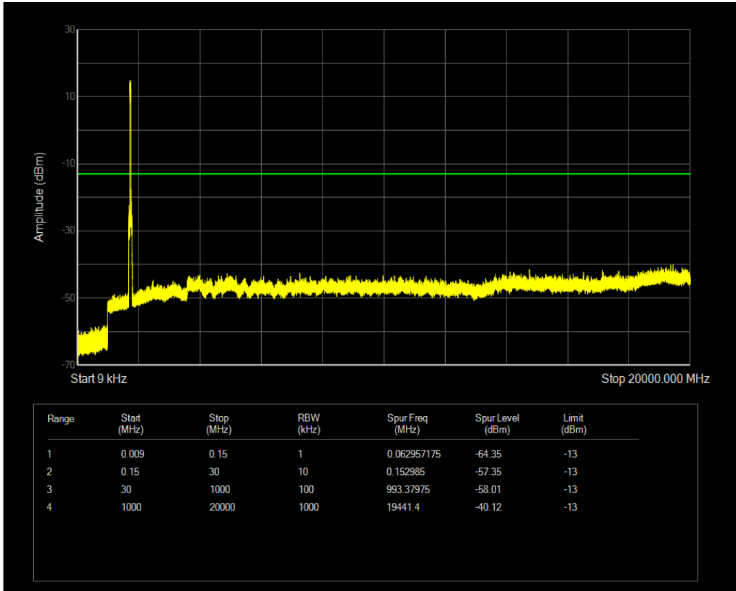
n66 SCS=30kHz DFT_QPSK BW=40MHz Channel=349000 RB=1@0
