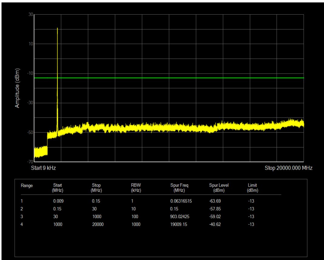
n66 SCS=30kHz DFT_QPSK BW=10MHz Channel=349000 RB=1@0
