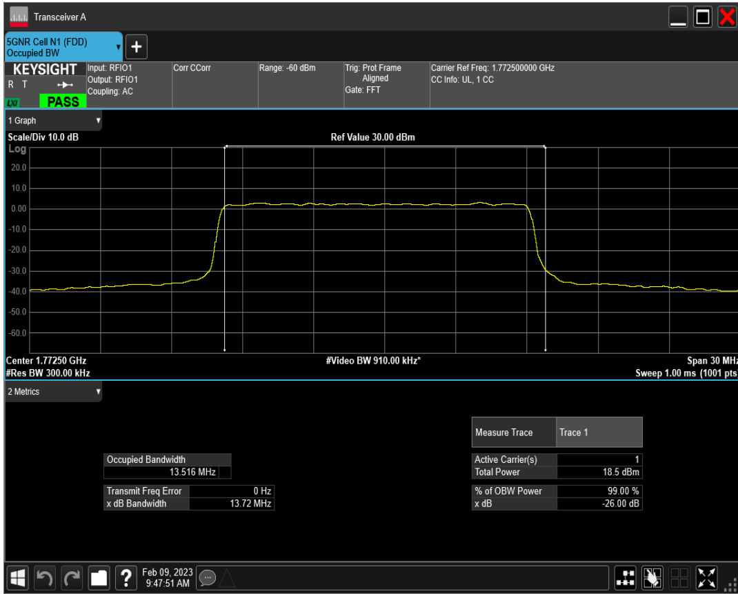
n66 SCS=30kHz CP_QPSK BW=15MHz Channel=354500 RB=38@0
