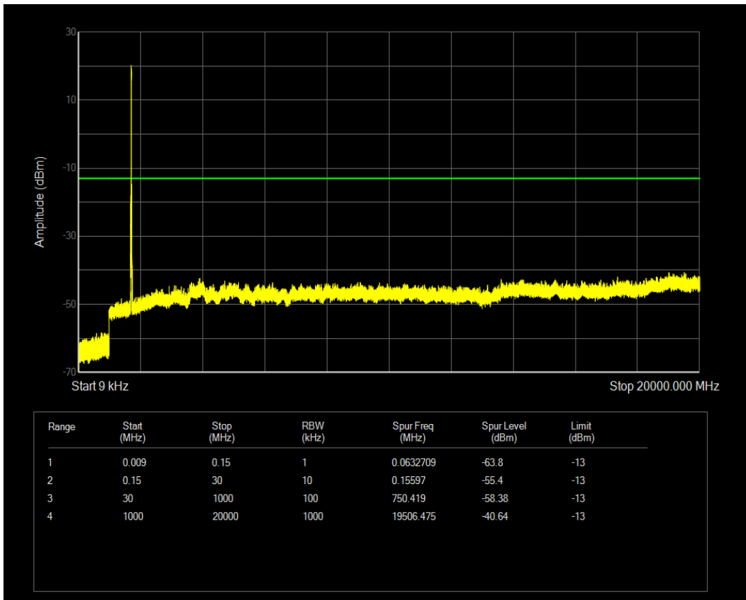
n66 SCS=30kHz DFT_QPSK BW=10MHz Channel=343000 RB=1@0
