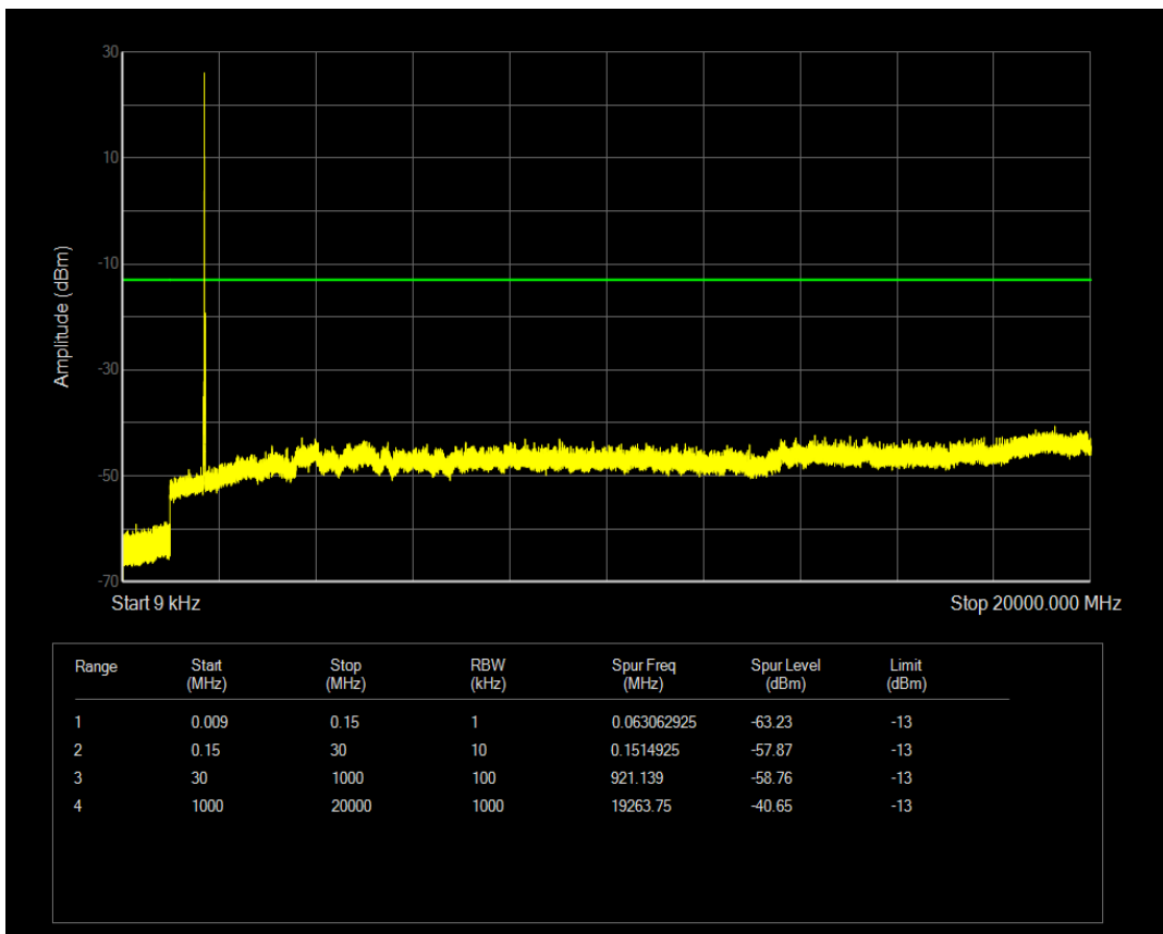
n66 SCS=30kHz DFT_QPSK BW=10MHz Channel=343000 RB=1@23
