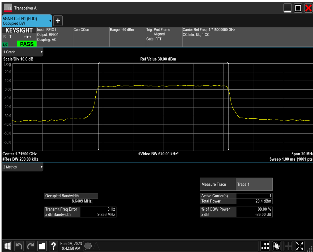
n66 SCS=30kHz DFT_QAM256 BW=10MHz Channel=343000 RB=24@0
