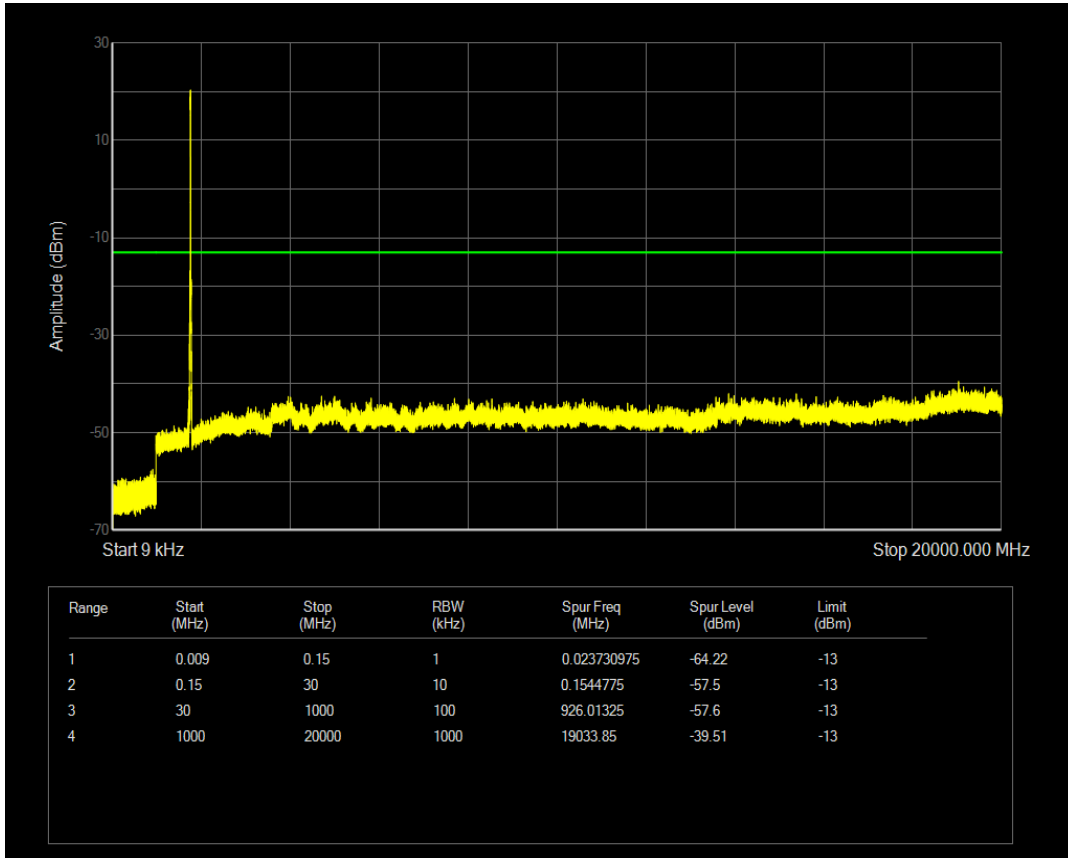
n66 SCS=30kHz DFT_QPSK BW=10MHz Channel=355000 RB=1@0
