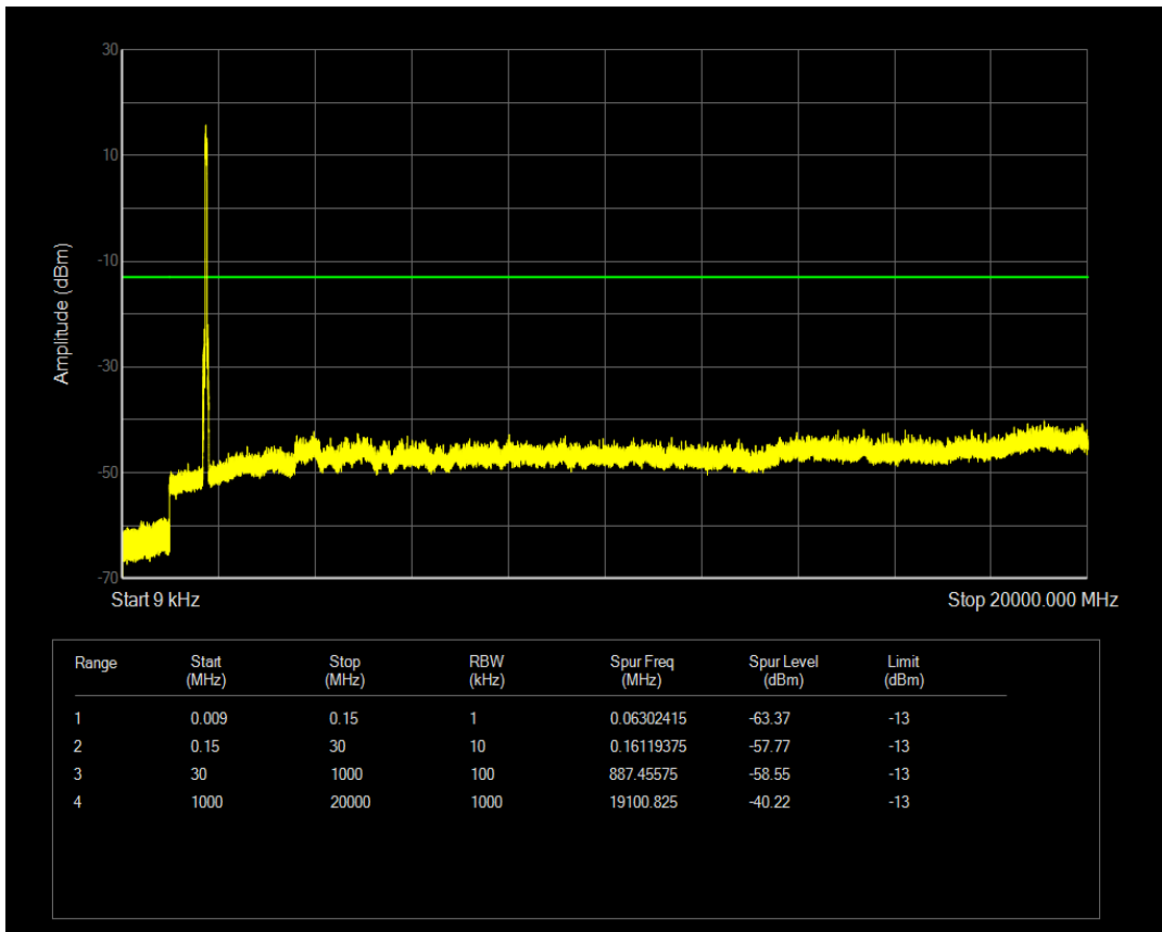
n66 SCS=30kHz DFT_QPSK BW=40MHz Channel=352000 RB=1@0
