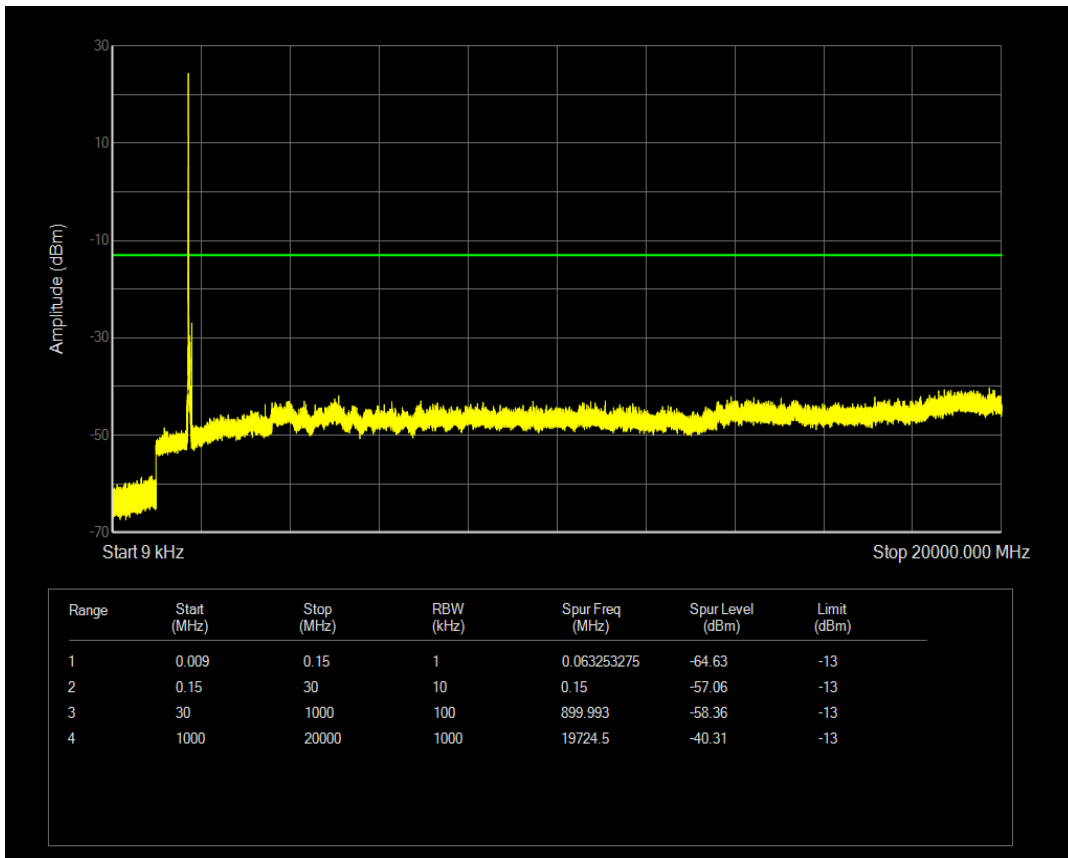
n66 SCS=15kHz DFT_QPSK BW=40MHz Channel=349000 RB=1@215
