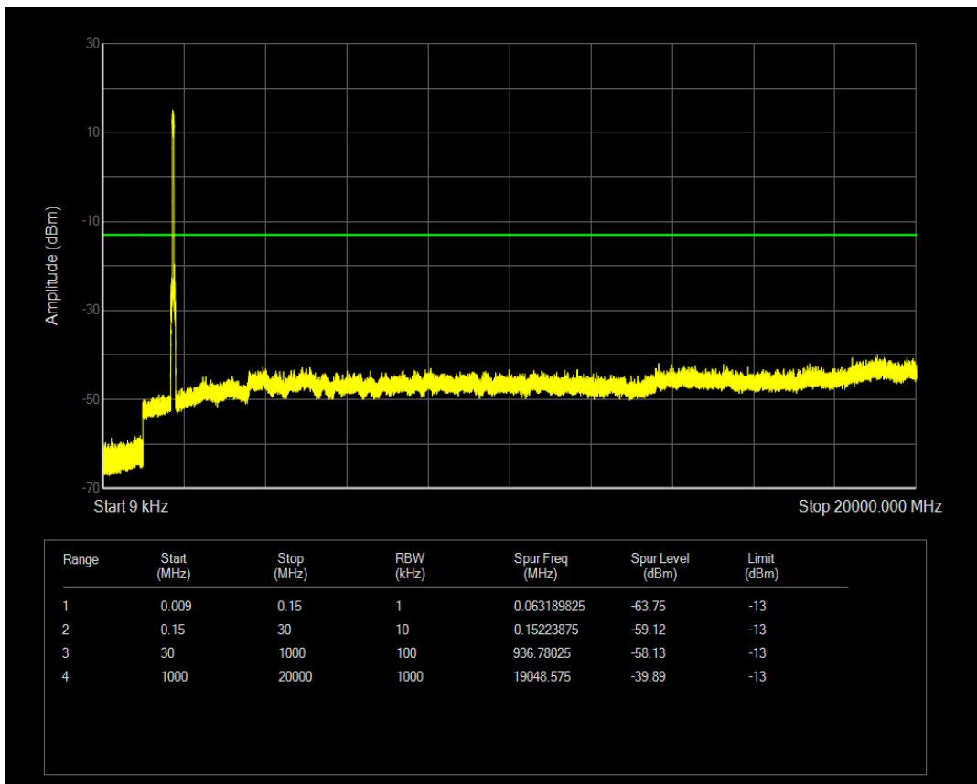
n66 SCS=15kHz DFT_QPSK BW=40MHz Channel=346000 RB=1@215
