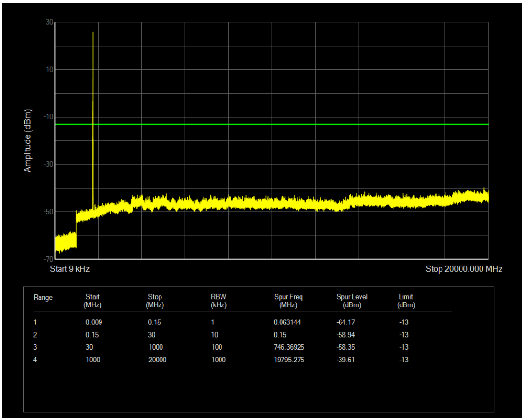
n66 SCS=15kHz DFT_QPSK BW=5MHz Channel=355500 RB=1@24
