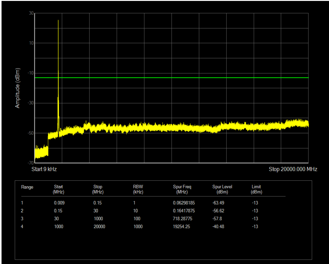
n66 SCS=15kHz DFT_QPSK BW=40MHz Channel=352000 RB=1@215
