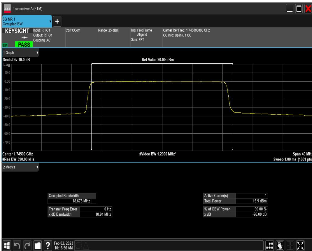
n66 SCS=15kHz CP_QPSK BW=20MHz Channel=349000 RB=106@0
