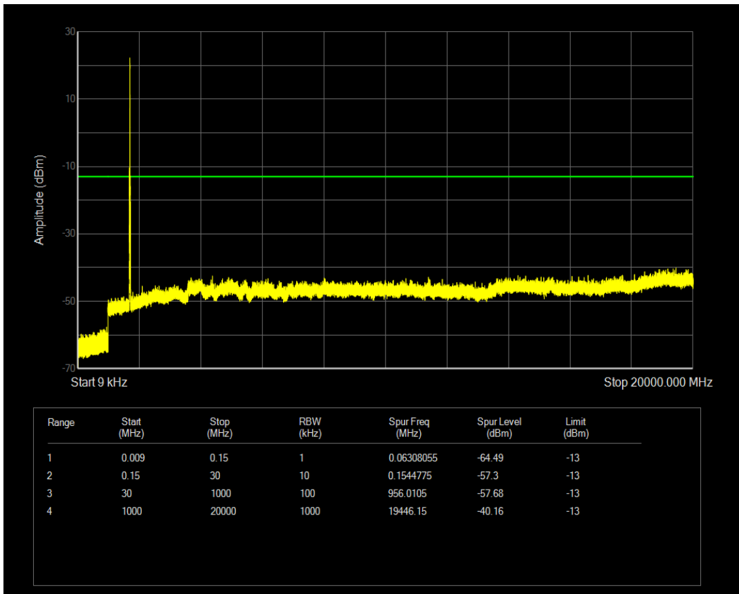
n66 SCS=15kHz DFT_QPSK BW=5MHz Channel=342500 RB=1@0
