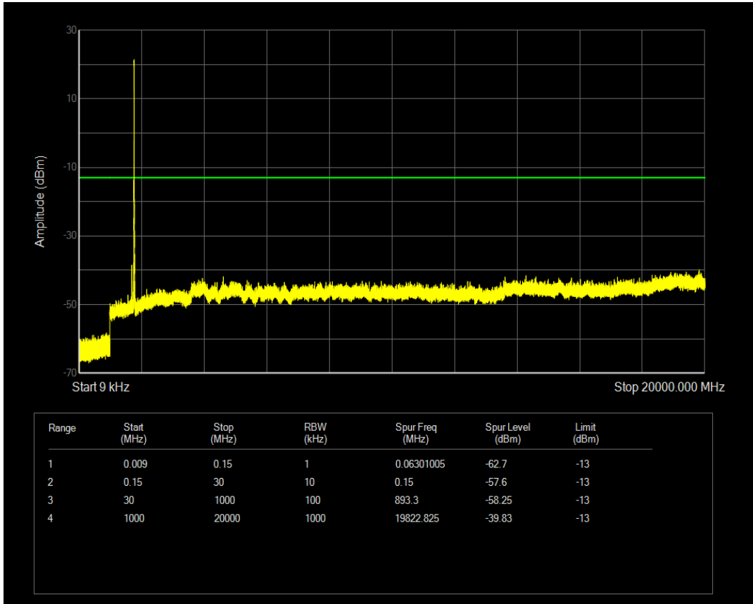
n66 SCS=15kHz DFT_QPSK BW=5MHz Channel=355500 RB=1@0
