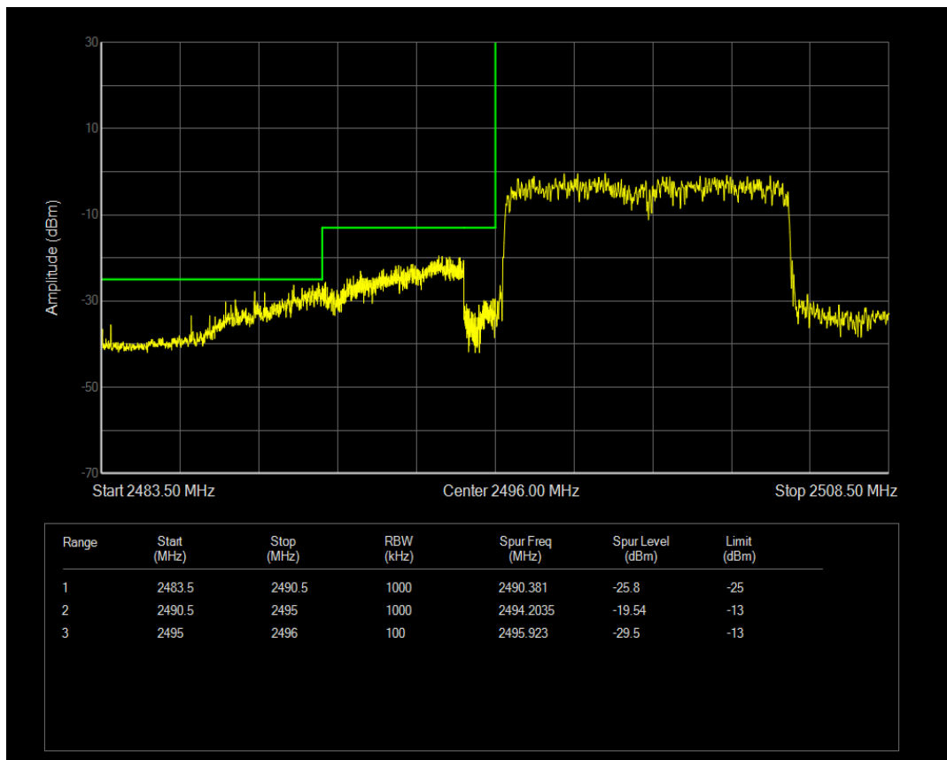
n41 SCS=15kHz DFT_QPSK BW=10MHz Channel=500202 RB=1@0
