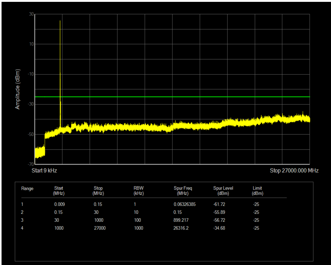
n41 SCS=15kHz DFT_QPSK BW=10MHz Channel=500202 RB=1@51
