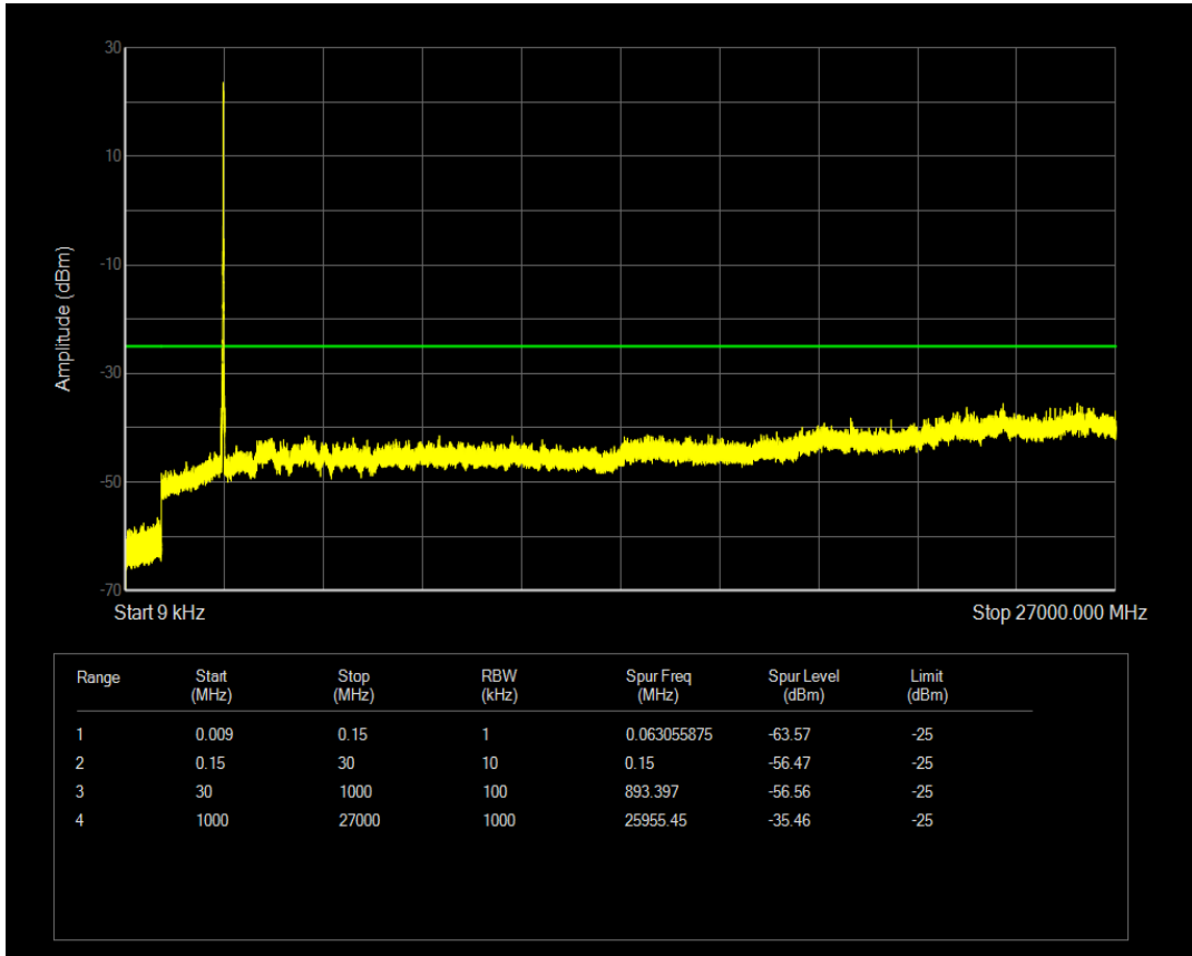
n41 SCS=15kHz DFT_QPSK BW=10MHz Channel=537000 RB=1@0
