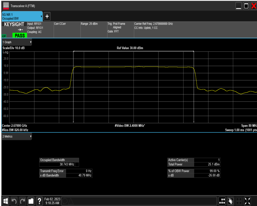
n41 SCS=15kHz DFT_QPSK BW=40MHz Channel=534000 RB=216@0
