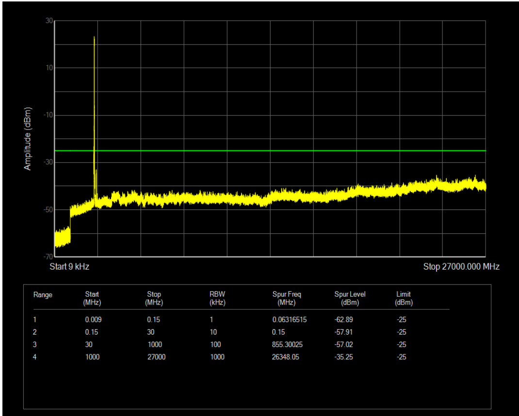
n41 SCS=15kHz DFT_QPSK BW=10MHz Channel=500202 RB=1@0
