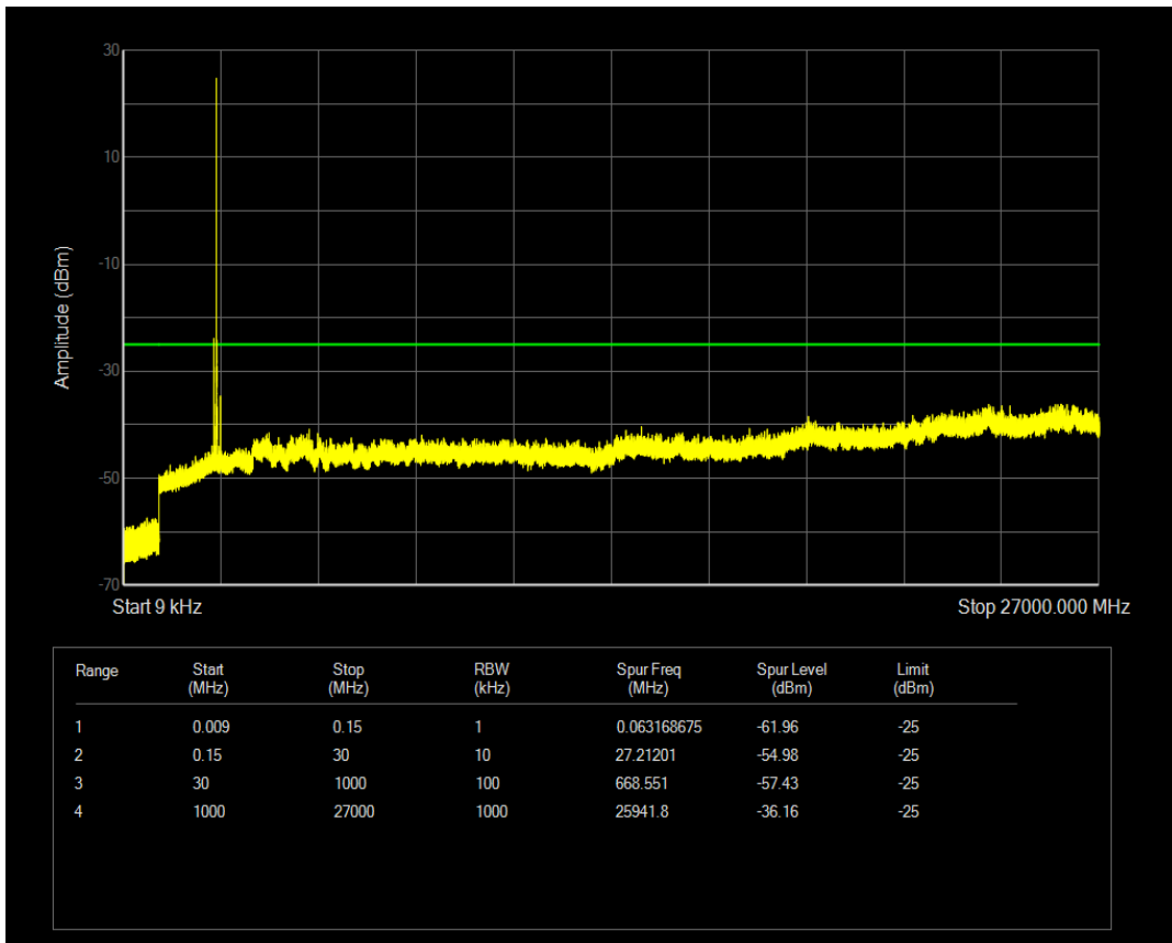
n41 SCS=15kHz DFT_QPSK BW=10MHz Channel=518601 RB=1@51
