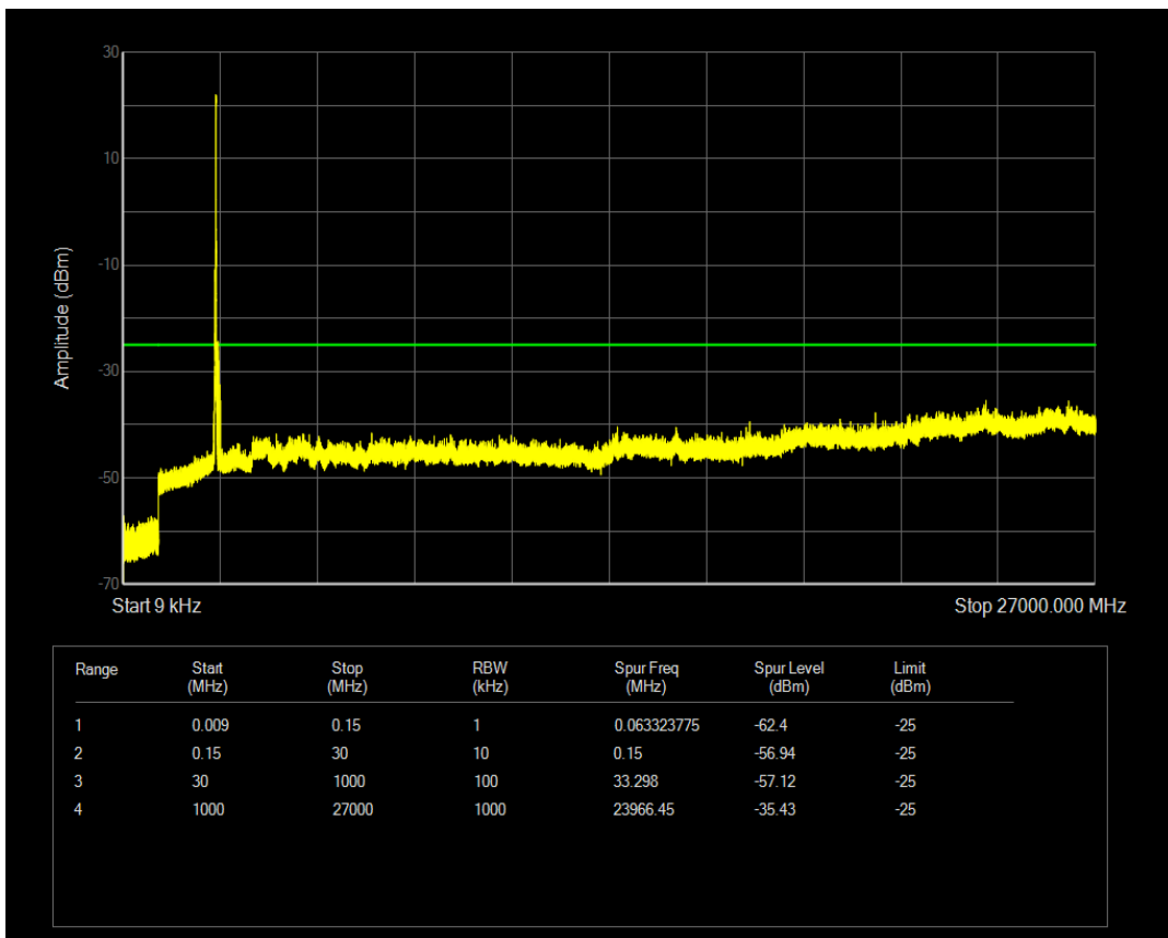
n41 SCS=15kHz DFT_QPSK BW=10MHz Channel=518601 RB=1@0
