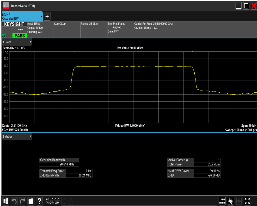
n41 SCS=15kHz DFT_QPSK BW=30MHz Channel=502200 RB=160@0
