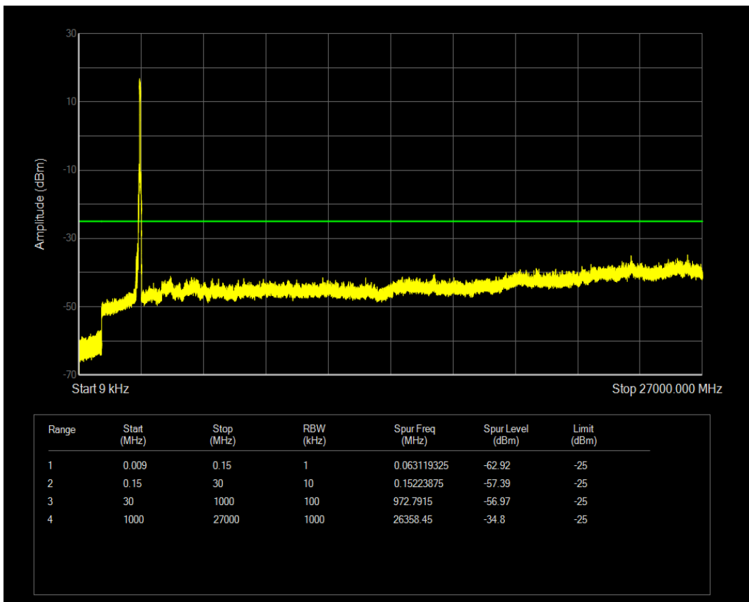
n41 SCS=15kHz DFT_QPSK BW=50MHz Channel=532998 RB=1@0
