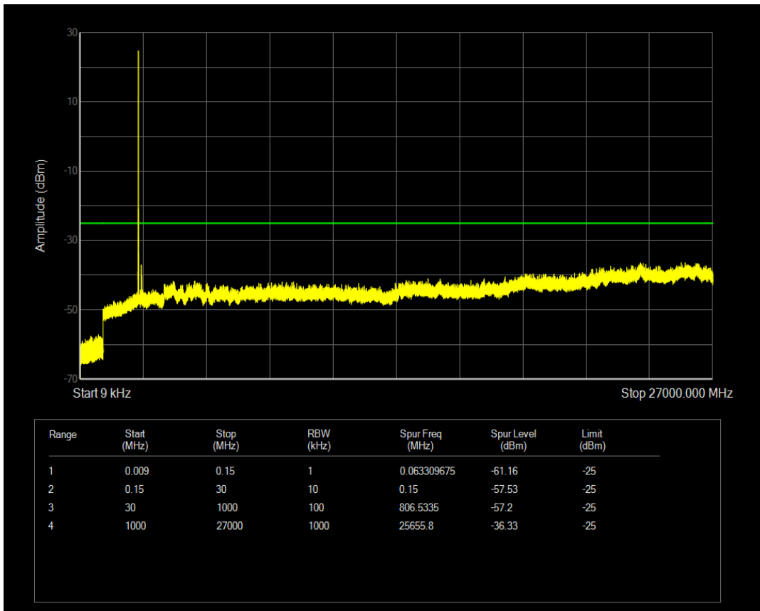
n41 SCS=15kHz DFT_QPSK BW=10MHz Channel=518601 RB=50@0
