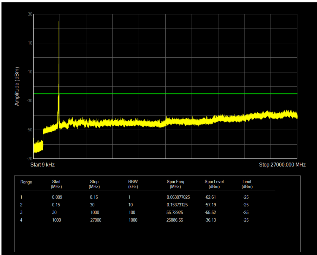
n41 SCS=15kHz DFT_QPSK BW=50MHz Channel=518601 RB=1@0
