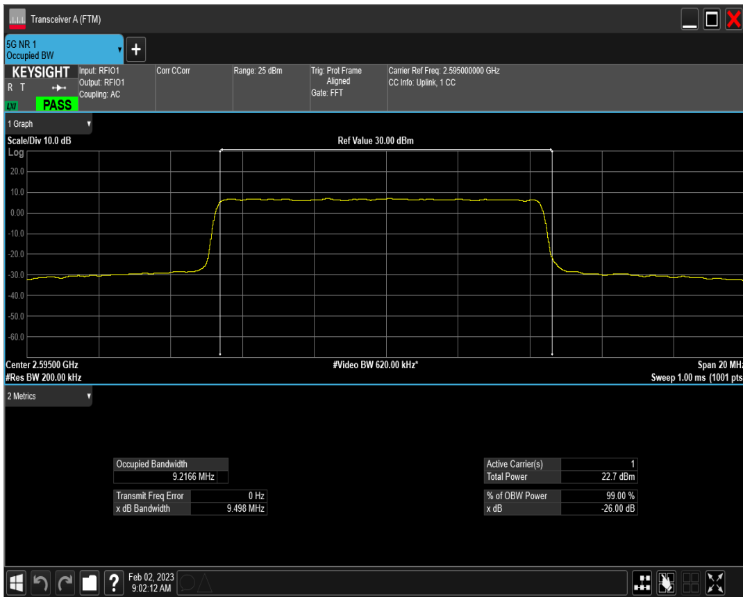
n38 SCS=15kHz DFT_QAM16 BW=10MHz Channel=519000 RB=50@0
