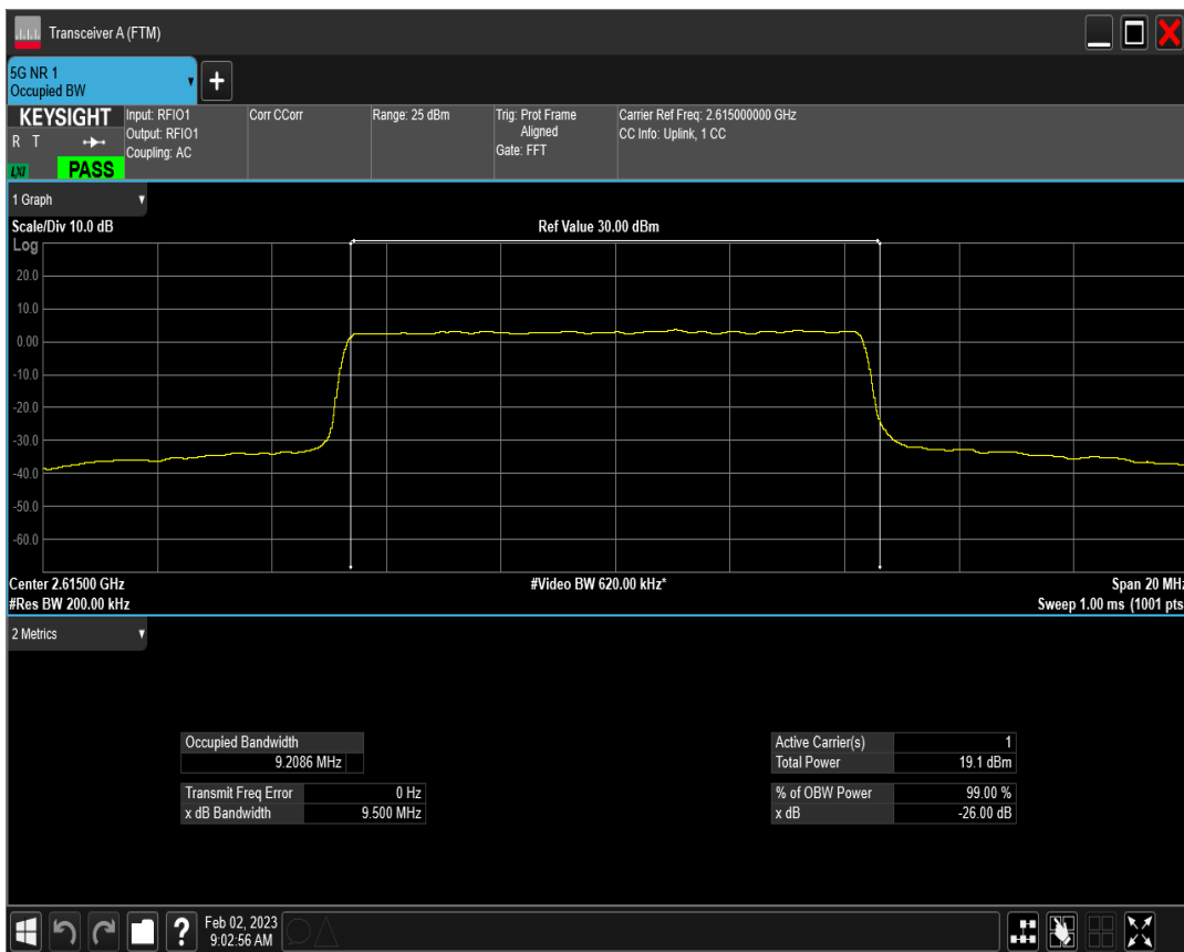
n38 SCS=15kHz CP_QPSK BW=10MHz Channel=523000 RB=52@0
