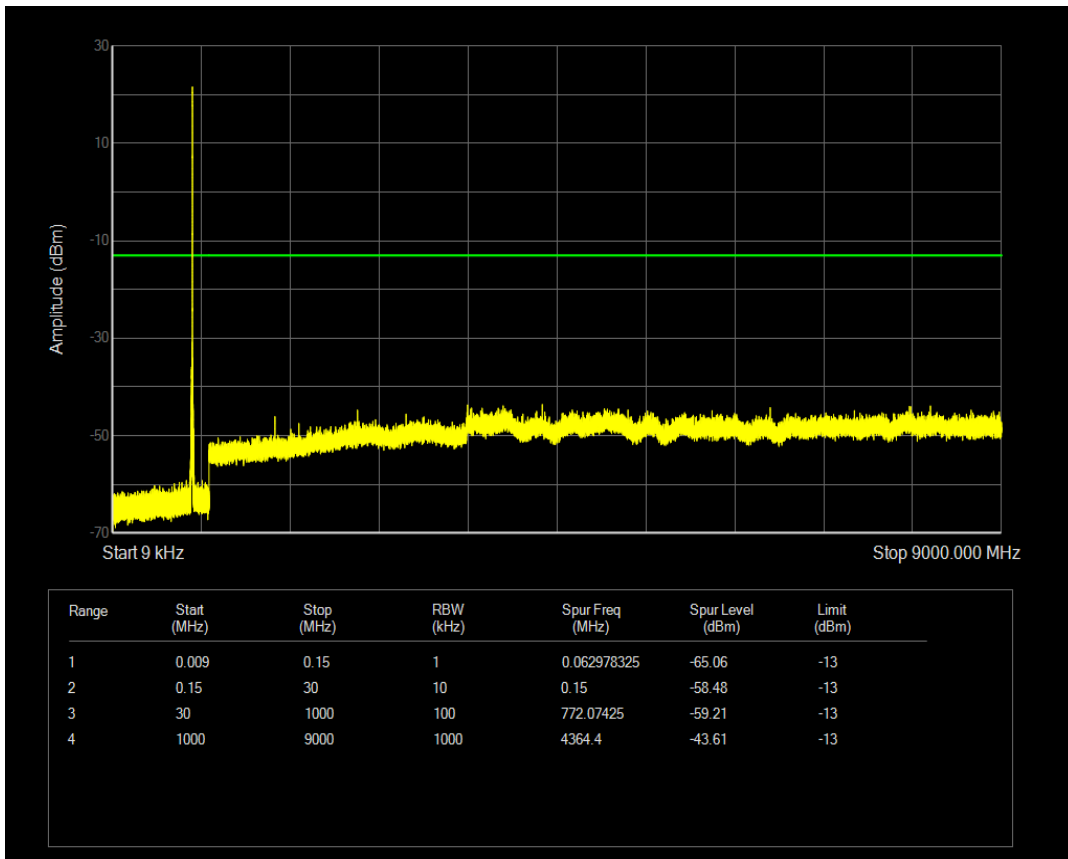
n5 SCS=30kHz DFT_QPSK BW=10MHz Channel=167300 RB=24@0
