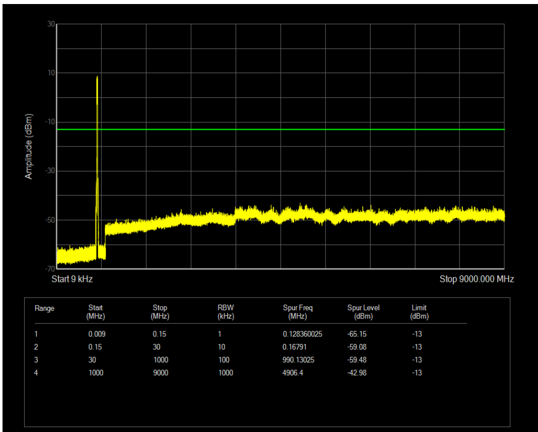
n5 SCS=30kHz DFT_QPSK BW=20MHz Channel=167800 RB=1@0
