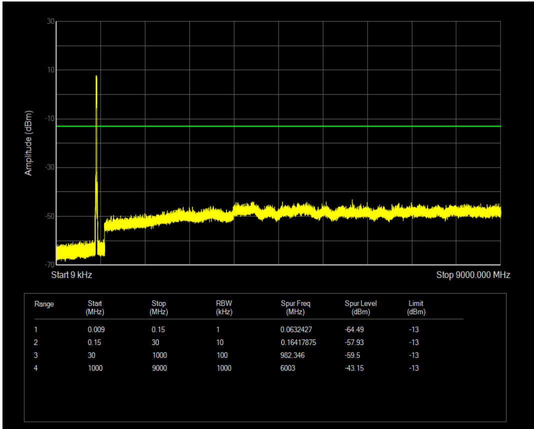
n5 SCS=30kHz DFT_QPSK BW=20MHz Channel=167300 RB=1@0
