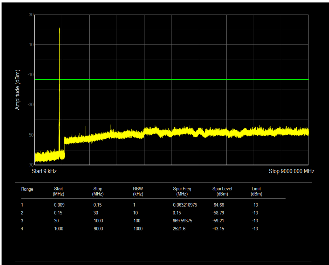
n5 SCS=30kHz DFT_QPSK BW=10MHz Channel=168800 RB=24@0
