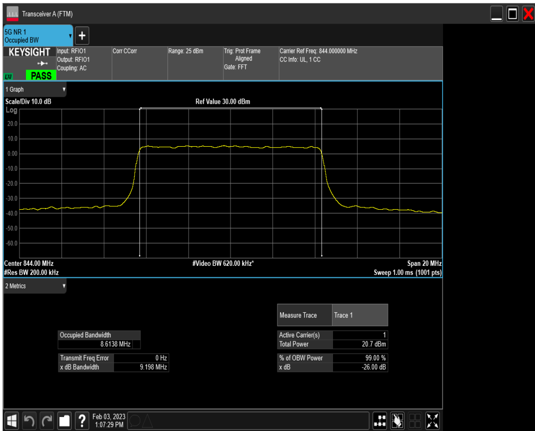
n5 SCS=30kHz DFT_QAM256 BW=10MHz Channel=168800 RB=24@0
