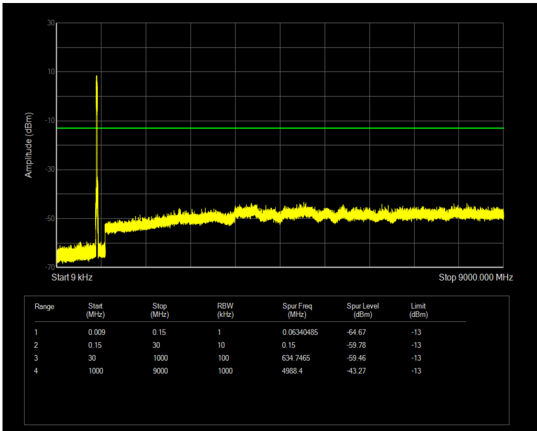
n5 SCS=30kHz DFT_QPSK BW=20MHz Channel=166800 RB=1@0
