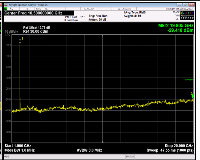
Band2-20MHz-16QAM-19100-1RB#0-Range2:1000~20000MHz
