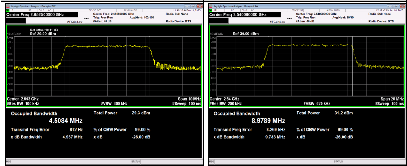
Band41-10MHz-QPSK-40640-50RB#0
