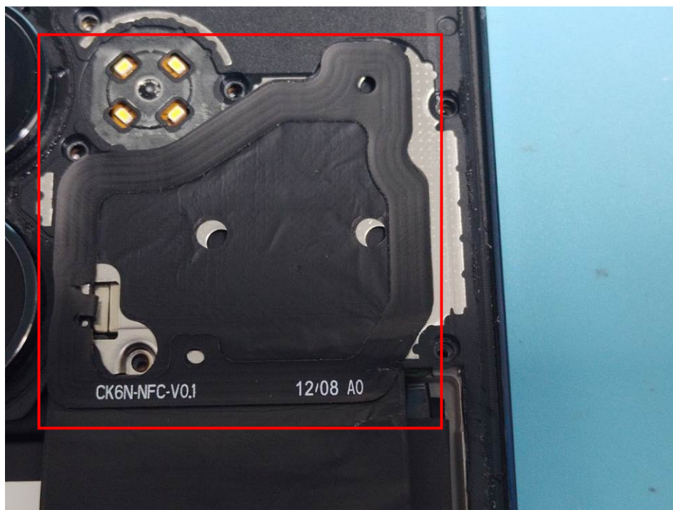
NFC Antenna
