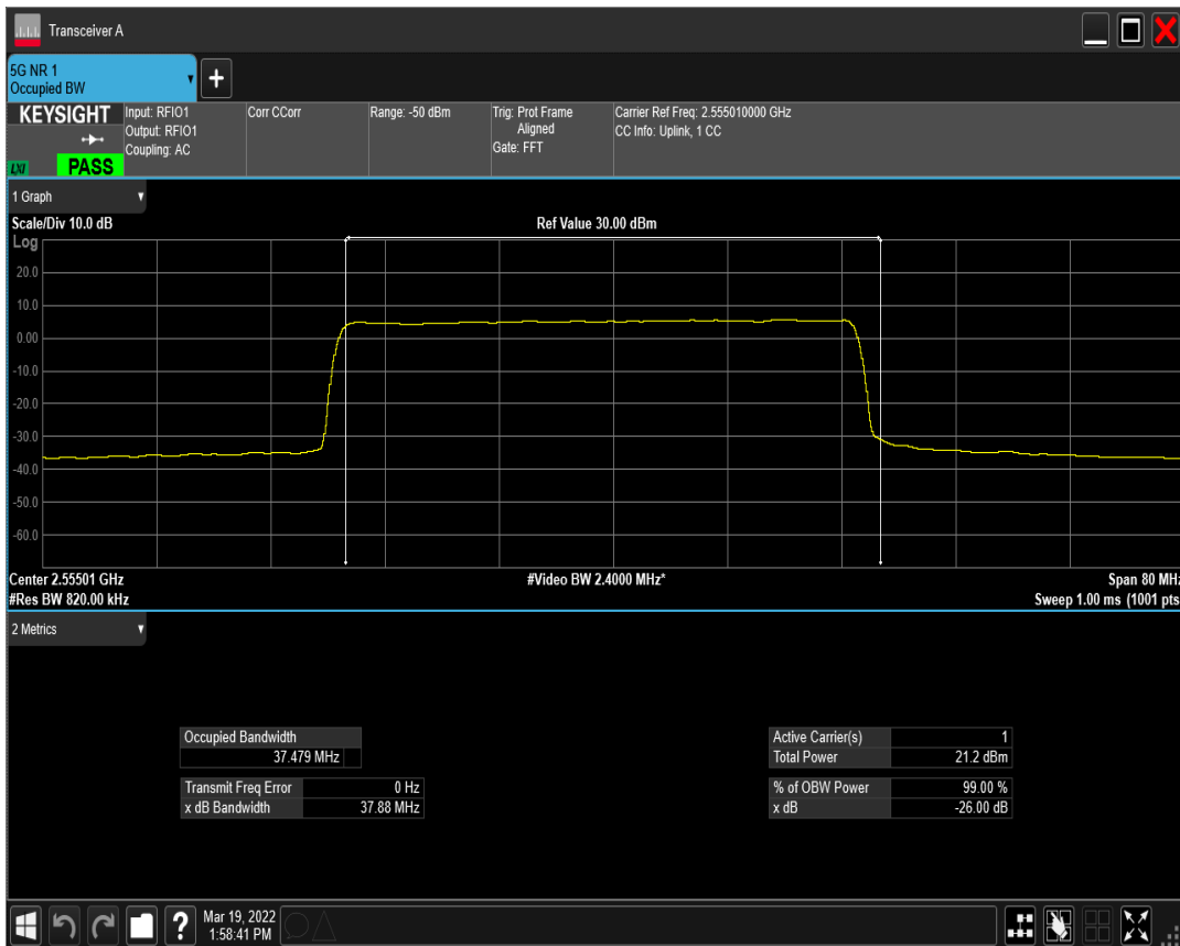
n41(2535-2655) SCS=30kHz CP_QPSK BW=40MHz Channel=511002 RB=106@0
