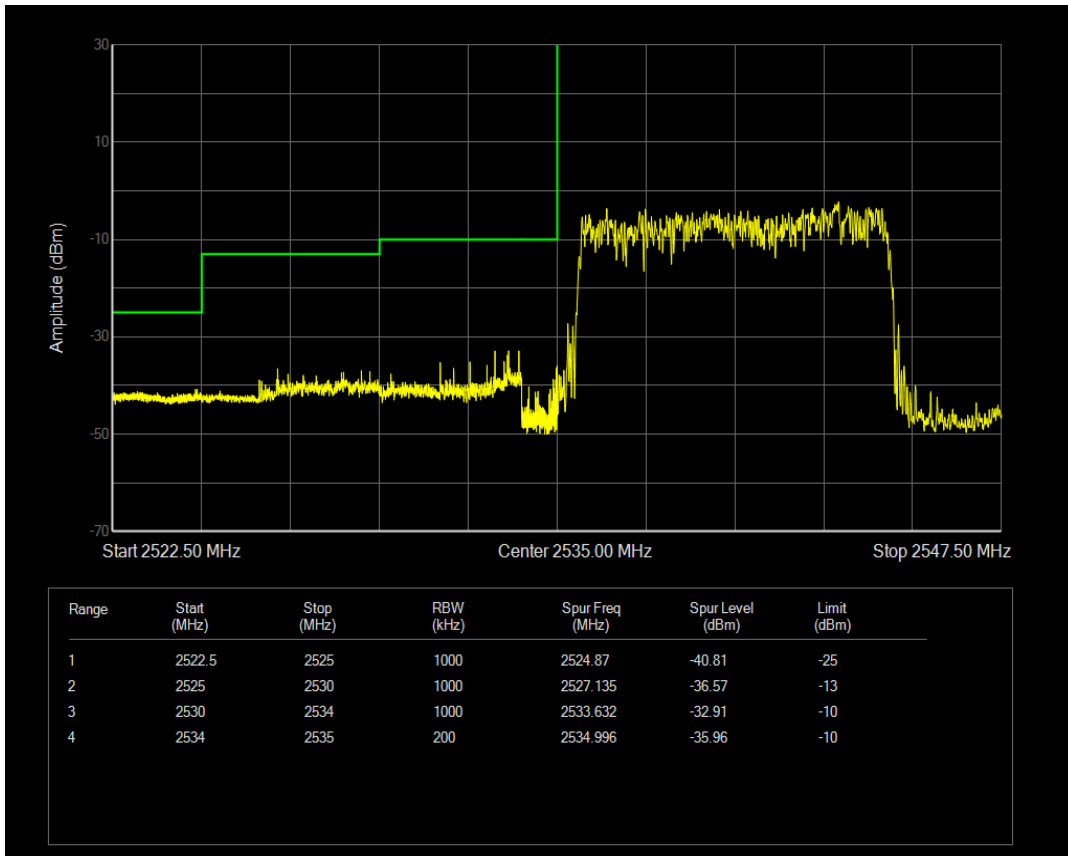
n41(2535-2655) SCS=30kHz DFT_QPSK BW=10MHz Channel=508002 RB=1@0
