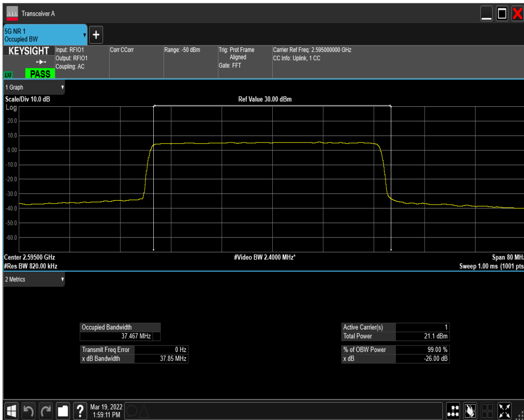
n41(2535-2655) SCS=30kHz CP_QPSK BW=40MHz Channel=519000 RB=106@0
