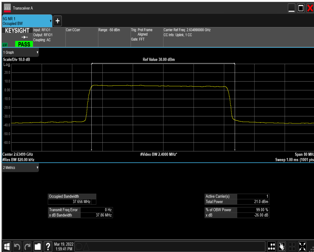
n41(2535-2655) SCS=30kHz CP_QPSK BW=40MHz Channel=526998 RB=106@0
