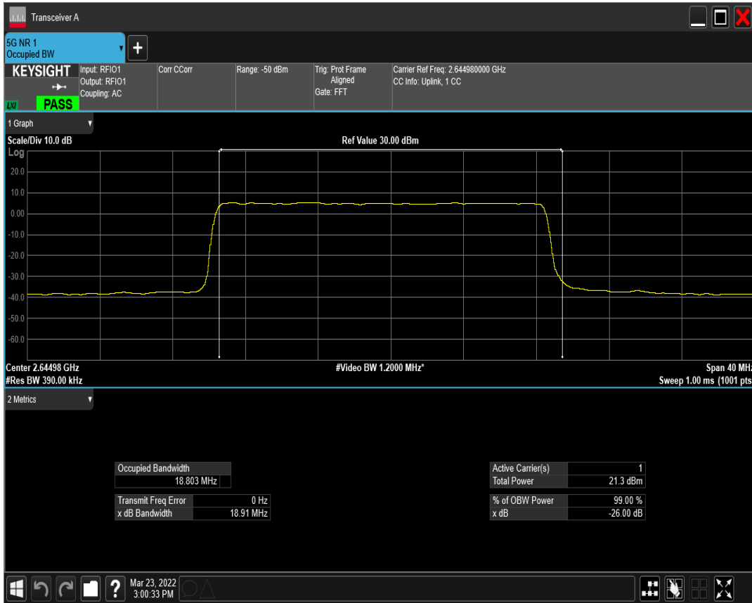
n41(2535-2655) SCS=15kHz CP_QPSK BW=20MHz Channel=528996 RB=106@0
