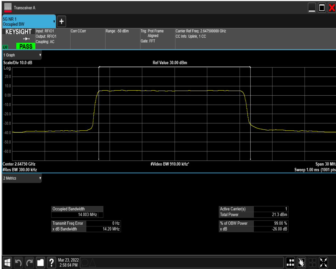
n41(2535-2655) SCS=15kHz CP_QPSK BW=15MHz Channel=529500 RB=79@0
