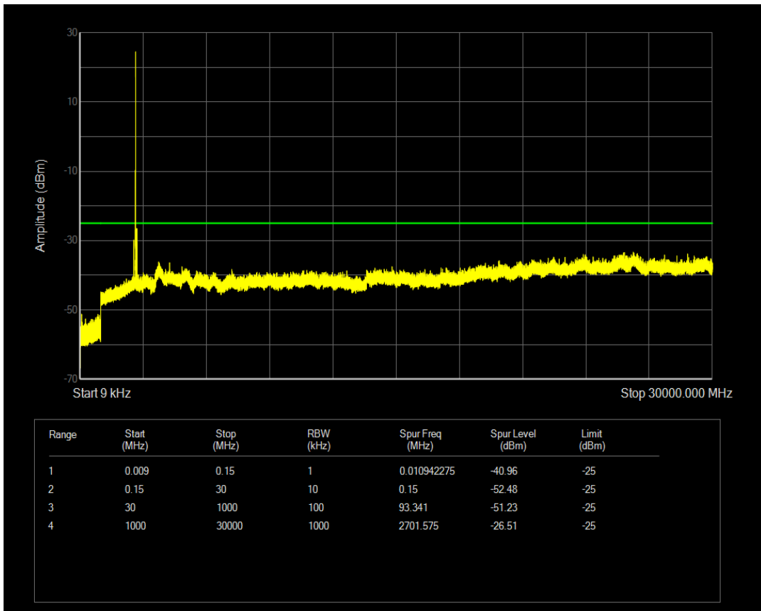
n41(2535-2655) SCS=15kHz DFT_QPSK BW=50MHz Channel=512004 RB=1@0
