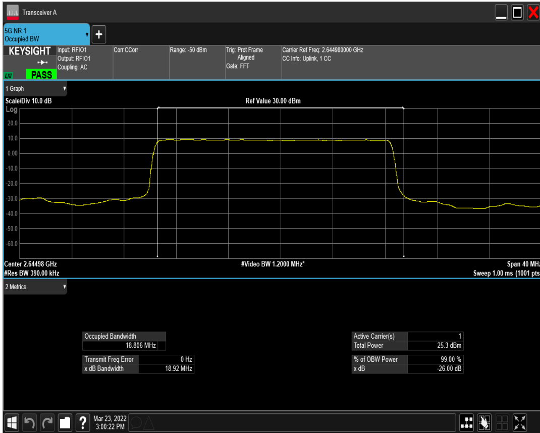
n41(2535-2655) SCS=15kHz DFT_QPSK BW=20MHz Channel=528996 RB=100@0
