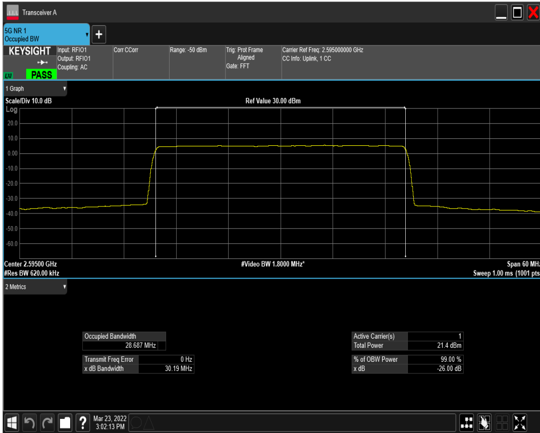
n41(2535-2655) SCS=15kHz CP_QPSK BW=30MHz Channel=519000 RB=160@0
