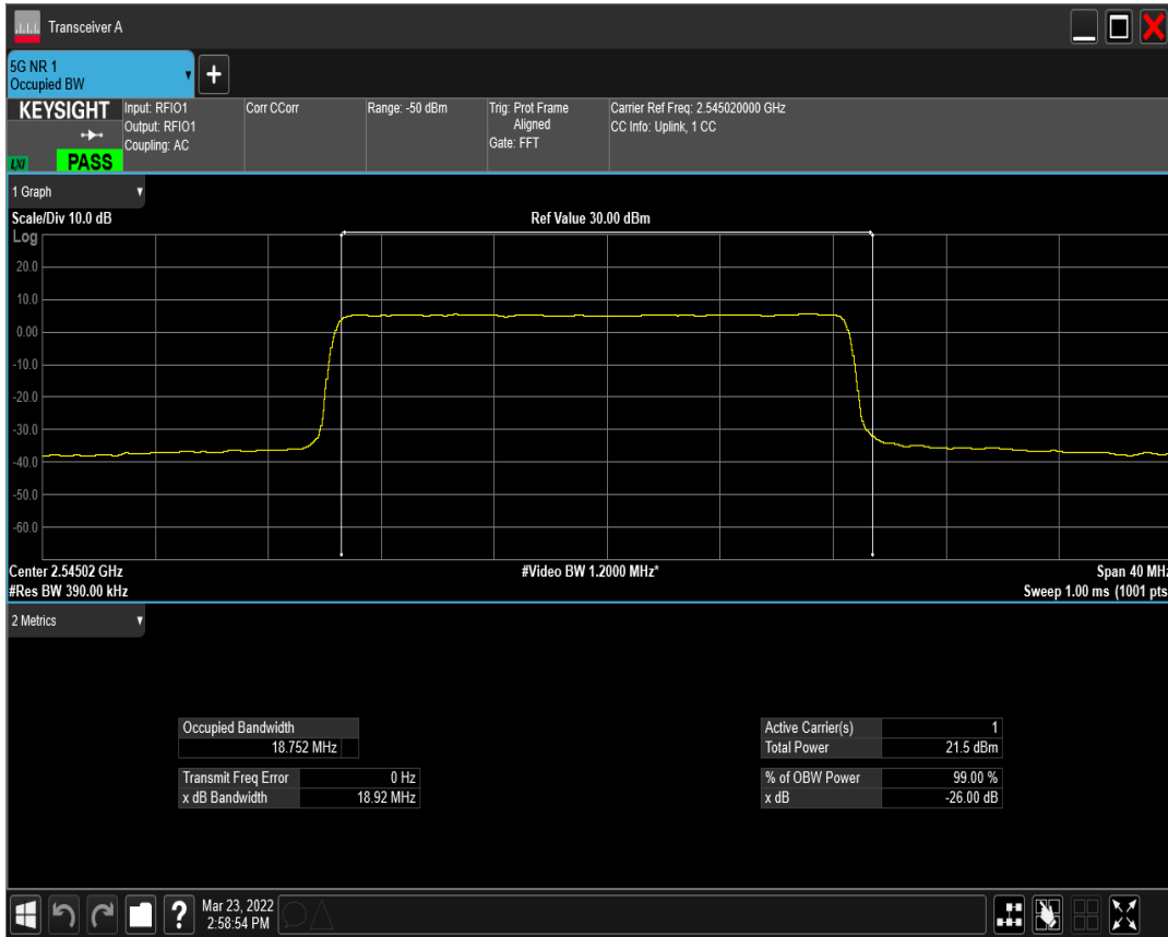
n41(2535-2655) SCS=15kHz CP_QPSK BW=20MHz Channel=509004 RB=106@0
