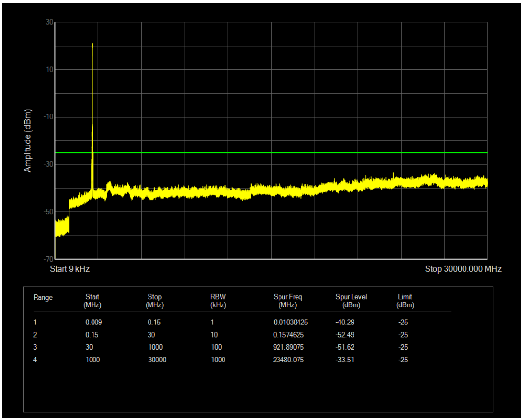
n41(2535-2655) SCS=15kHz DFT_QPSK BW=10MHz Channel=519000 RB=1@0
