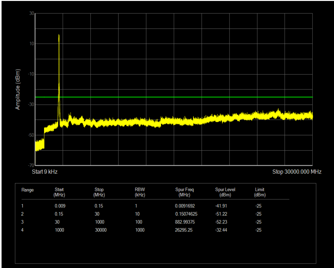
n41(2535-2655) SCS=15kHz DFT_QPSK BW=50MHz Channel=519000 RB=1@0
