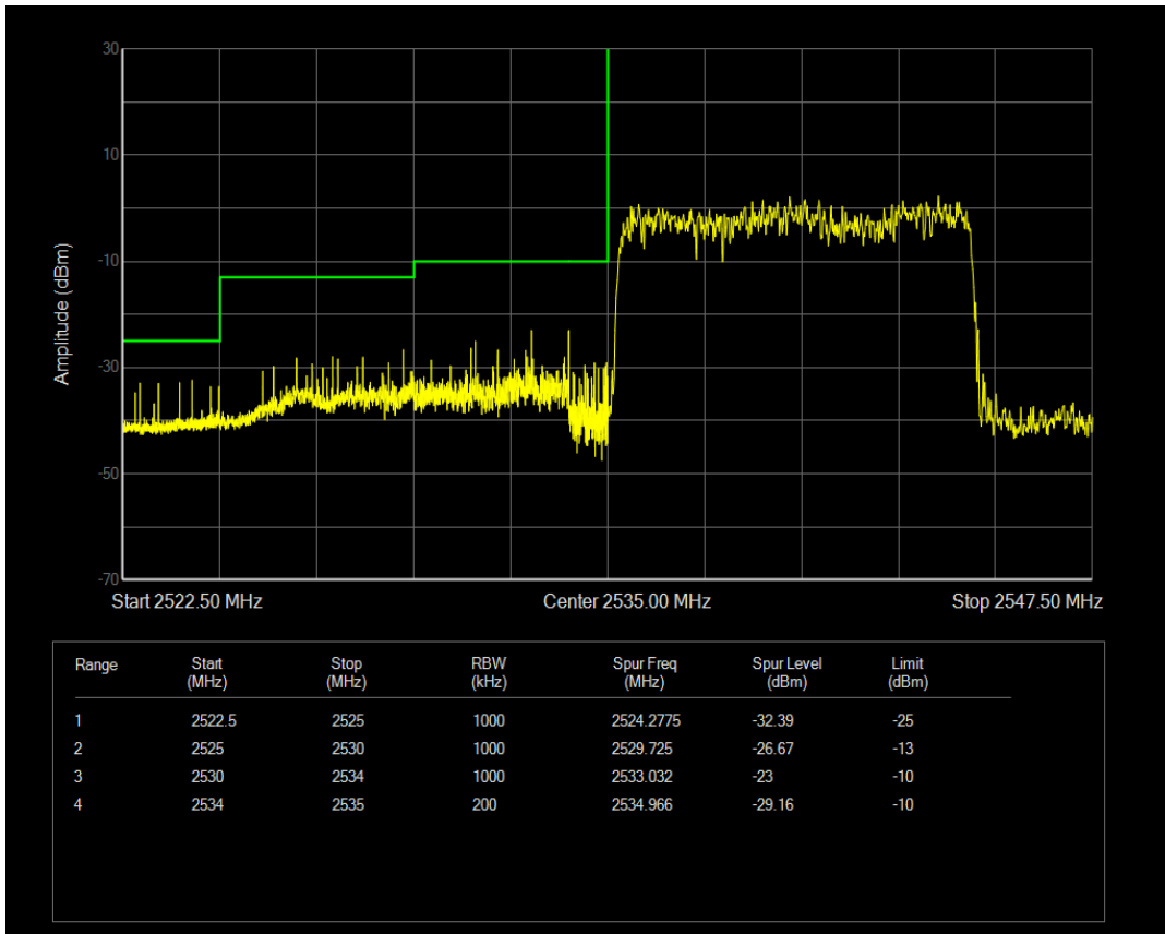
n41(2535-2655) SCS=15kHz DFT_QPSK BW=10MHz Channel=508002 RB=1@0
