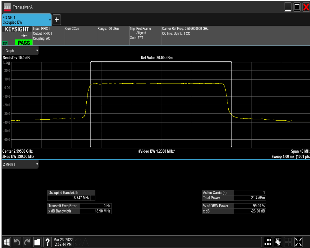
n41(2535-2655) SCS=15kHz CP_QPSK BW=20MHz Channel=519000 RB=106@0
