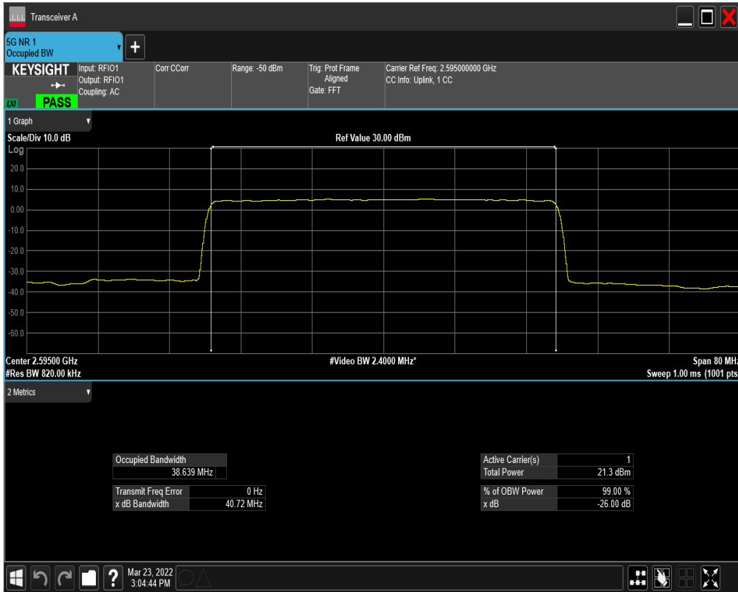
n41(2535-2655) SCS=15kHz CP_QPSK BW=40MHz Channel=519000 RB=216@0
