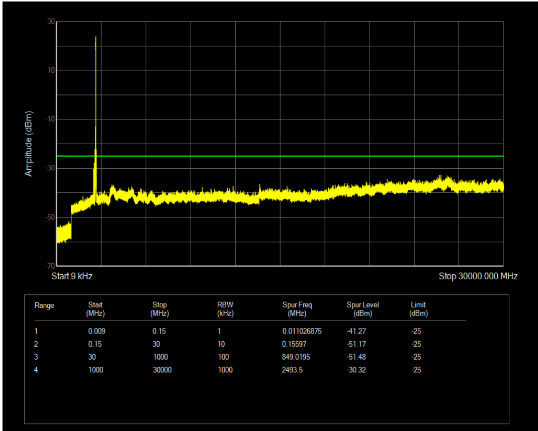
n41(2535-2655) SCS=15kHz DFT_QPSK BW=10MHz Channel=529998 RB=1 @0
