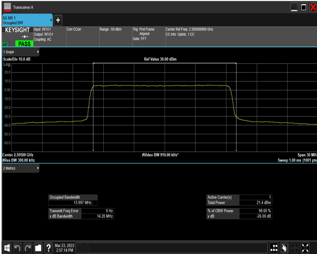
n41(2535-2655) SCS=15kHz CP_QPSK BW=15MHz Channel=519000 RB=79@0
