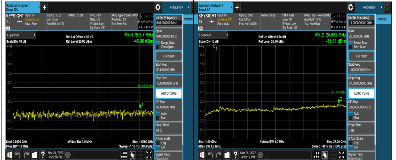
Band41-5MHz-16QAM-40065-1RB#0-Range1:30~ 1000MHz Band41-5MHz-16QAM-40065-1RB#0-Range2:1000~2 7000MHz
