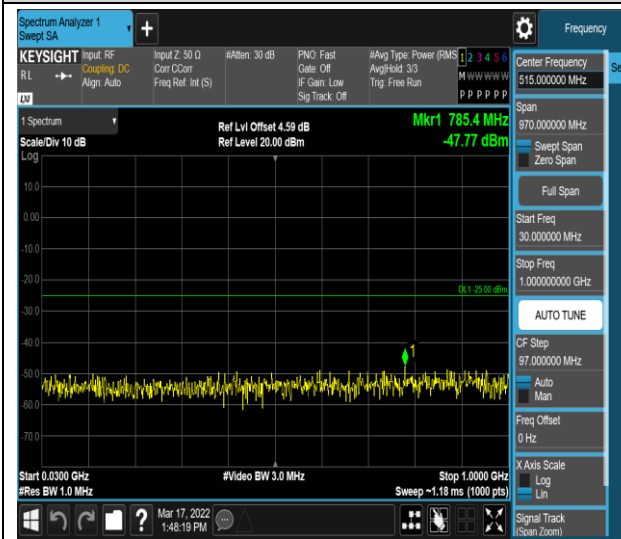
Band41-5MHz-QPSK-40065-1RB#0-Range1:30~1000MHz
