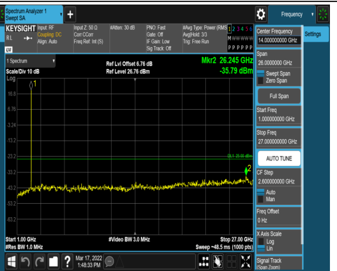
Band41-5MHz-QPSK-40065-1RB#0-Range2:1000~27000MHz
