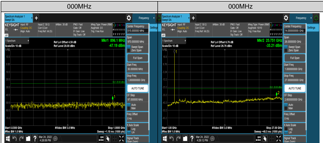
Band41-5MHz-QPSK-41215-1RB#0-Range1:30~1 000MHz Band41-5MHz-QPSK-41215-1RB#0-Range2:1000~27 000MHz
