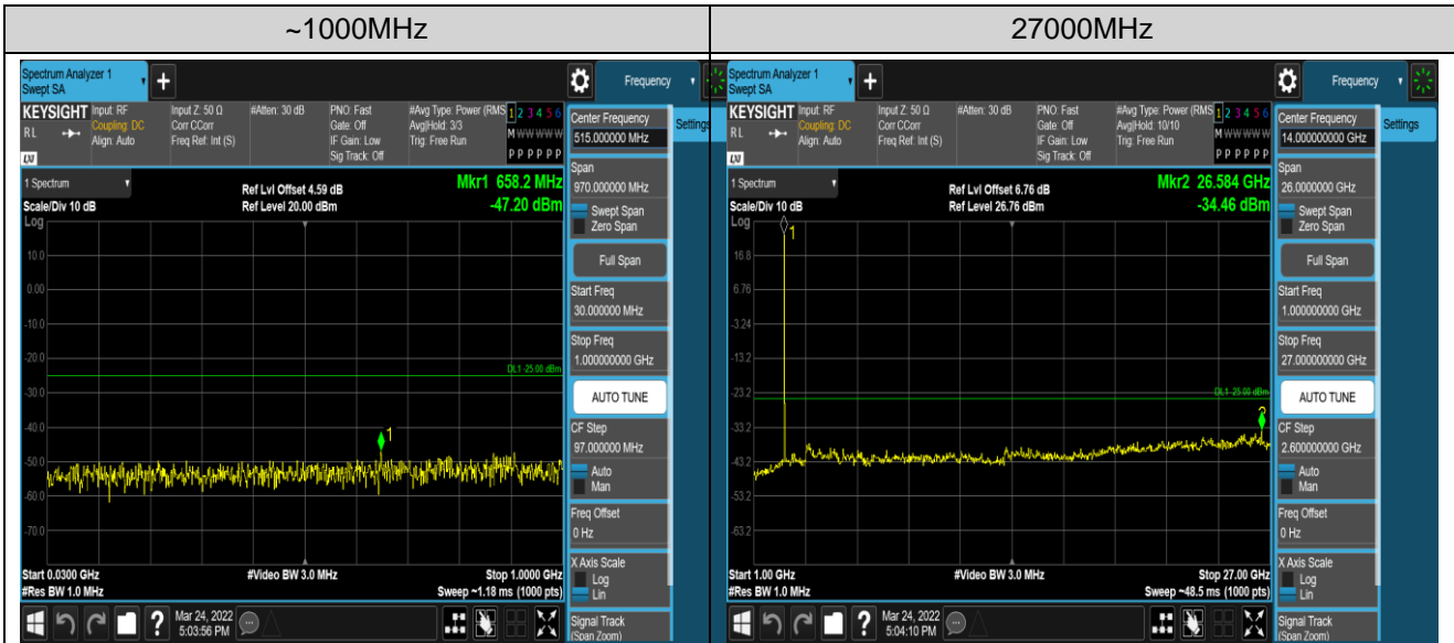
Band41-20MHz-16QAM-40640-1RB#0-Range1:30 ~1000MHz Band41-20MHz-16QAM-40640-1RB#0-Range2:1000~ 27000MHz
