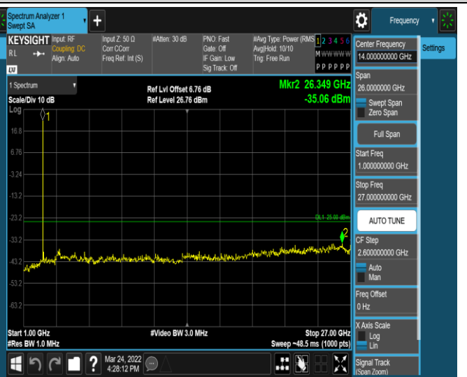
Band41-5MHz-QPSK-40640-1RB#0-Range2:1000~27000MHz
