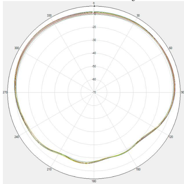
2.4G WIFI&BT \Theta=90^\circ
