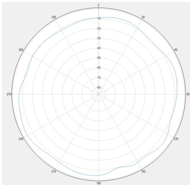
GPS \Phi=90^\circ
