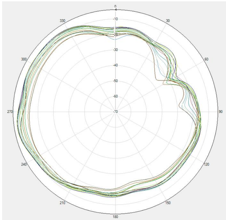
5G WIFI Theta=90deg
