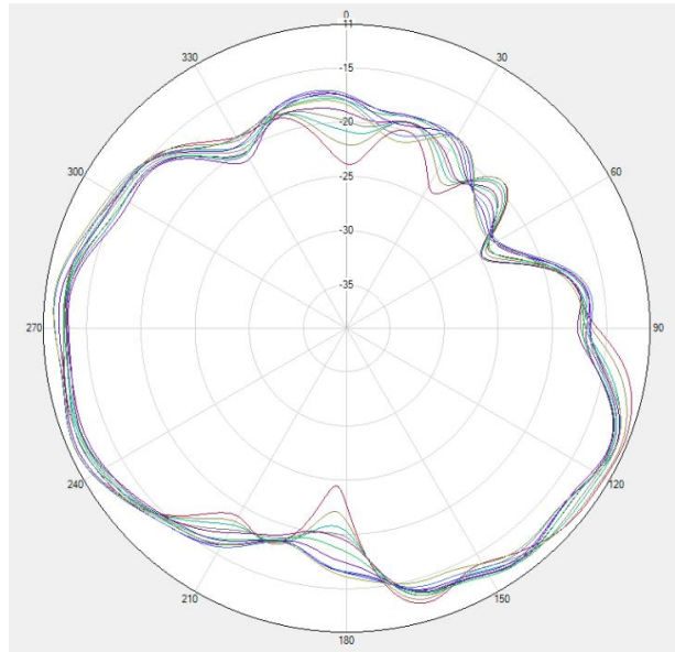
GSM850 / WCDMA B5 / LTE B5/B20 Phi=90deg
