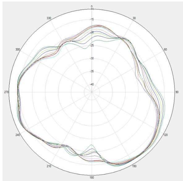
GSM850 / WCDMA B5 / LTE B5/B20 Phi=0deg
