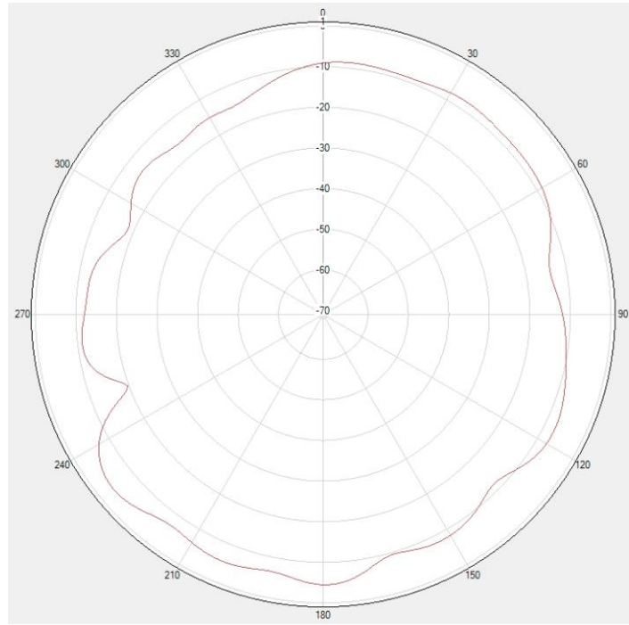
GPS \Phi=0^\circ
