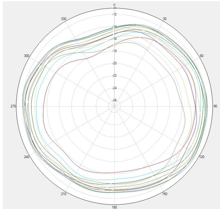
LTE B28 Theta=90deg
