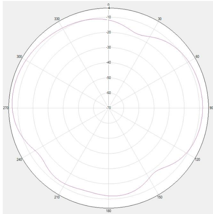
GPS \Theta = 90^\circ
