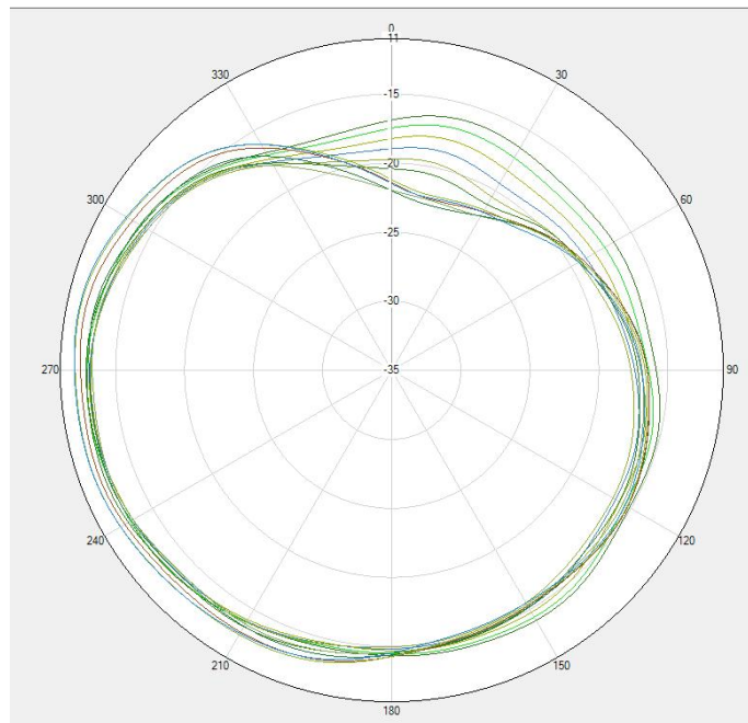
GSM850 / WCDMA B5 / LTE B5/B20 Theta=90deg
