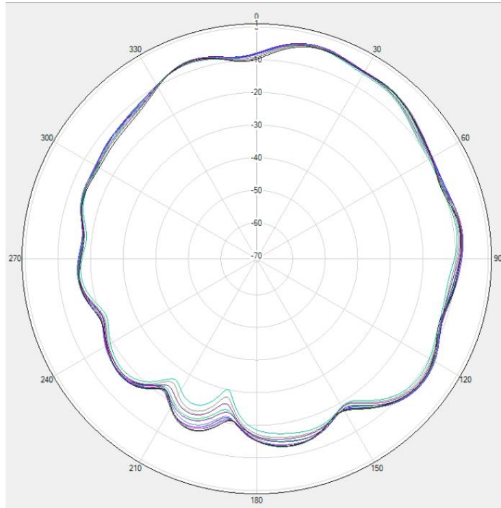
2.4G WIFI&BT \Phi=90^\circ
