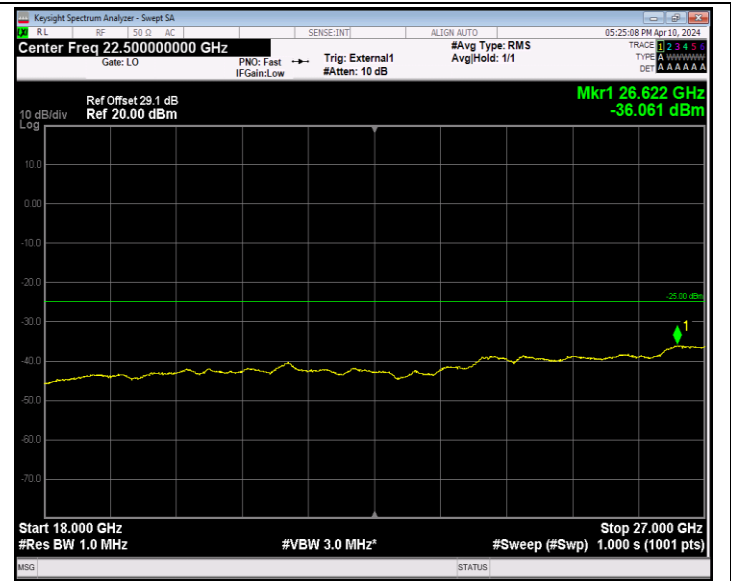
Band41_5MHz_64QAM_40620_1RB#0_18000~27000_18000~27 000
