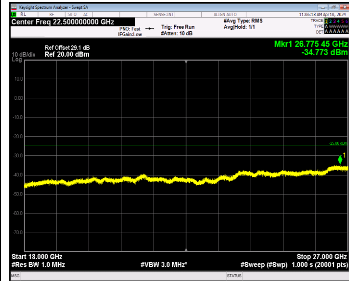
Band7_20MHz_16QAM_20850_1RB#0_18000~27000_18000~27 000
