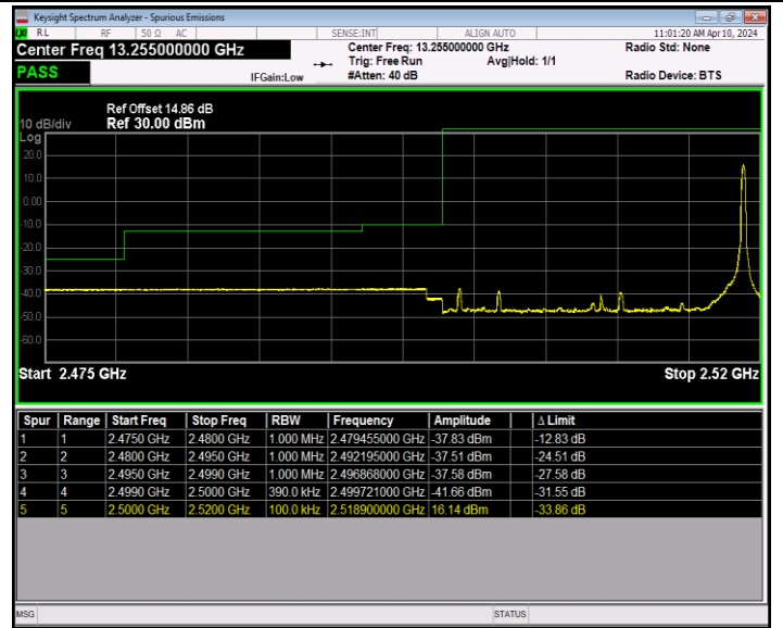
Band7_20MHz_QPSK_20850_1RB#99
