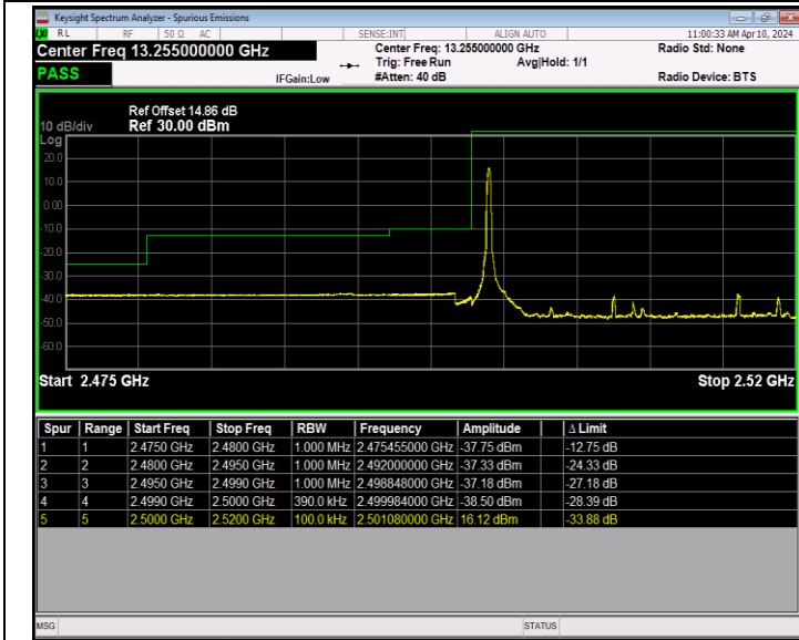
Band7_20MHz_QPSK_20850_1RB#0
