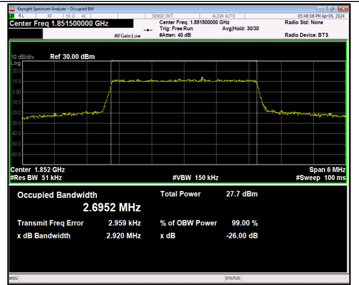
Band2-3MHz-QPSK-18615-15RB#0-PASS
