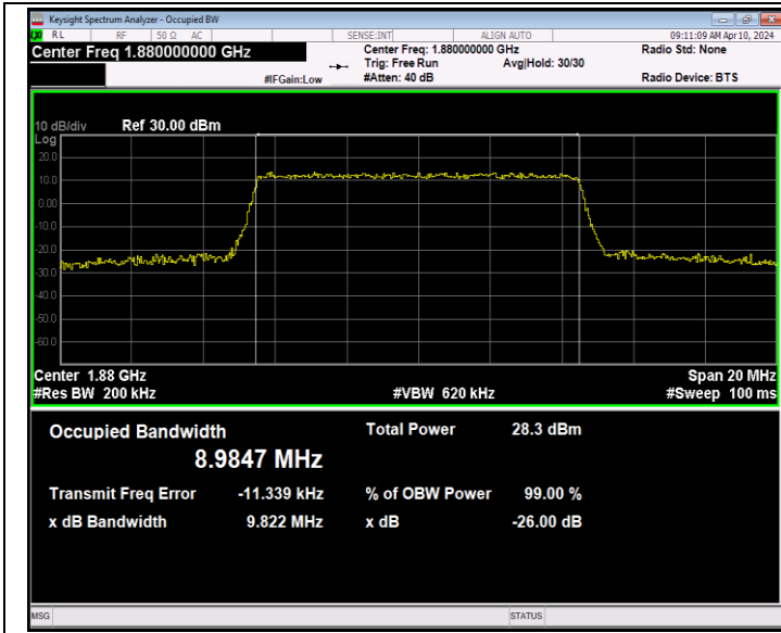
Band2-10MHz-QPSK-18900-50RB#0-PASS
