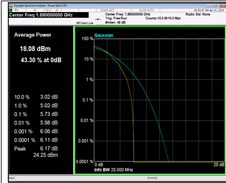
Band2-20MHz-64QAM-18900-1RB#0-PASS
