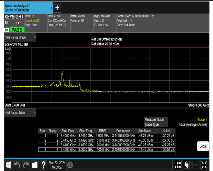
Band42_20MHz_QPSK_42190_1RB#0
