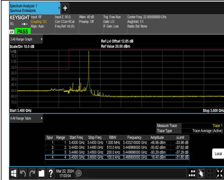
Band42_20MHz_QPSK_42190_1RB#99
