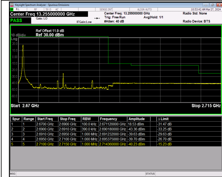
Band41_20MHz_QPSK_41490_1RB#0
