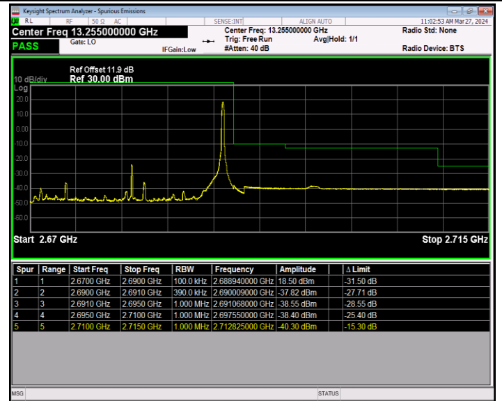
Band41_20MHz_QPSK_41490_1RB#99
