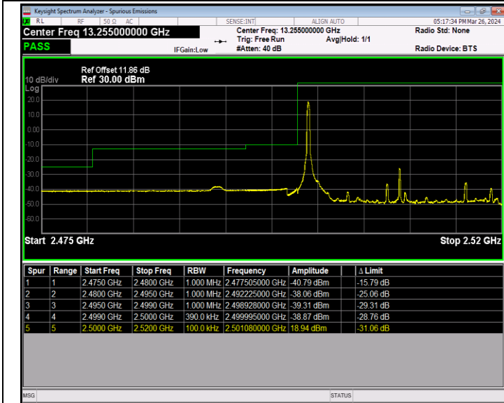
Band7_20MHz_QPSK_20850_1RB#0
