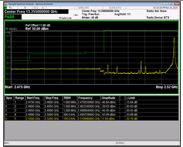
Band7_20MHz_16QAM_20850_1RB#99
