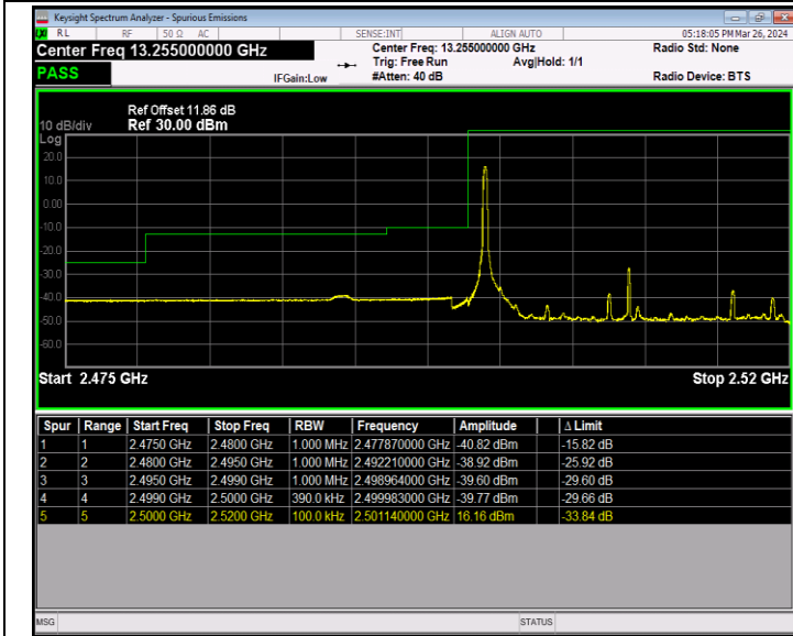
Band7_20MHz_64QAM_20850_1RB#0
