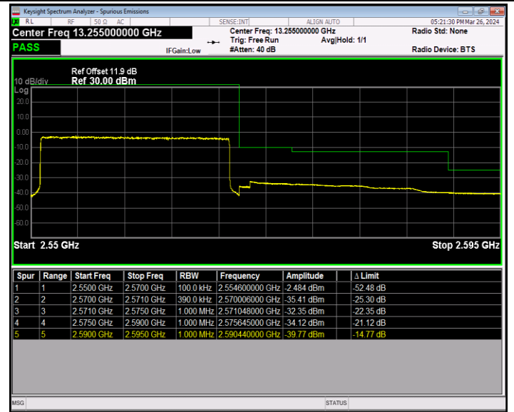
Band7_20MHz_QPSK_21350_100RB#0
