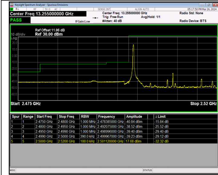
Band7_20MHz_16QAM_20850_1RB#0
