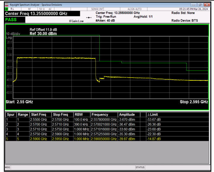
Band7_20MHz_16QAM_21350_100RB#0
