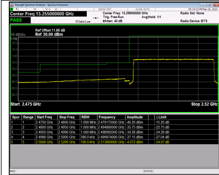
Band7_20MHz_16QAM_20850_100RB#0
