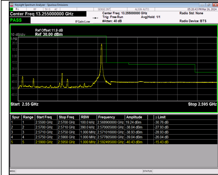
Band7_20MHz_QPSK_21350_1RB#99
