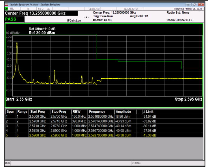
Band7_20MHz_QPSK_21350_1RB#0
