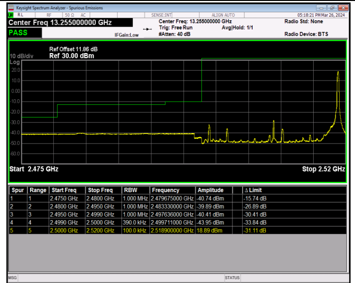
Band7_20MHz_QPSK_20850_1RB#99
