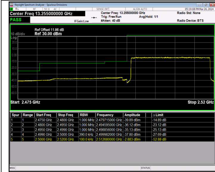
Band7_20MHz_QPSK_20850_100RB#0
