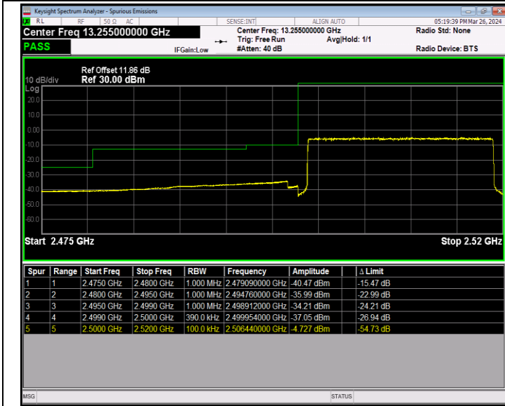
Band7_20MHz_64QAM_20850_100RB#0
