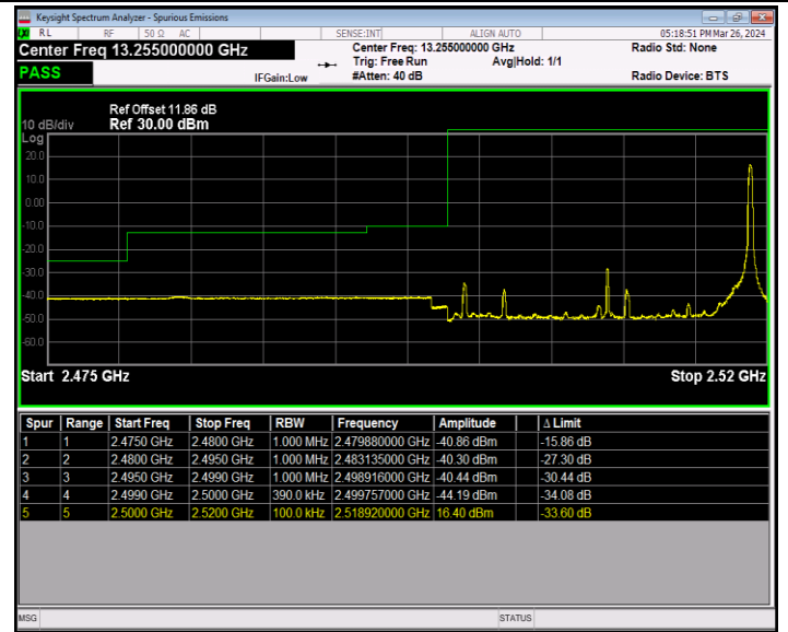
Band7_20MHz_64QAM_20850_1RB#99
