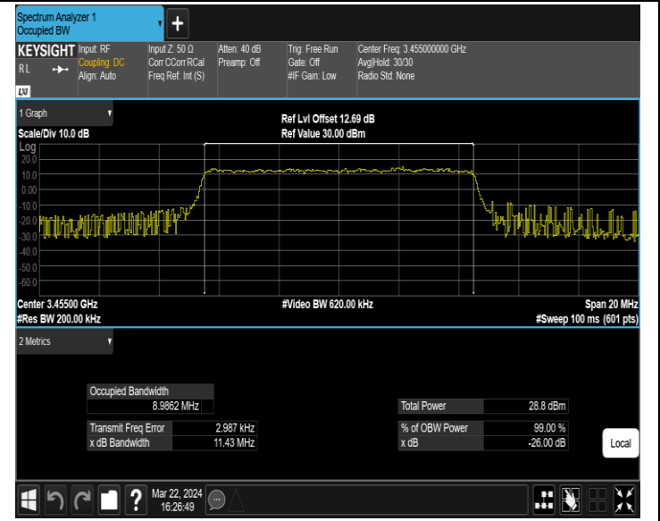
42(3450-3550)-10MHz-64QAM-42140-50RB#0-PASS
