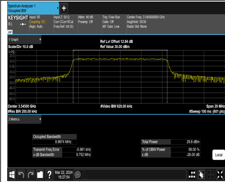
42(3450-3550)-10MHz-16QAM-43040-50RB#0-PASS
