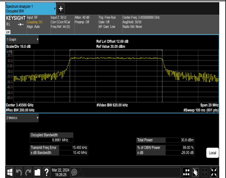
42(3450-3550)-10MHz-QPSK-42140-50RB#0-PASS
