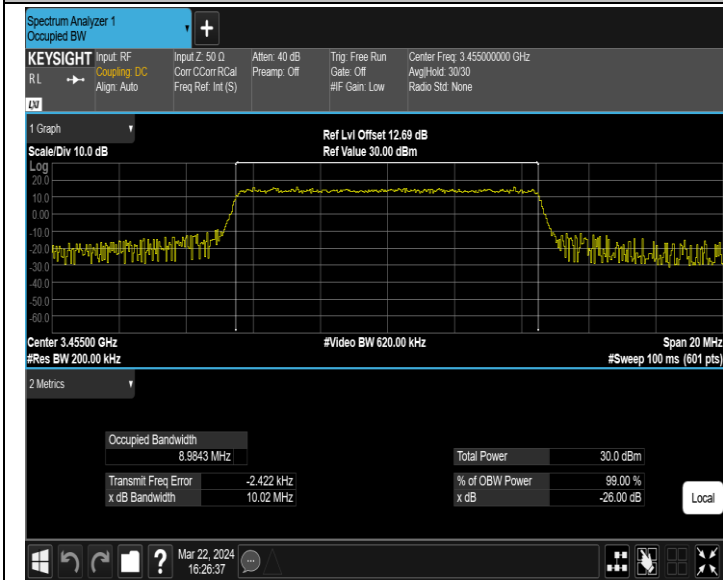
42(3450-3550)-10MHz-16QAM-42140-50RB#0-PASS
