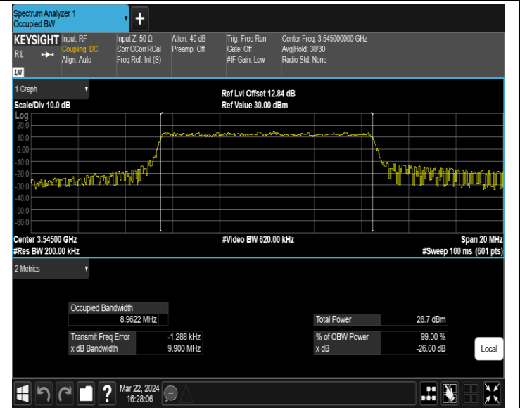
42(3450-3550)-10MHz-64QAM-43040-50RB#0-PASS
