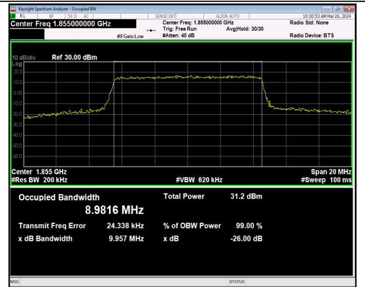
Band2-10MHz-QPSK-18650-50RB#0-PASS
