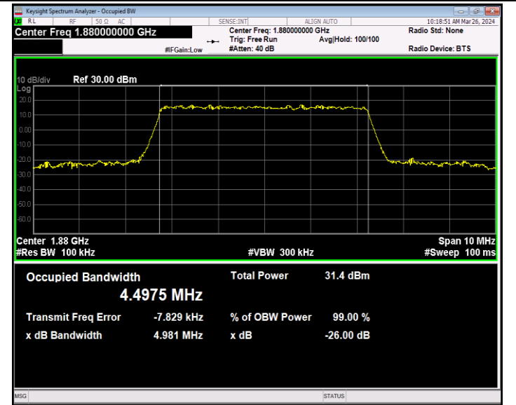
Band2-5MHz-QPSK-18900-25RB#0-PASS
