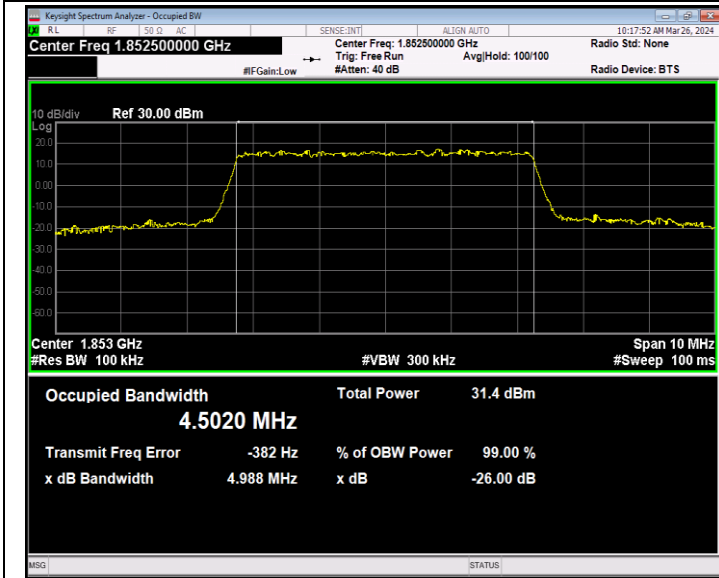
Band2-5MHz-QPSK-18625-25RB#0-PASS
