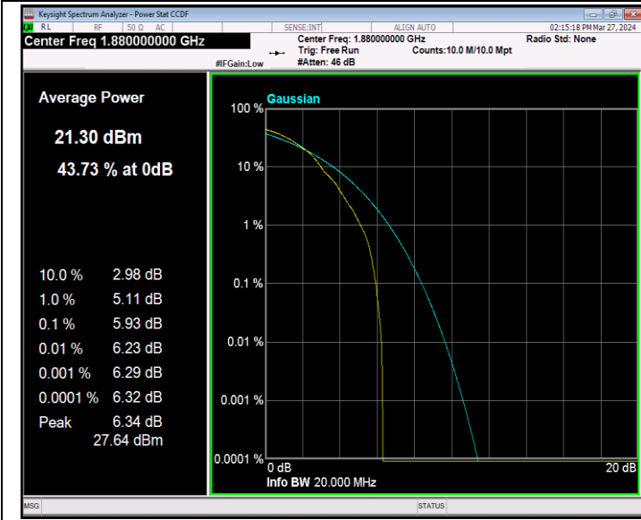
Band2-20MHz-64QAM-18900-1RB#0-PASS
