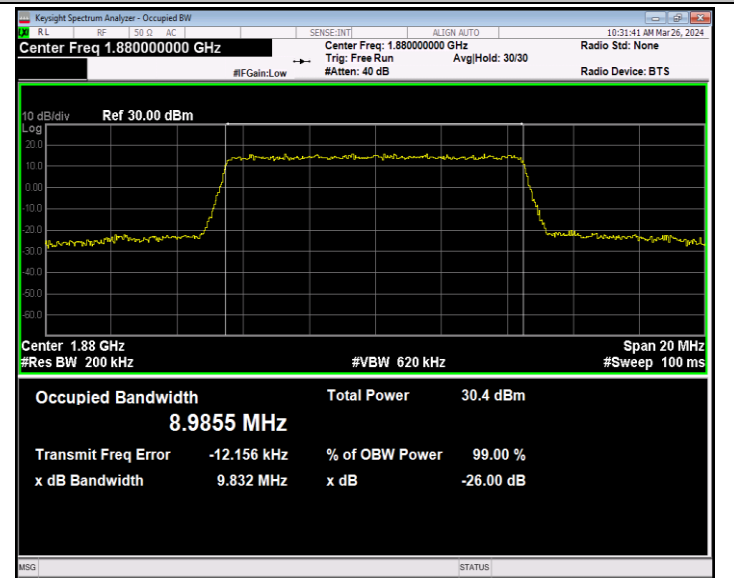
Band2-10MHz-16QAM-18900-50RB#0-PASS
