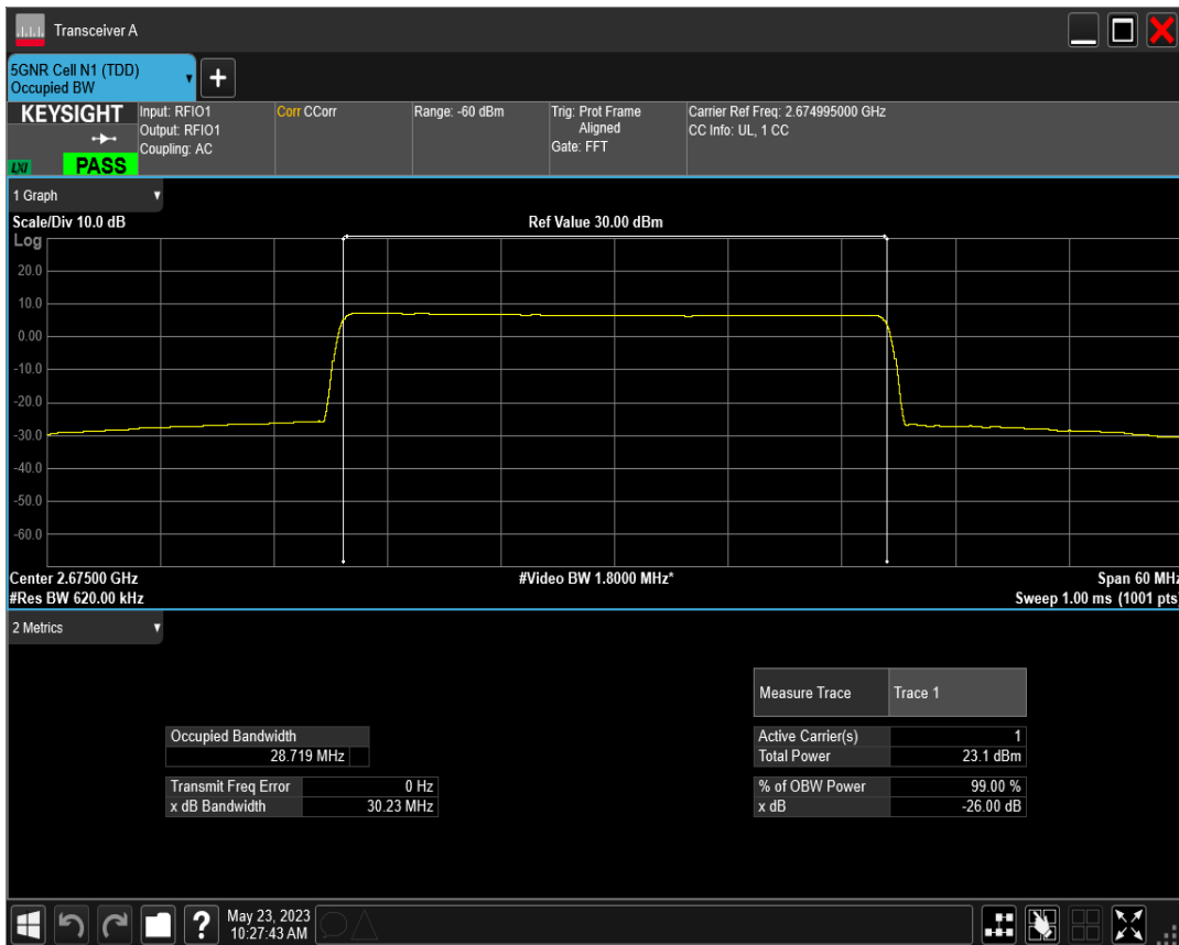
n41 SCS=15kHz CP_QPSK BW=30MHz Channel=534999 RB=160@0
