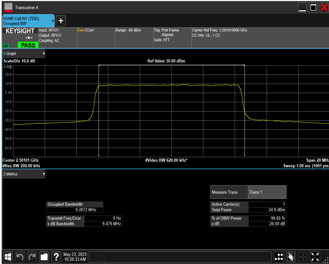
n41 SCS=15kHz DFT_QAM16 BW=10MHz Channel=500202 RB=50@0
