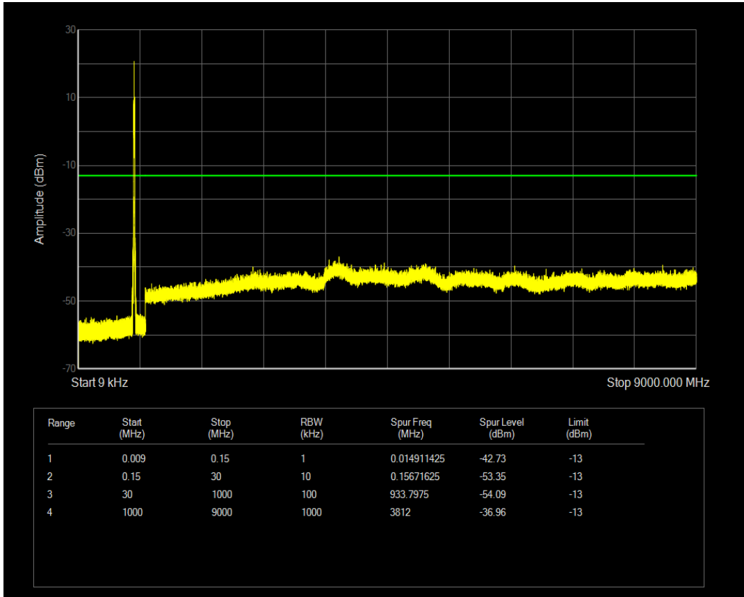
n5 SCS=30kHz DFT_QPSK BW=20MHz Channel=167800 RB=1@0
