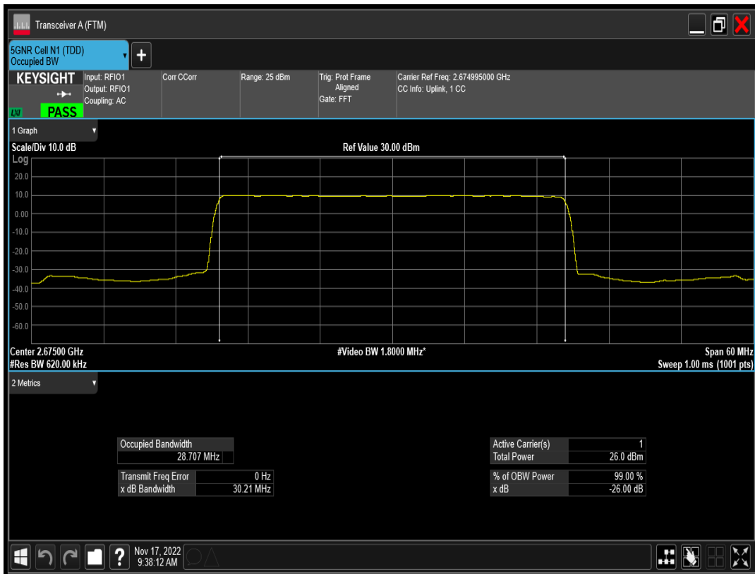
n41 SCS=15kHz DFT_QPSK BW=30MHz Channel=534999 RB=160@0
