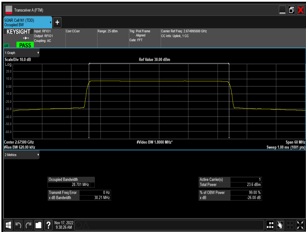
n41 SCS=15kHz CP_QPSK BW=30MHz Channel=534999 RB=160@0
