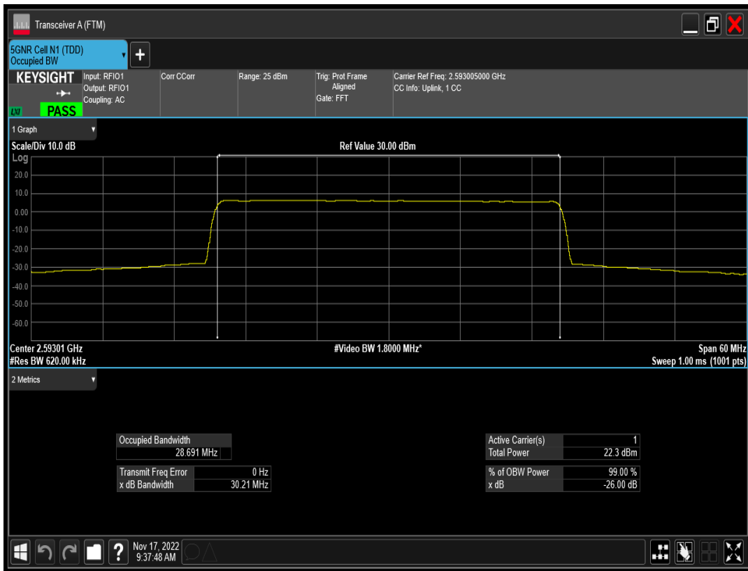
n41 SCS=15kHz CP_QPSK BW=30MHz Channel=518601 RB=160@0
