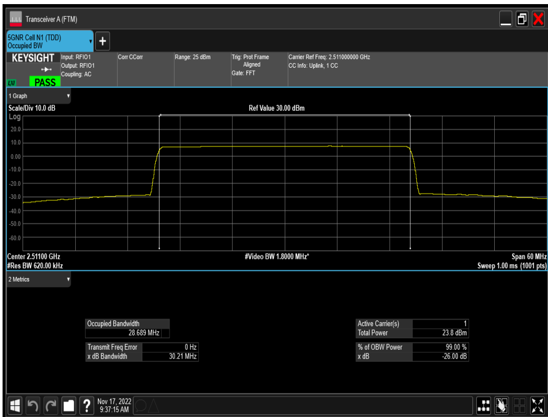
n41 SCS=15kHz CP_QPSK BW=30MHz Channel=502200 RB=160@0
