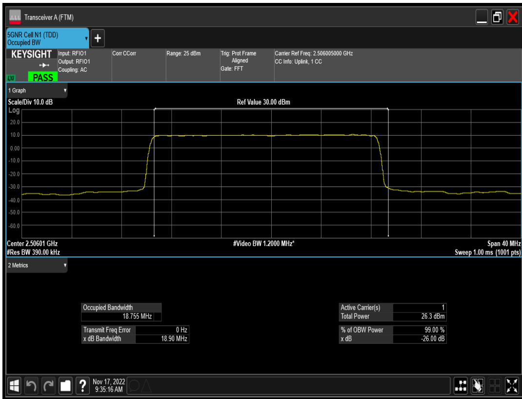
n41 SCS=15kHz DFT_QPSK BW=20MHz Channel=501201 RB=100@0
