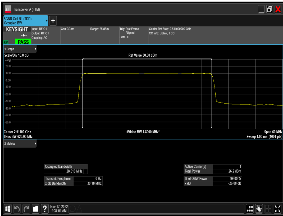
n41 SCS=15kHz DFT_QPSK BW=30MHz Channel=502200 RB=160@0
