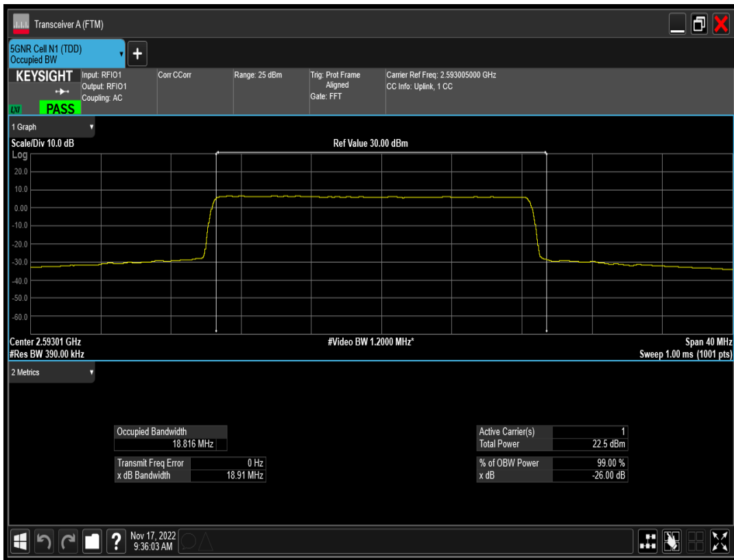
n41 SCS=15kHz CP_QPSK BW=20MHz Channel=518601 RB=106@0
