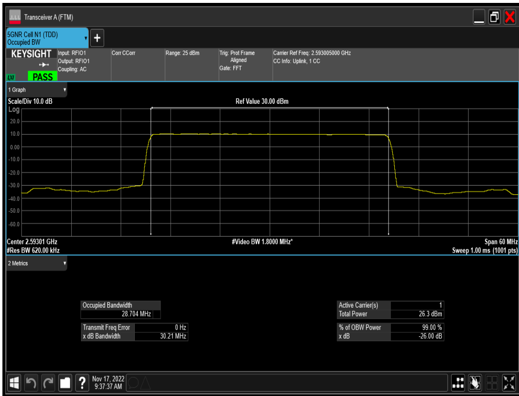
n41 SCS=15kHz DFT_QPSK BW=30MHz Channel=518601 RB=160@0
