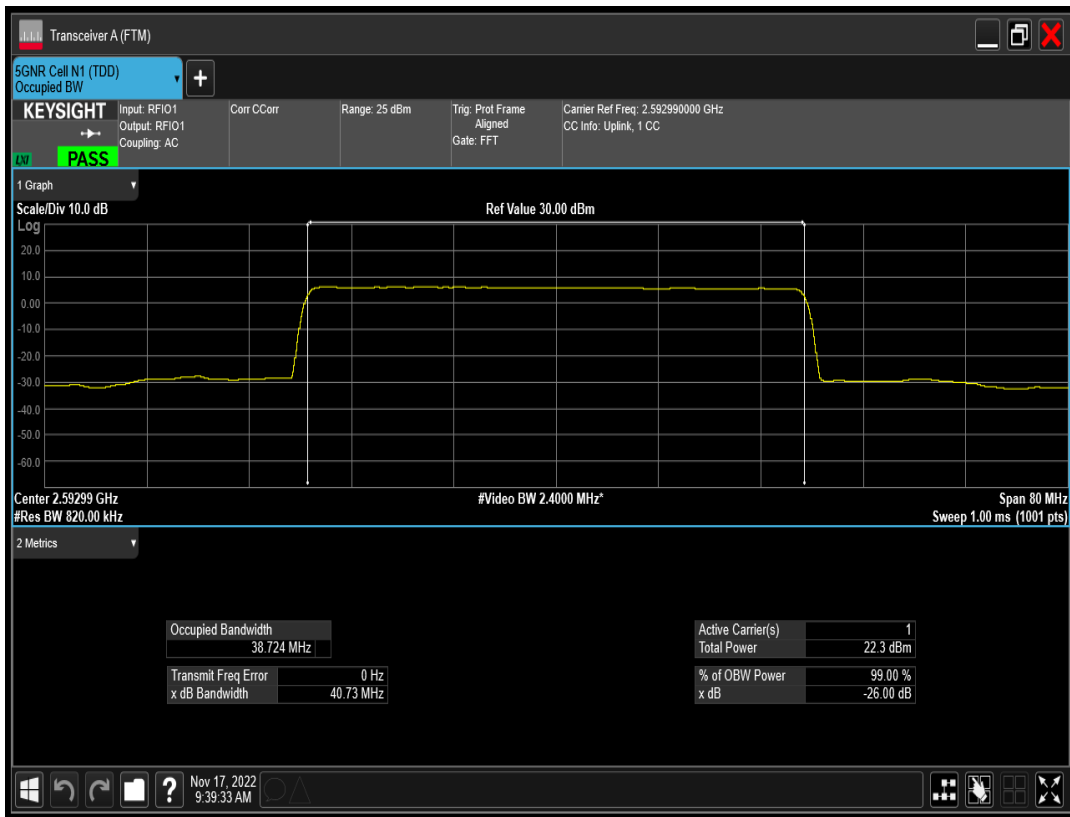
n41 SCS=15kHz CP_QPSK BW=40MHz Channel=518598 RB=216@0
