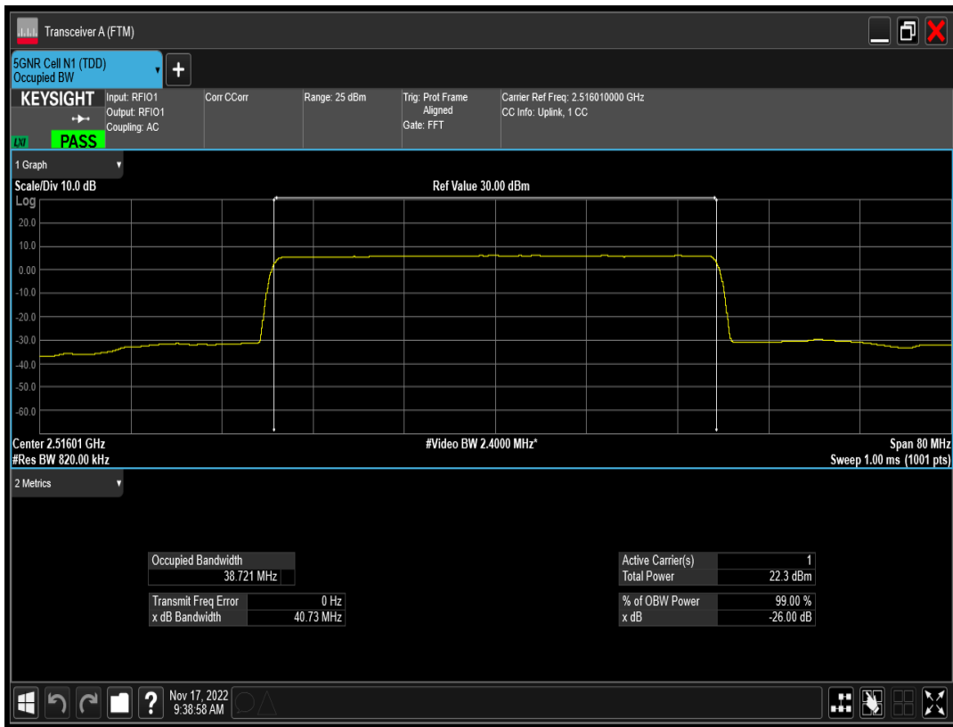
n41 SCS=15kHz CP_QPSK BW=40MHz Channel=503202 RB=216@0
