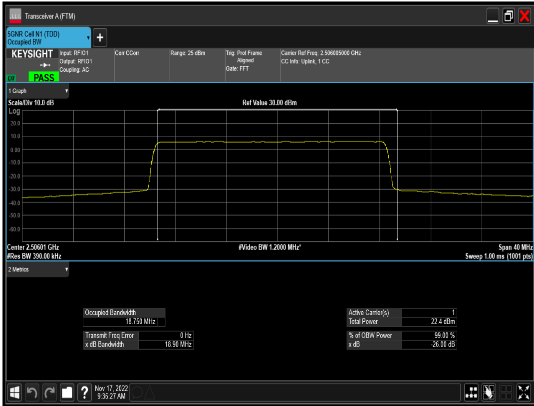
n41 SCS=15kHz CP_QPSK BW=20MHz Channel=501201 RB=106@0
