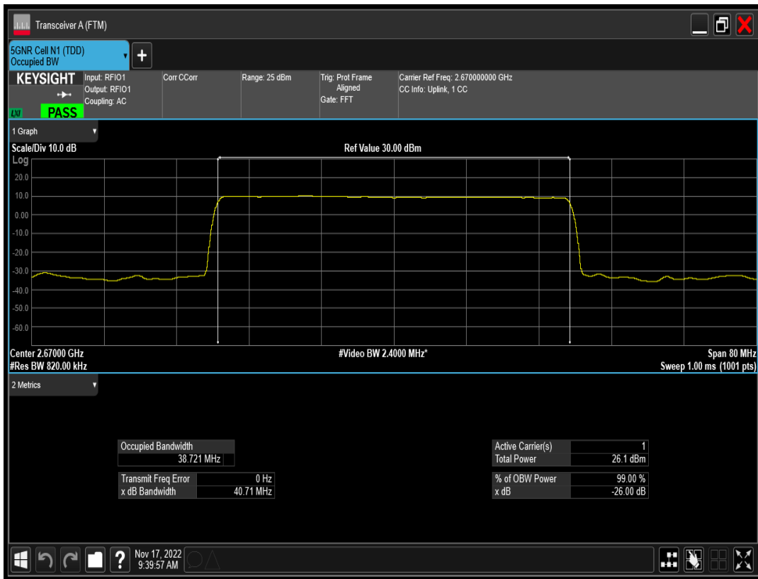
n41 SCS=15kHz DFT_QPSK BW=40MHz Channel=534000 RB=216@0
