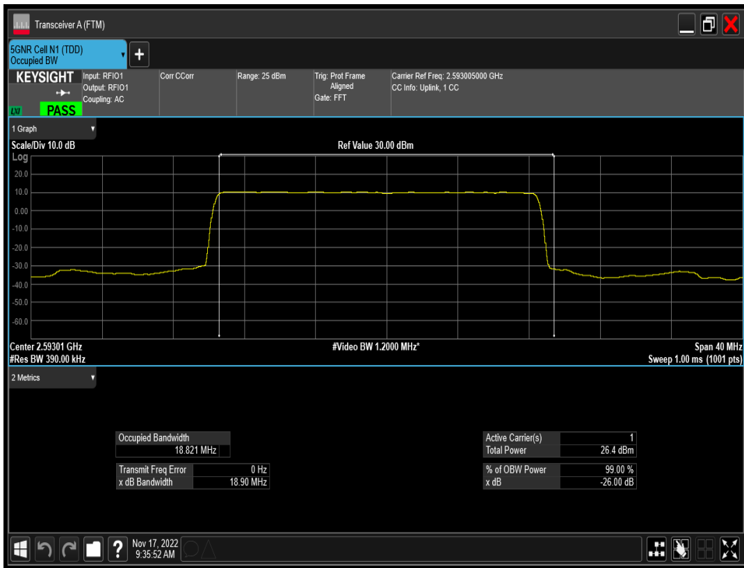
n41 SCS=15kHz DFT_QPSK BW=20MHz Channel=518601 RB=100@0
