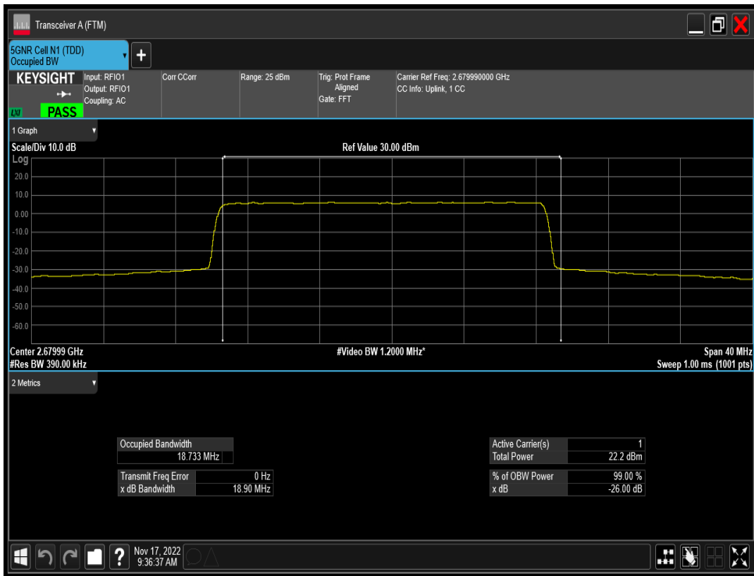
n41 SCS=15kHz CP_QPSK BW=20MHz Channel=535998 RB=106@0
