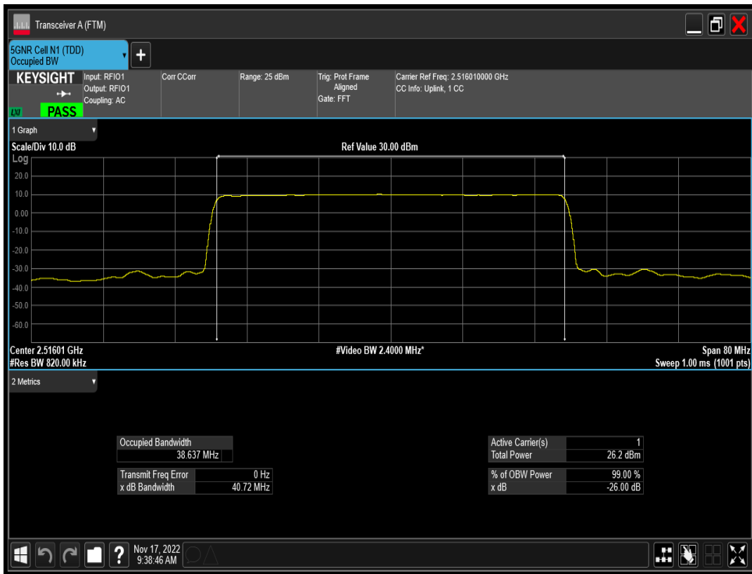
n41 SCS=15kHz DFT_QPSK BW=40MHz Channel=503202 RB=216@0
