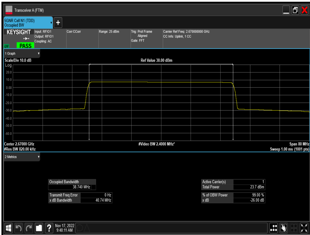
n41 SCS=15kHz CP_QPSK BW=40MHz Channel=534000 RB=216@0
