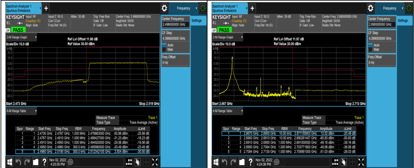
Band41-20MHz-QPSK-41490-1RB#99
