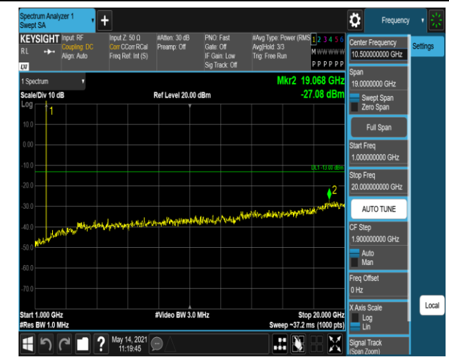
Band4-1.4MHz-QPSK-20175-1RB#0-Range2:1000~20000MHz
