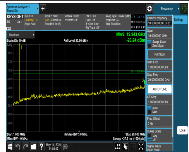
Band2-20MHz-16QAM-19100-1RB#0-Range2:1000~20
