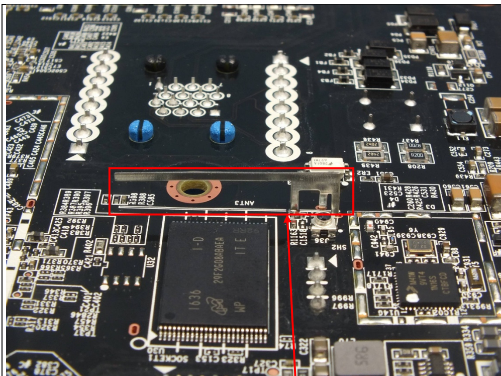
BT/Zigbee Ant.
